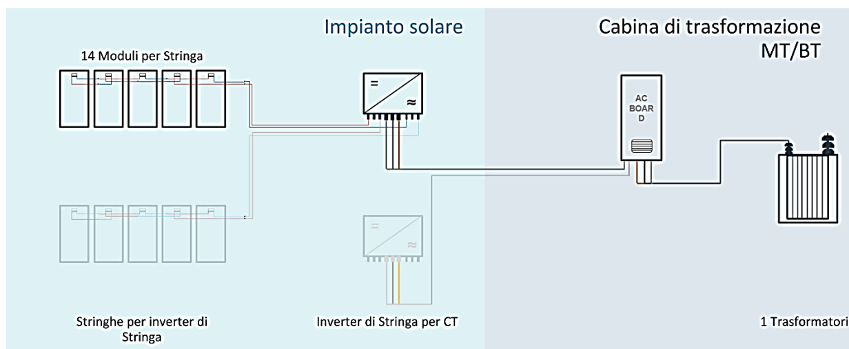
Figura 1-Schema di configurazione elettrica semplificata
