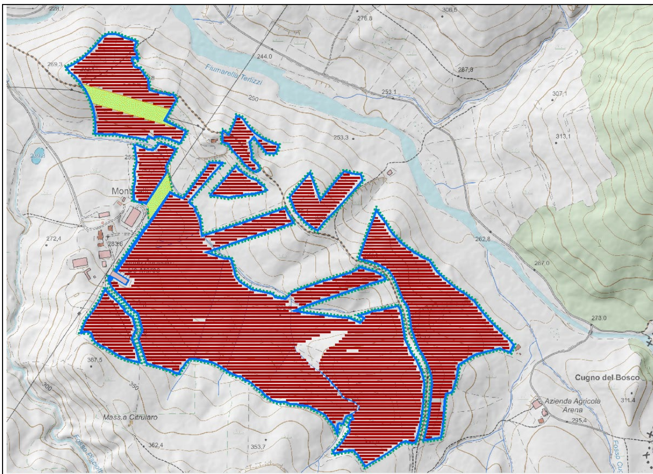
Tav.1: Layout impianto da realizzare
