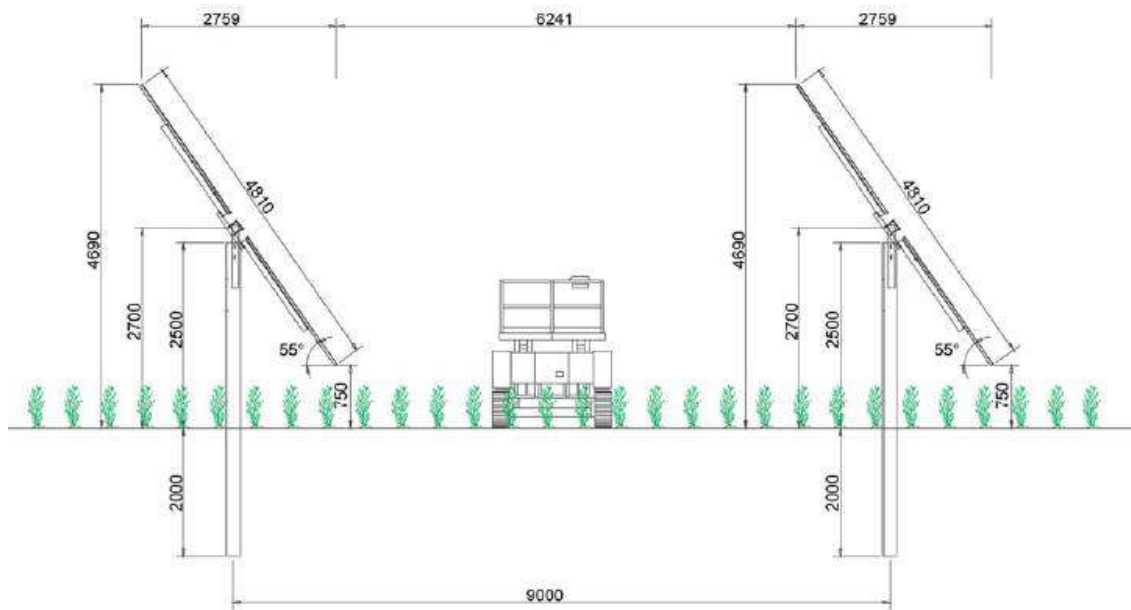
Figure 12.1. – Sezione tipo Aree coltivate
