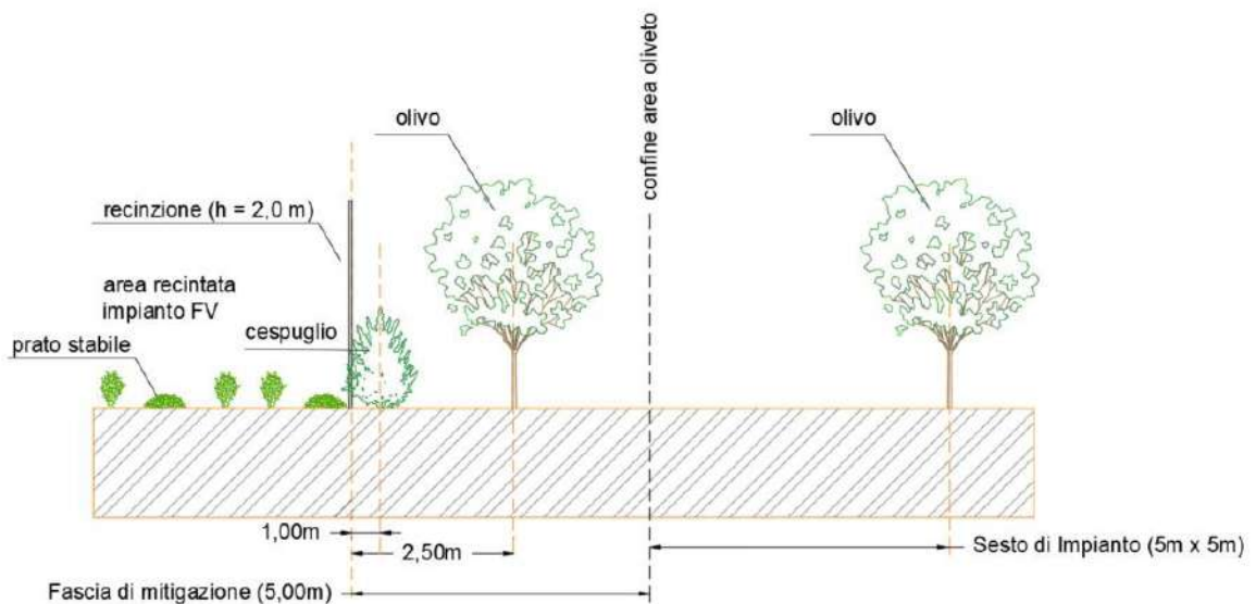
Figure 12.3. – Stralcio di sezione dell'area perimetrale dell'impianto.
