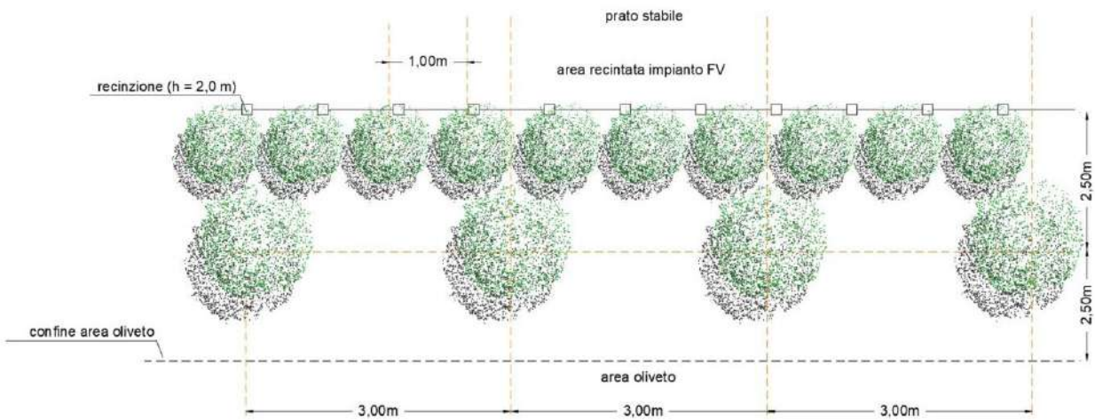
Figure 12.2. – Sezione polispecifica (planimetria di progetto).
