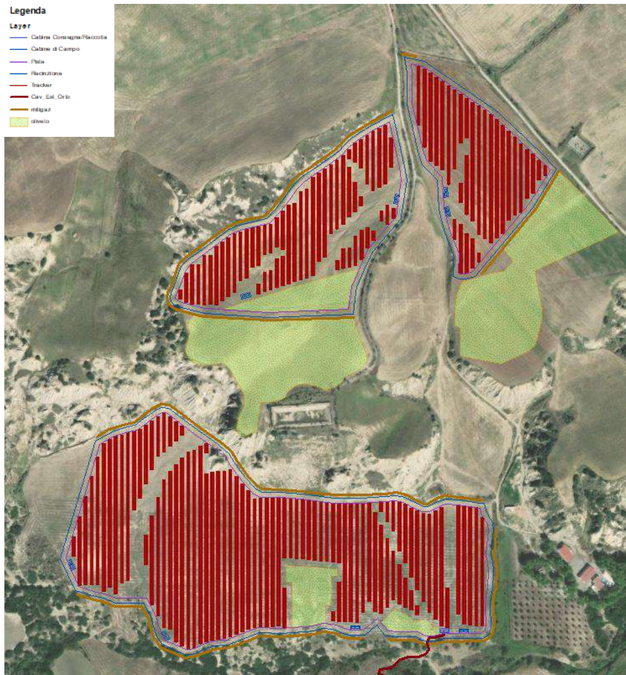
Figura 3.1. – Area di interesse dell'Impianto Agrivoltaico.
