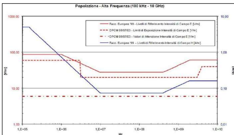
Figura 3.12. – Livelli esposizione Alta Frequenza (100Hz – 10 GHz).
