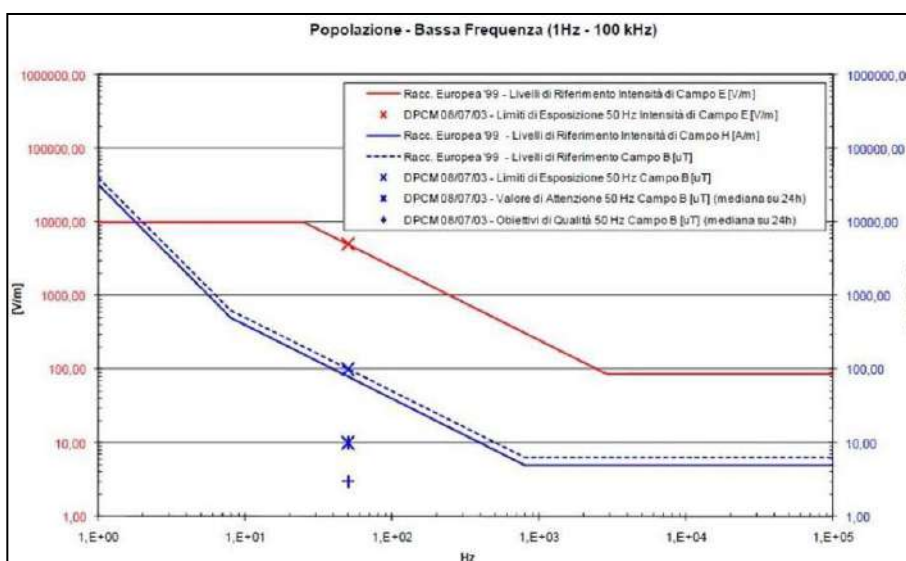
Figura 3.11. – Livelli esposizione Bassa Frequenza (1Hz – 100 kHz).
