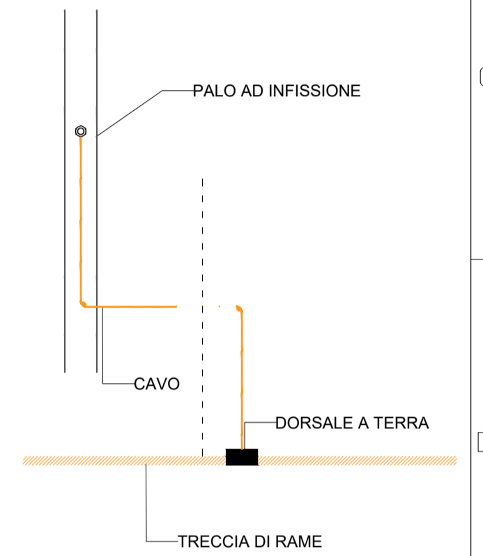
Schema di collegamento struttura a dorsale di terra
