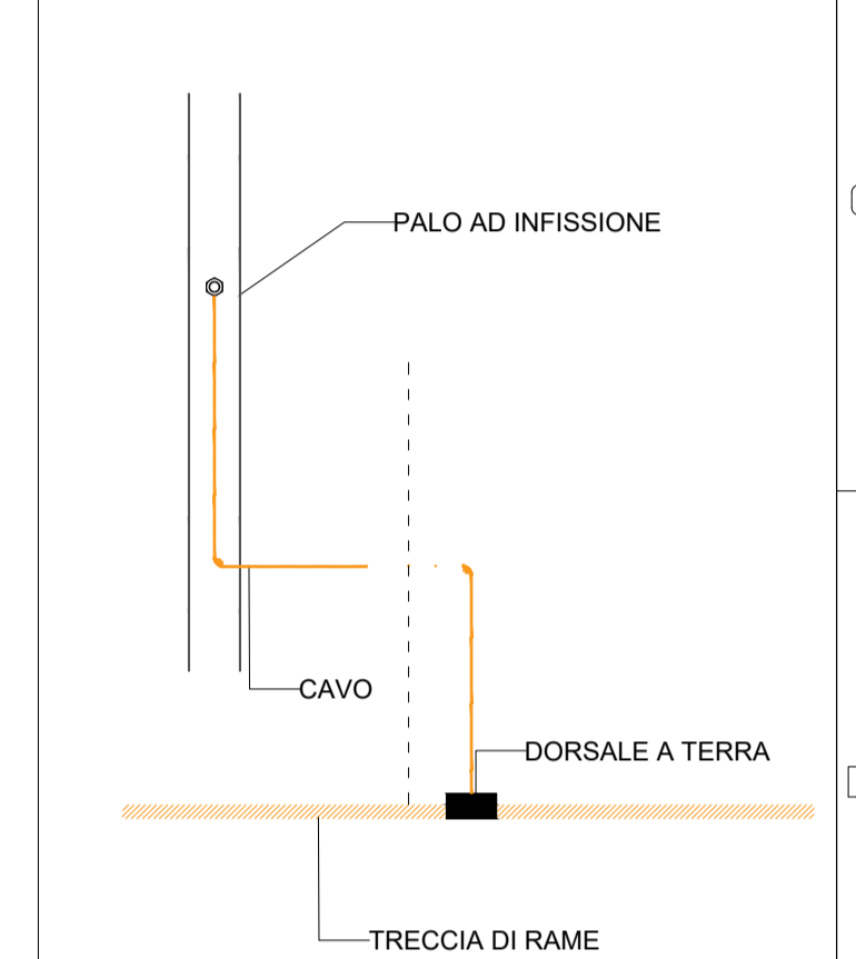
Schema di collegamento struttura a dorsale di terra
