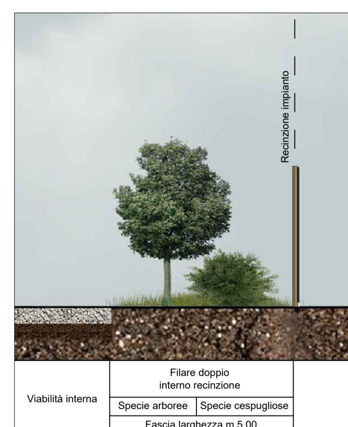
Sezione schematica delle fasce vegetali perimetrali - Tipo C
