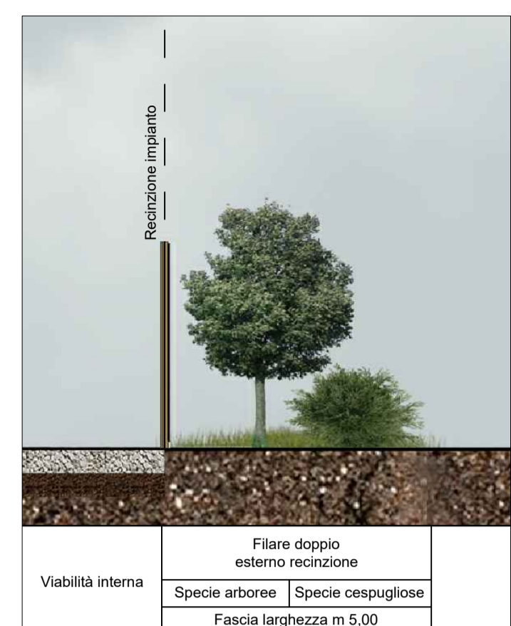
Sezione schematica delle fasce vegetali perimetrali - Tipo B
