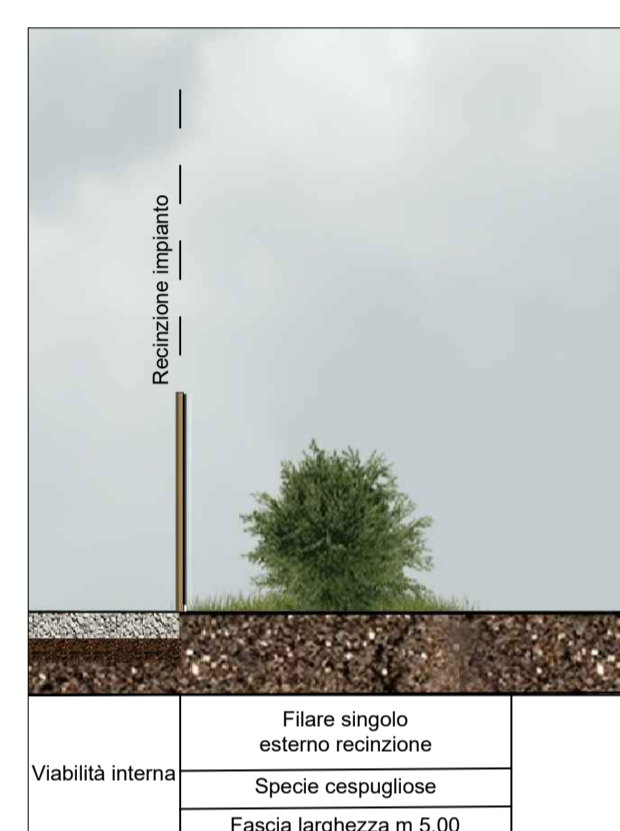
Sezione schematica delle fasce vegetali perimetrali - Tipo D
