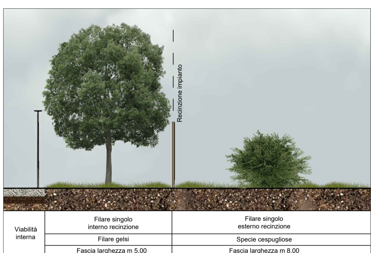
Sezione schematica delle fasce vegetali perimetrali - Tipo E
