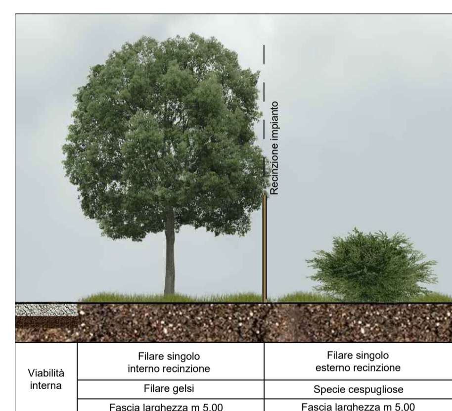
Sezione schematica delle fasce vegetali perimetrali - Tipo F
