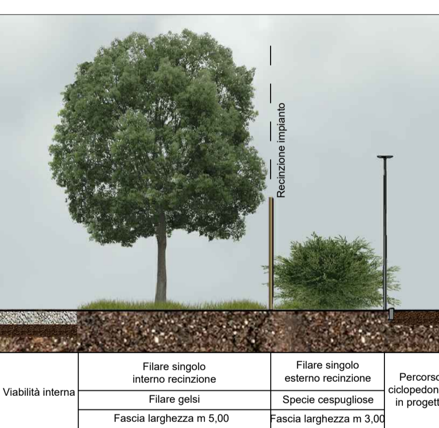
Sezione schematica delle fasce vegetali perimetrali - Tipo H
