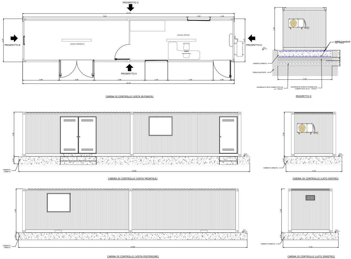
Fig. 21 - Cabina di controllo
