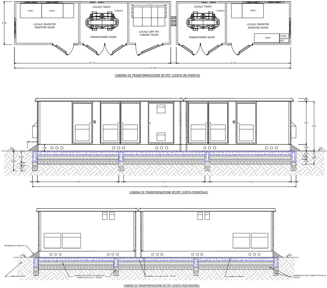
Fig. 19 - Cabina di trasformazione BT/MT
