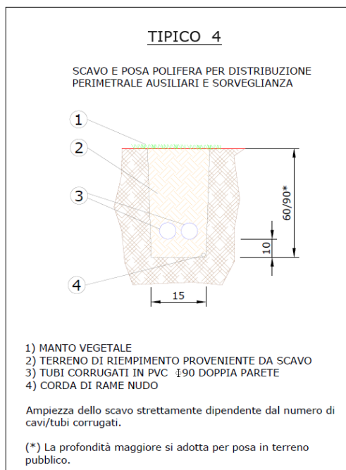
Fig. 18 – Tipici scavi e posa cavi
