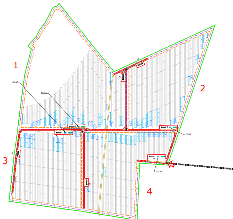
Fig. 7 - Layout di impianto
