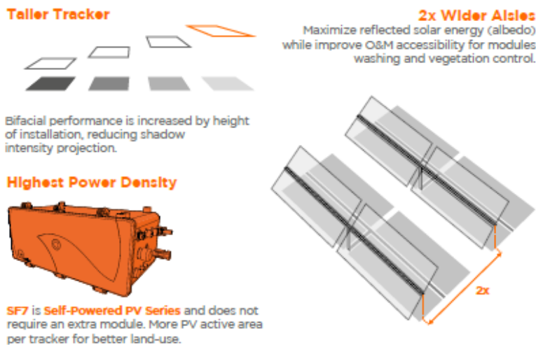
Fig. 9 - Dimensioni, specifiche tecniche e prestazionali Inseguitori solari (Tracker)
