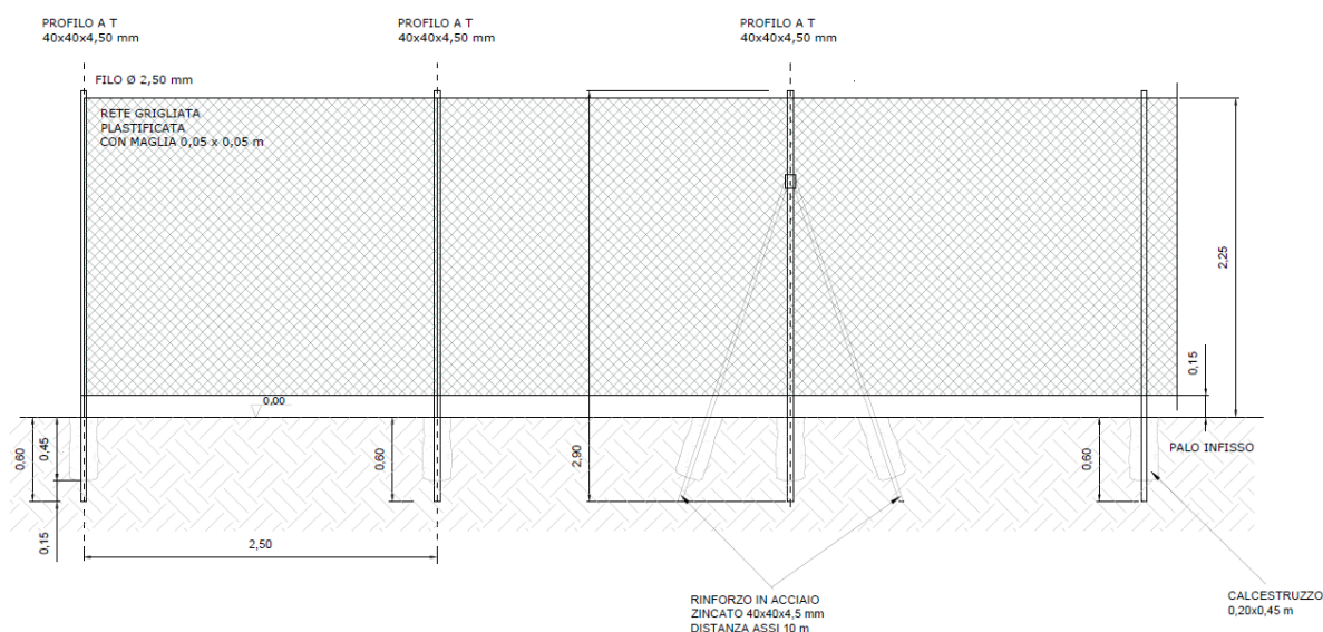
Fig. 15 – Recinzione perimetrale
