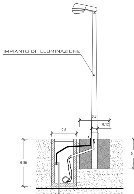
Fig. 25 – Sistema di illuminazione
