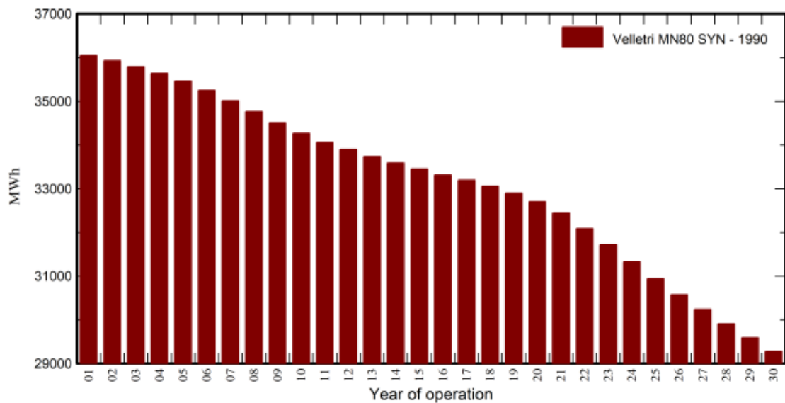
Fig. 30 – Producibilità dell'impianto con degrado moduli (30 anni)
