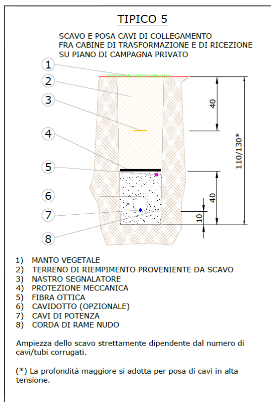
Fig. 18 – Tipici scavi e posa cavi
