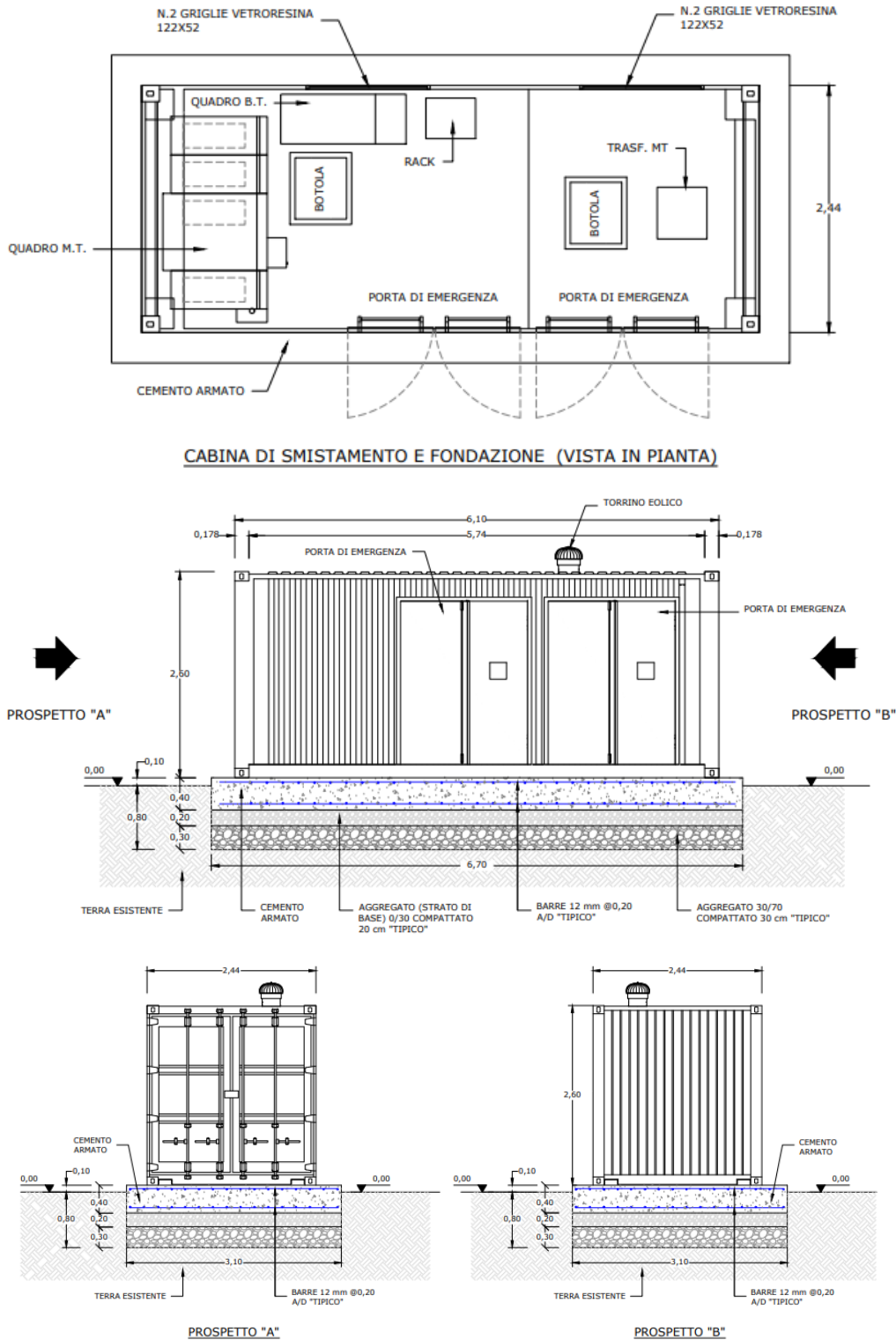
Fig. 20 - Cabina di smistamento
