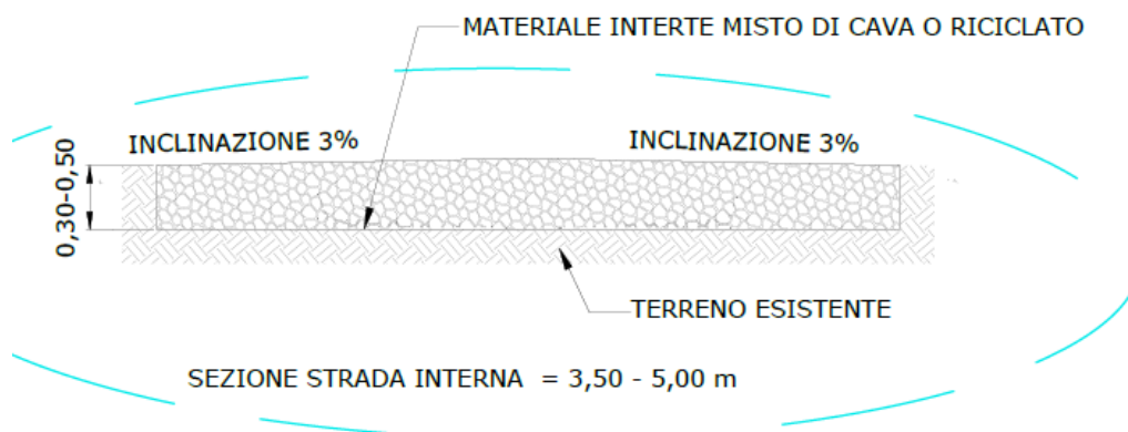
Fig. 17 – Viabilità interna
