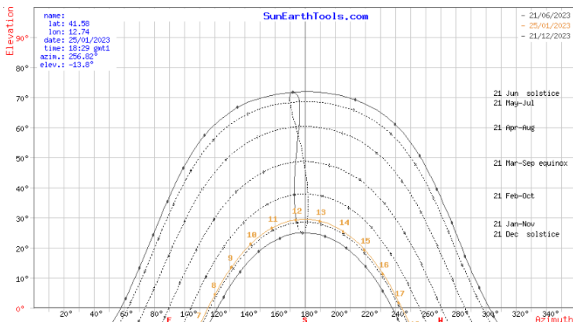
Fig. 28 - Diagramma Solare Polare (riferito al sito di Velletri)
