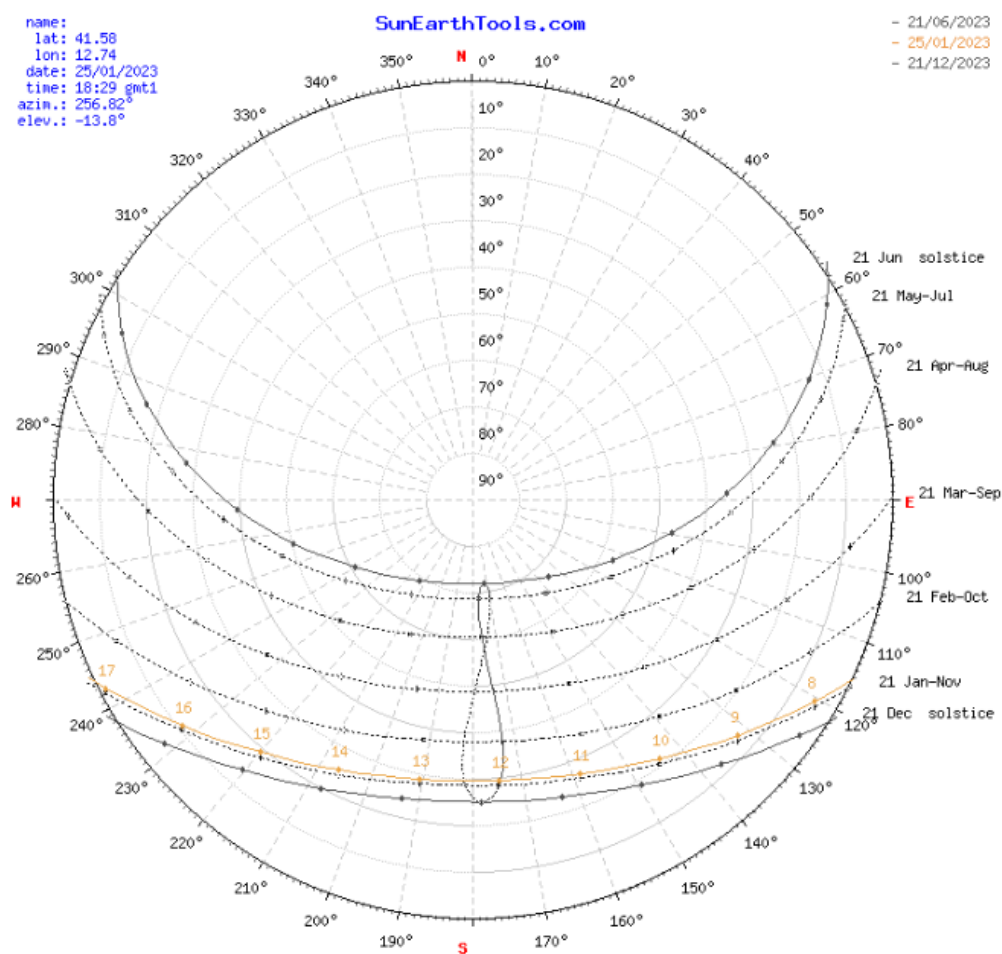
Fig. 27 - Diagramma Solare Polare (riferito al sito di Velletri)
