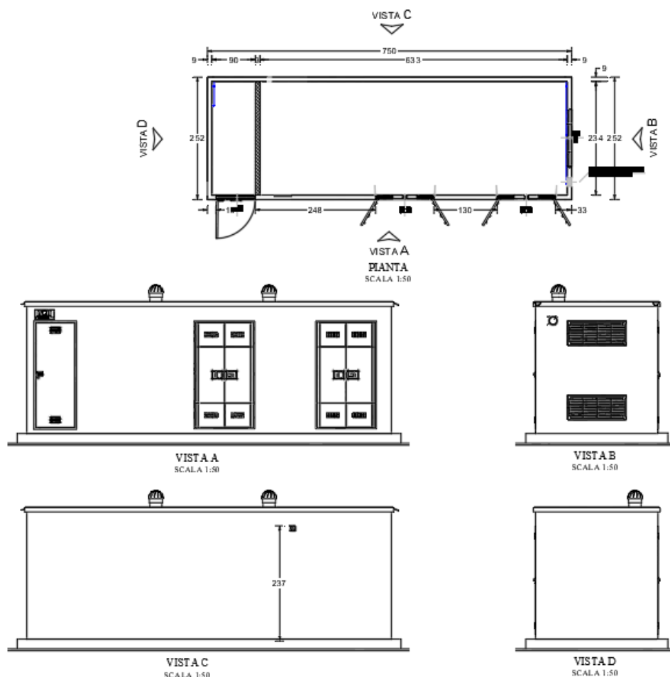
Fig. 23 – Locale tecnico tipo 2
