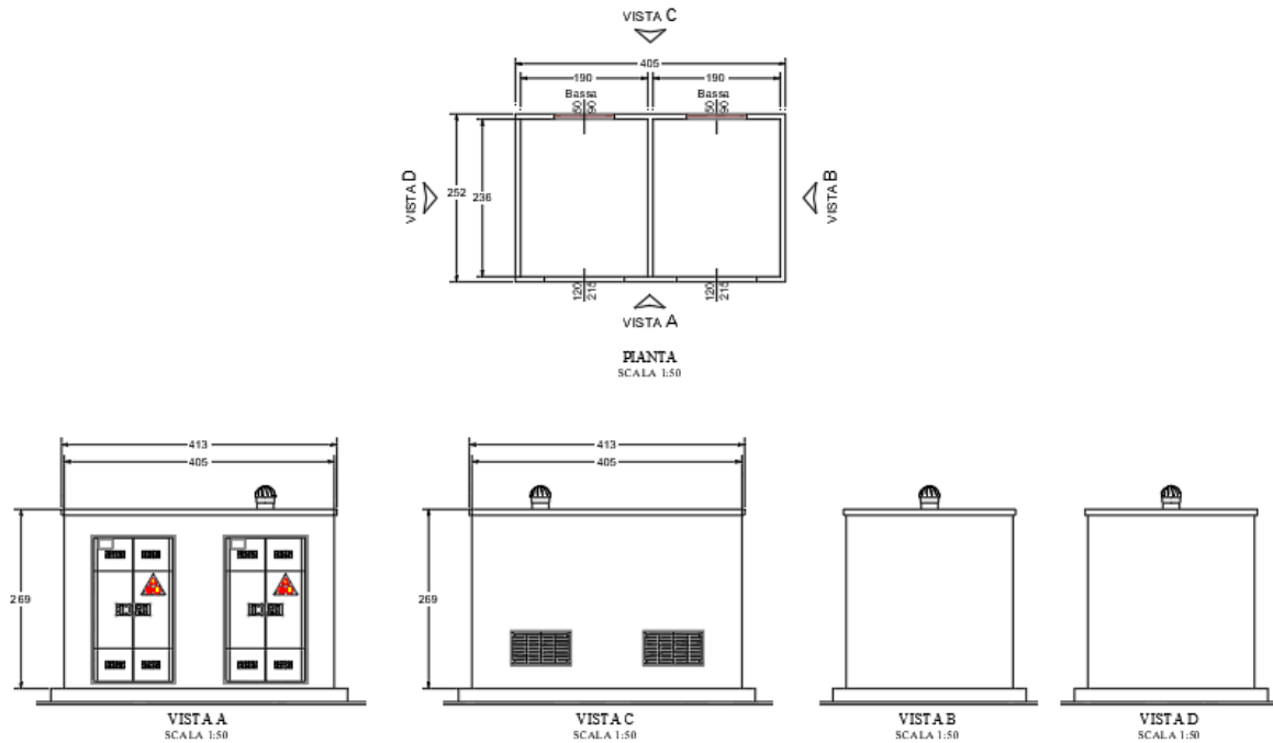
Fig. 22 – Locale tecnico tipo 1
