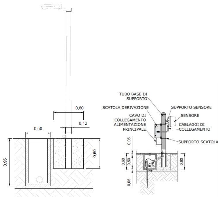
Fig. 24 – Sistema antintrusione
