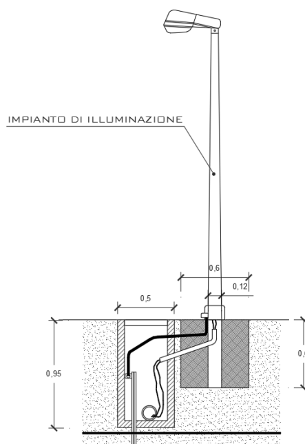
Fig. 2 – Sistema di illuminazione
