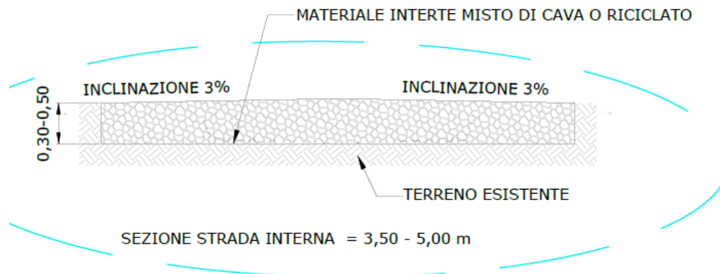
Fig. 21 – Viabilità interna
