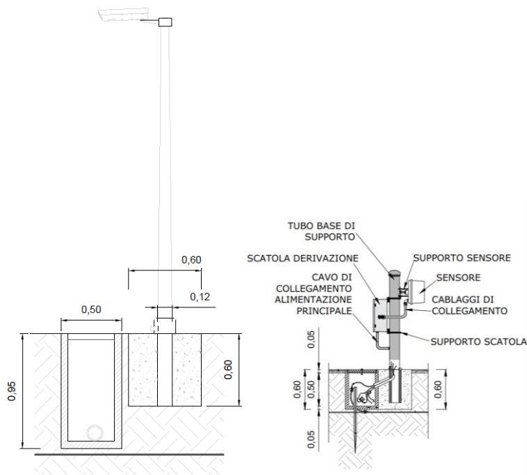
Fig. 22 – Sistema antintrusione
