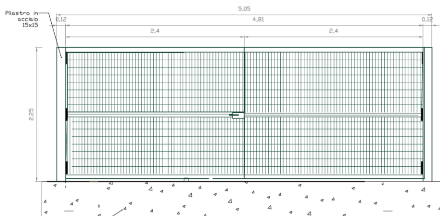
Fig. 20 – Cannello carrabile
