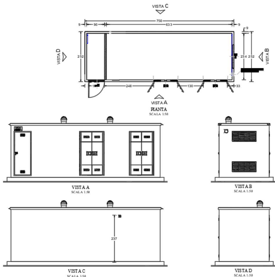
Fig. 18 – Locale tecnico tipo 2
