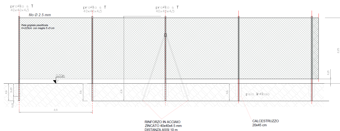
Fig. 19 – Particolare della recinzione
