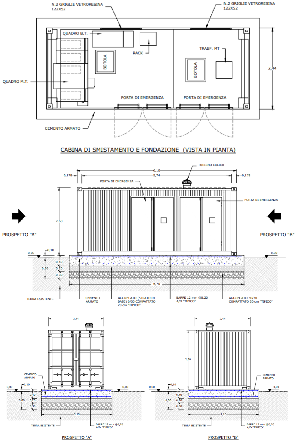
Fig. 15 - Cabina di smistamento
