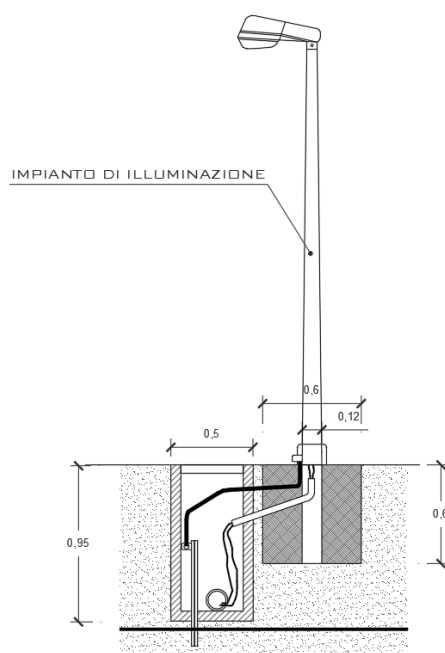
Fig. 23 – Sistema di illuminazione
