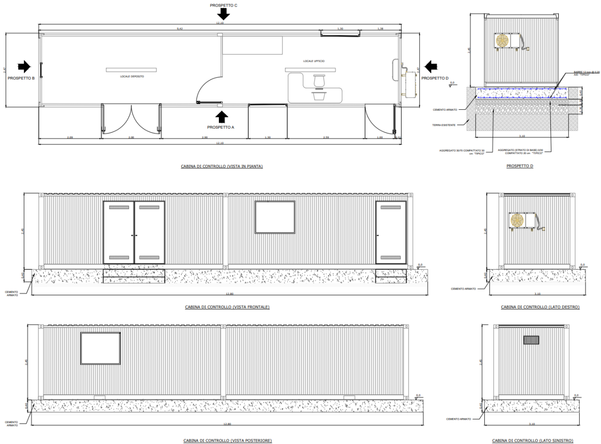
Fig. 16 - Cabina di controllo
