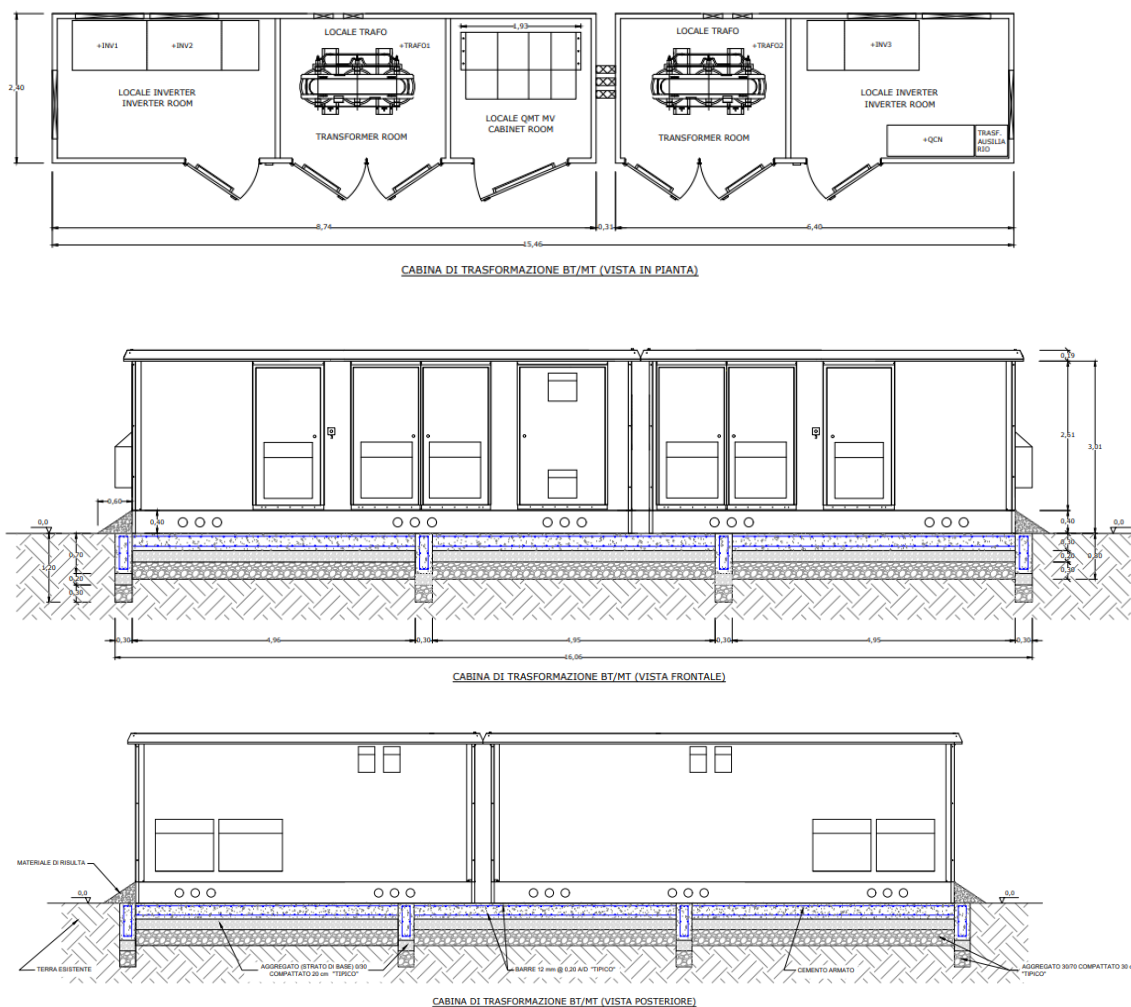
Fig. 14 - Cabina di trasformazione BT/MT
