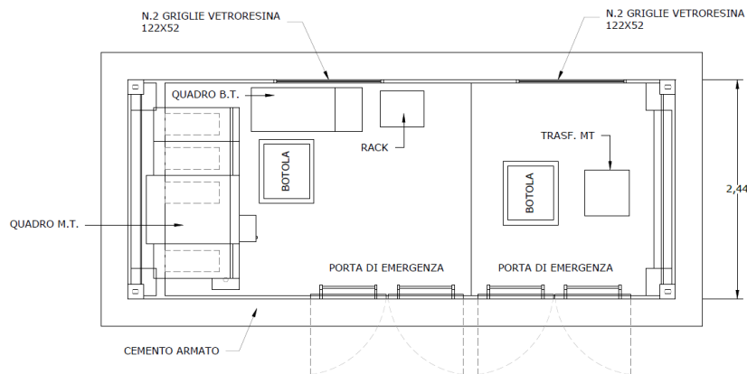
Fig.5 - Ingombri cabine di smistamento
