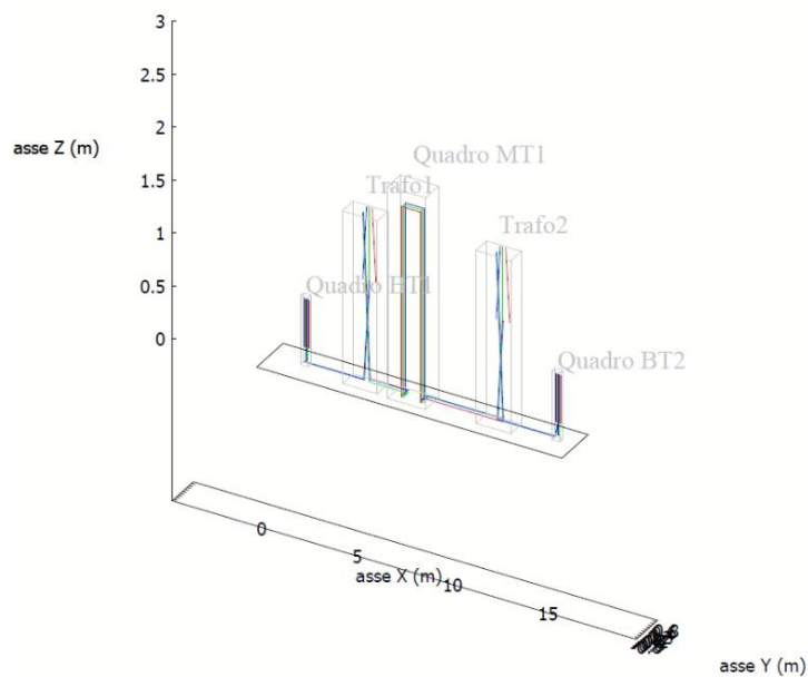
Fig.7 - Modello spaziale cablaggi nelle cabine di trasformazione MT/BT da 3.000 kVA
