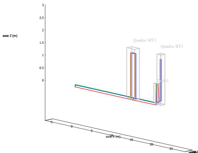
Fig.8 - Modello spaziale cablaggi nella cabina di ricezione
