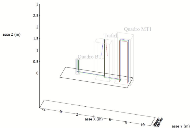
Fig.6 - Modello spaziale cablaggi nelle cabine di trasformazione MT/BT da 2.000 kVA
