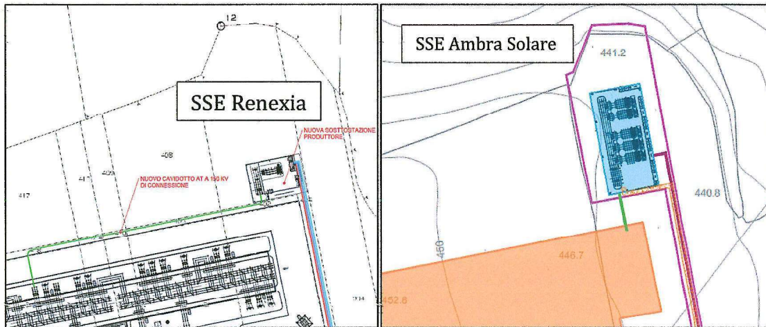
Figura 1: SSE Renexia (sinistra), SSE Ambra Solare (destra)
