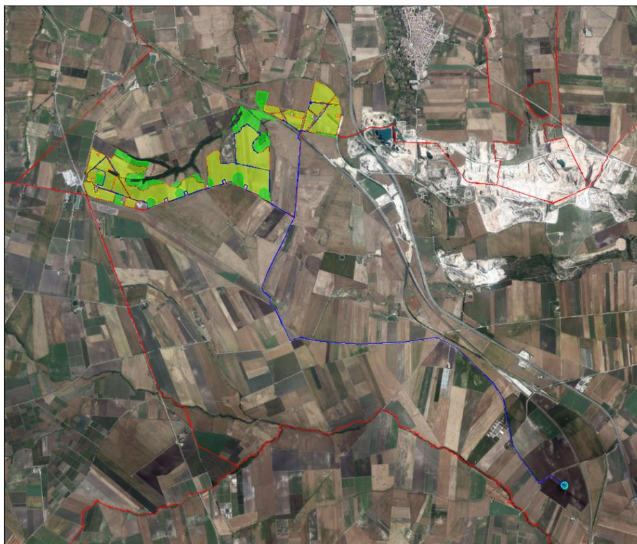
Figura 1: Inquadramento su ortofoto delle aree occupate dal futuro impianto fotovoltaico
