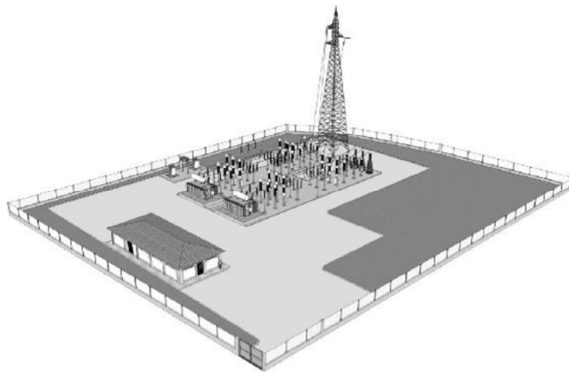
Fig. 3a: Rappresentazione di una tipica Stazione di Utente 150/20 kV con apparecchiature isolate in aria
