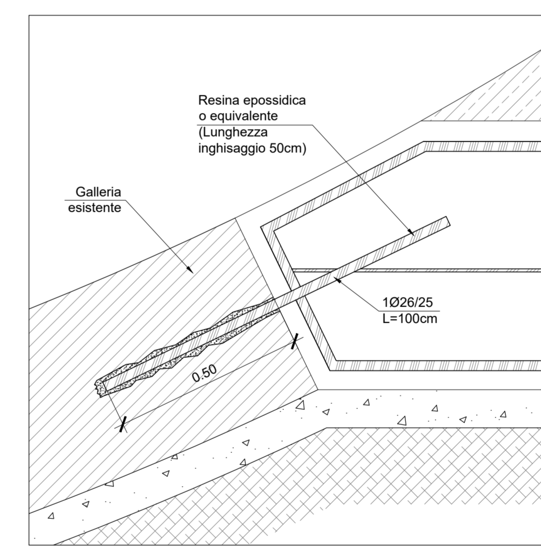
SEZIONE C-C SCALA 1:50
