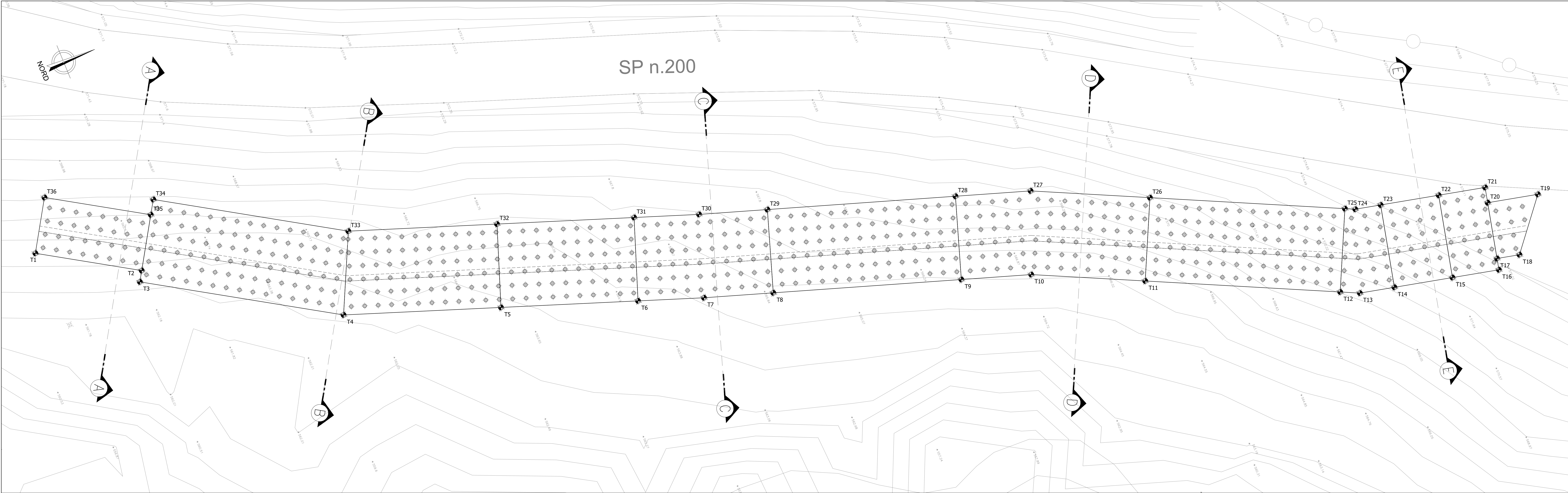
PIANTA TRACCIAMENTO MURO DI SOTTOSCARPA ASSE 3 1:100
