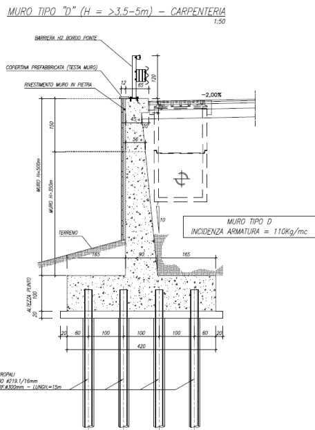
Figura 4.5 - Muri Asse 5: muro tipo D.
