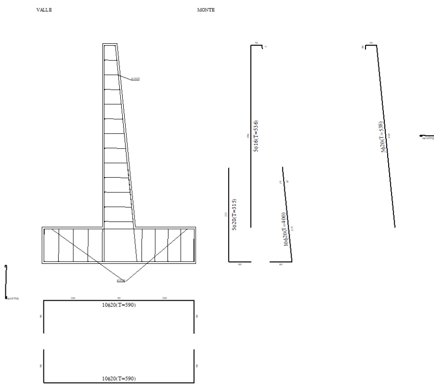
Figura 5.25 – Muri di sottoscarpa, muro Tipo D: distinta ferri.
