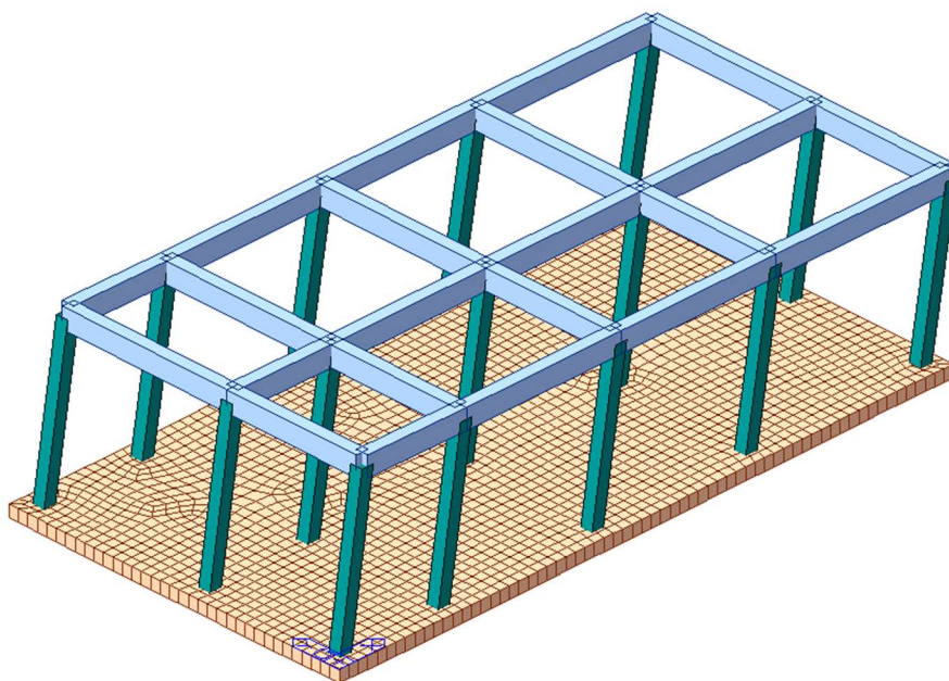
Modo 2 – Traslazionale lungo Y
