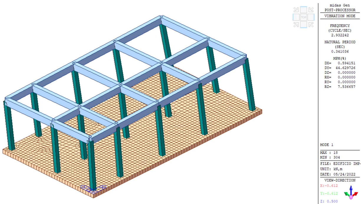
Modo 1 – Traslazionale lungo X
