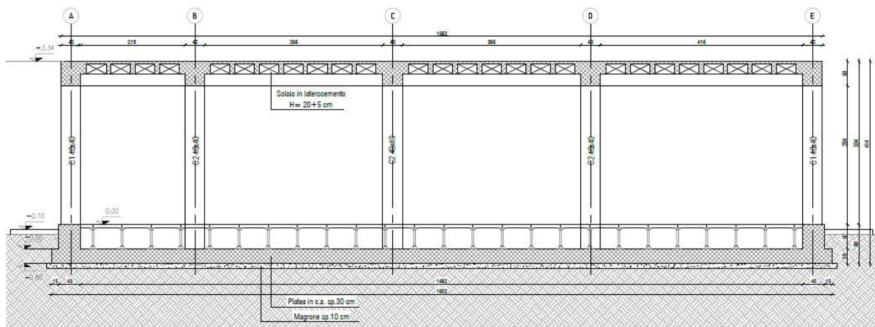
Figura 3: Sezione AA
