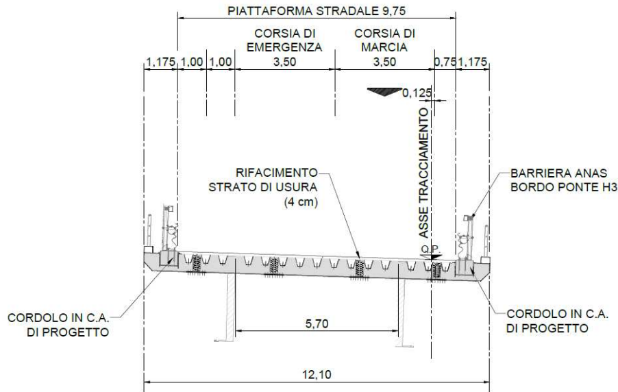
Nuovo cordolo in progetto con barriera di sicurezza
