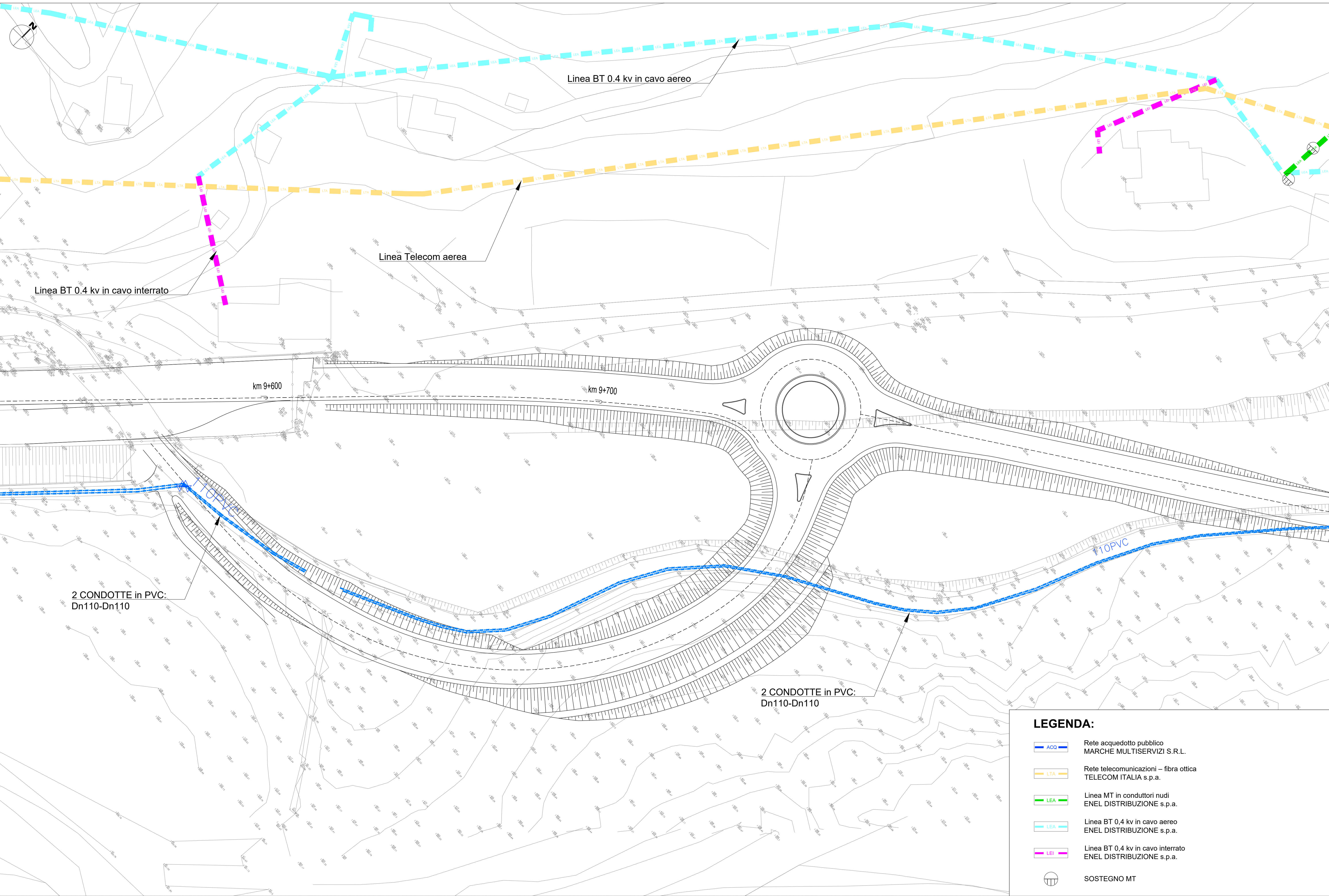
PLANIMETRIA DI CENSIMENTO DELLE INTERFERENZE - COMUNE DI SAN GIUSTINO - scala 1:500
