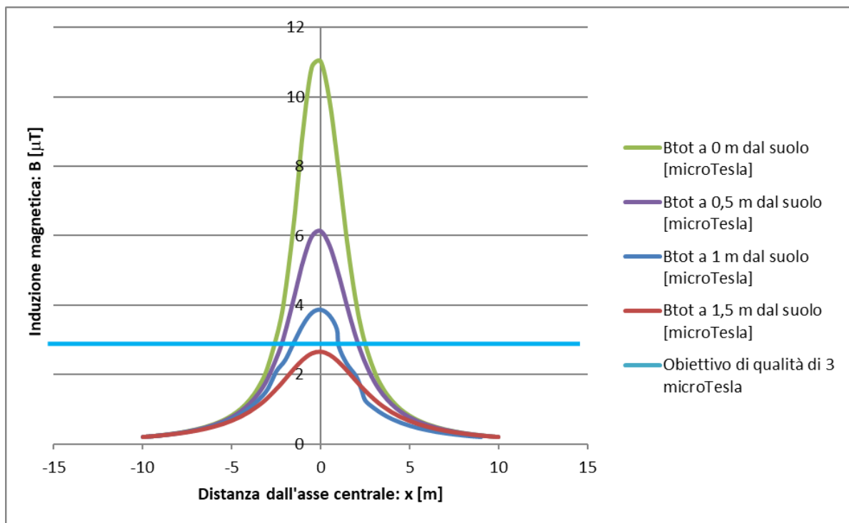
Figura 3: Andamento del campo magnetico generato dal cavidotto, composto da sei terne: 630 mm 2
