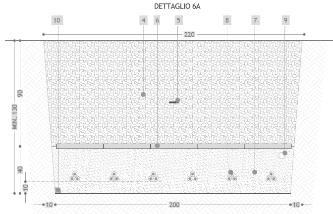
Figura 2: Sezione tipo cavidotto composta da sei terne da 630 mm 2
