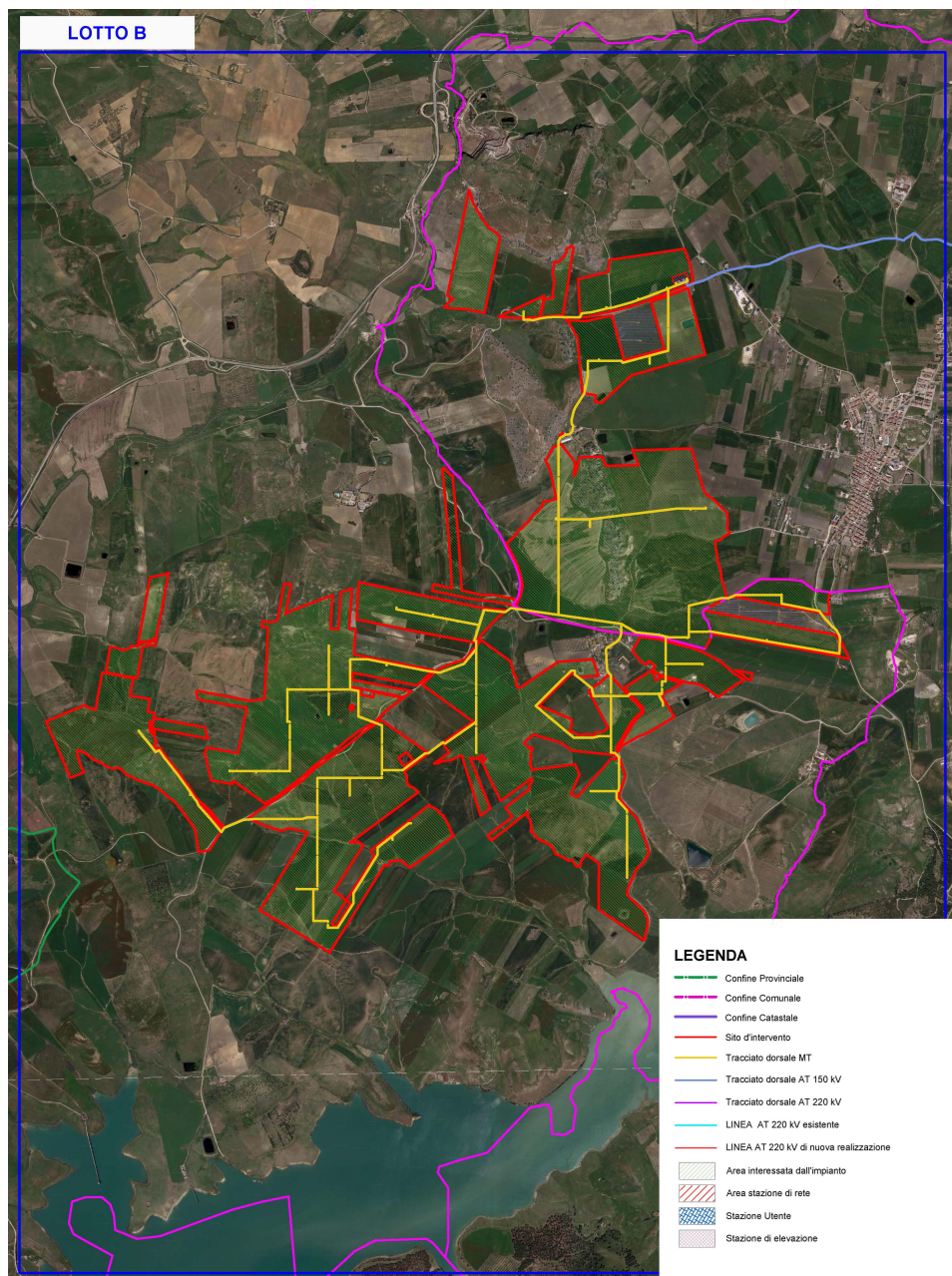
Figura 3 C - Ortofoto dell'area di impianto agro-fotovoltaico denominato "Lotto B" ricadente nei comuni di Monreale (PA) e di Roccamena (PA) in località contrade contrade Capparini, Gamberi, Ponte e Sticca
