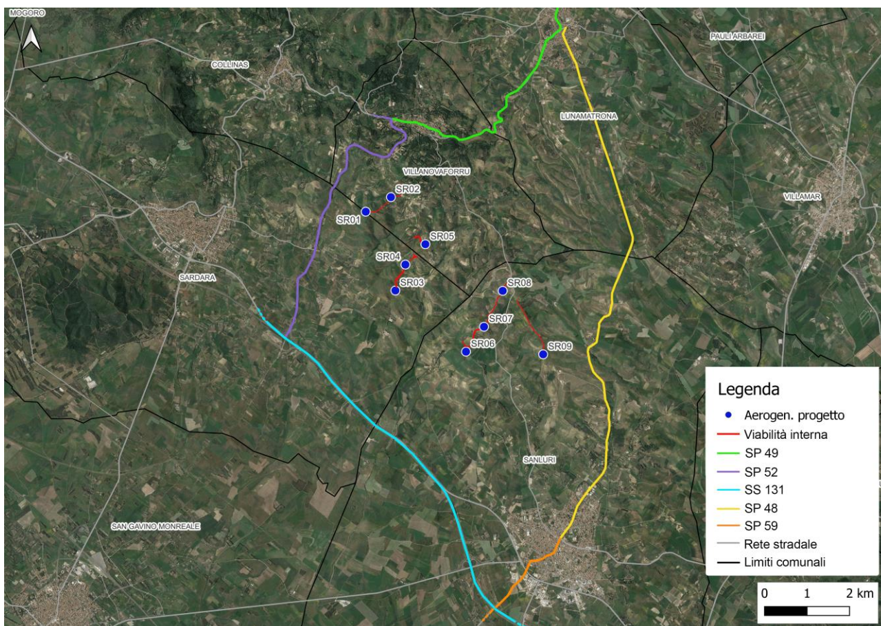
Figura 3.2 - Sistema della viabilità di accesso all'impianto
