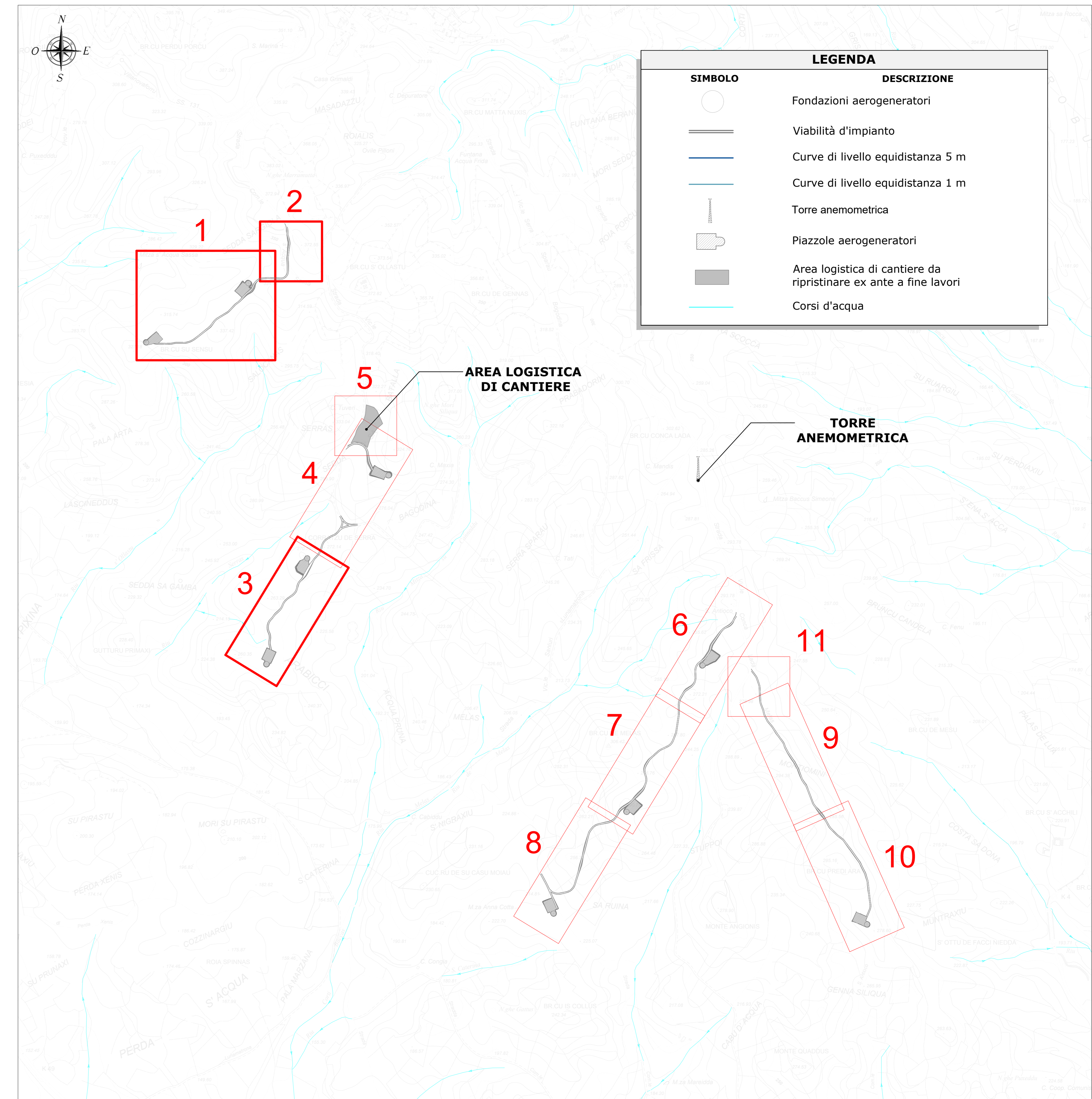
PLANIMETRIA QUADRO 2 - SCALA 1:1.000
