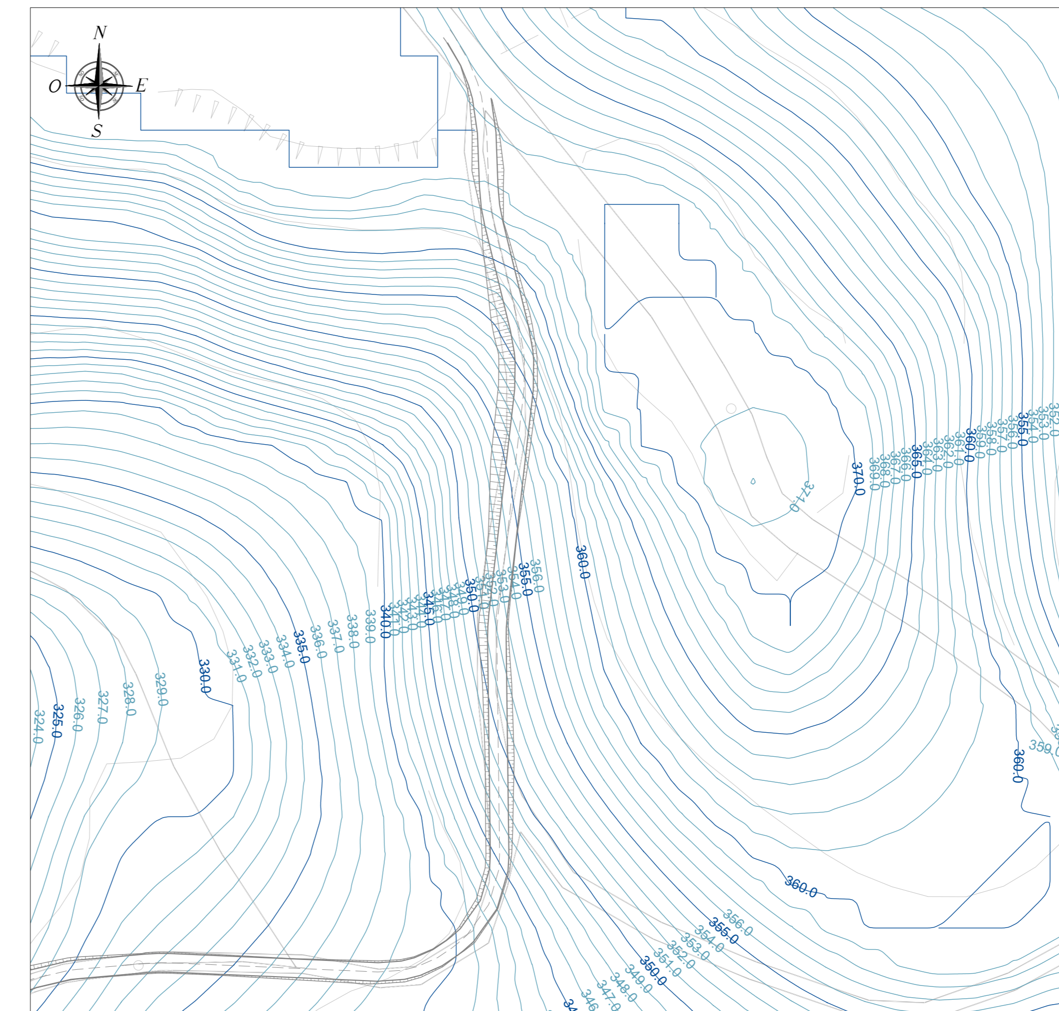
PLANIMETRIA QUADRO 2 - SCALA 1:1.000
