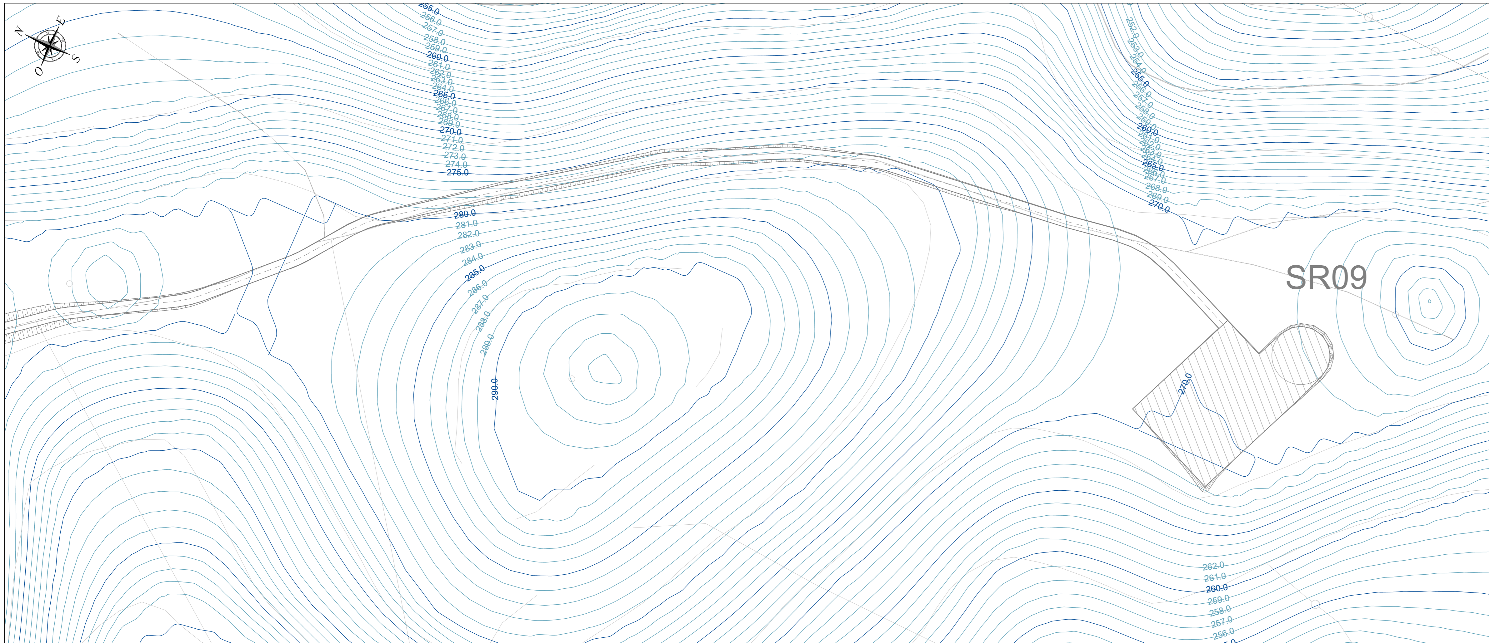
PLANIMETRIA QUADRO 10 - SCALA 1:1.000
