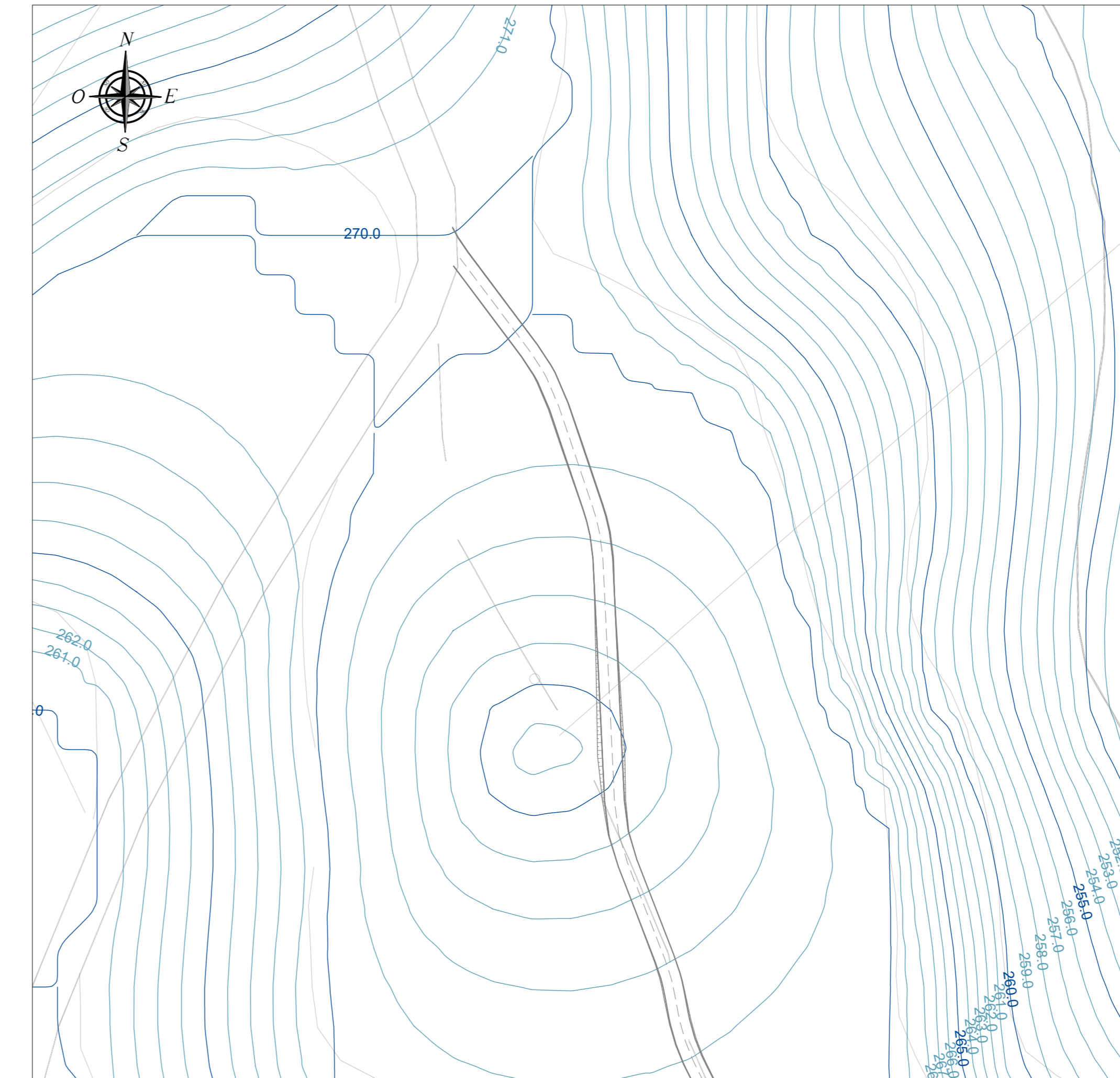
PLANIMETRIA QUADRO 11 - SCALA 1:1.000
