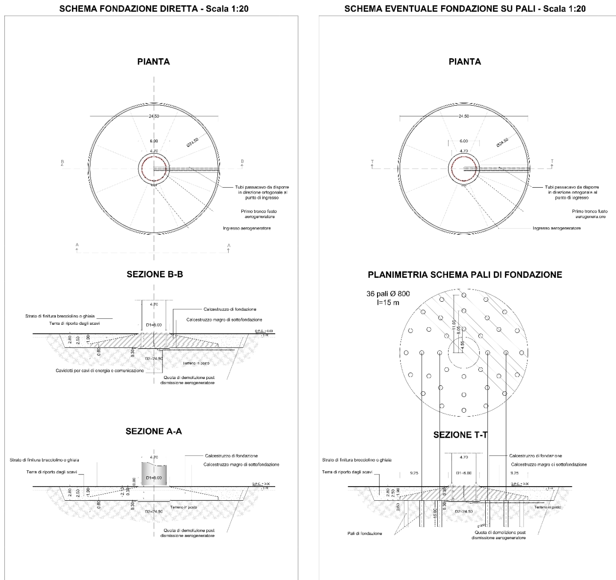
Figura 5.37 – Soluzioni costruttive delle strutture di fondazione degli aerogeneratori
