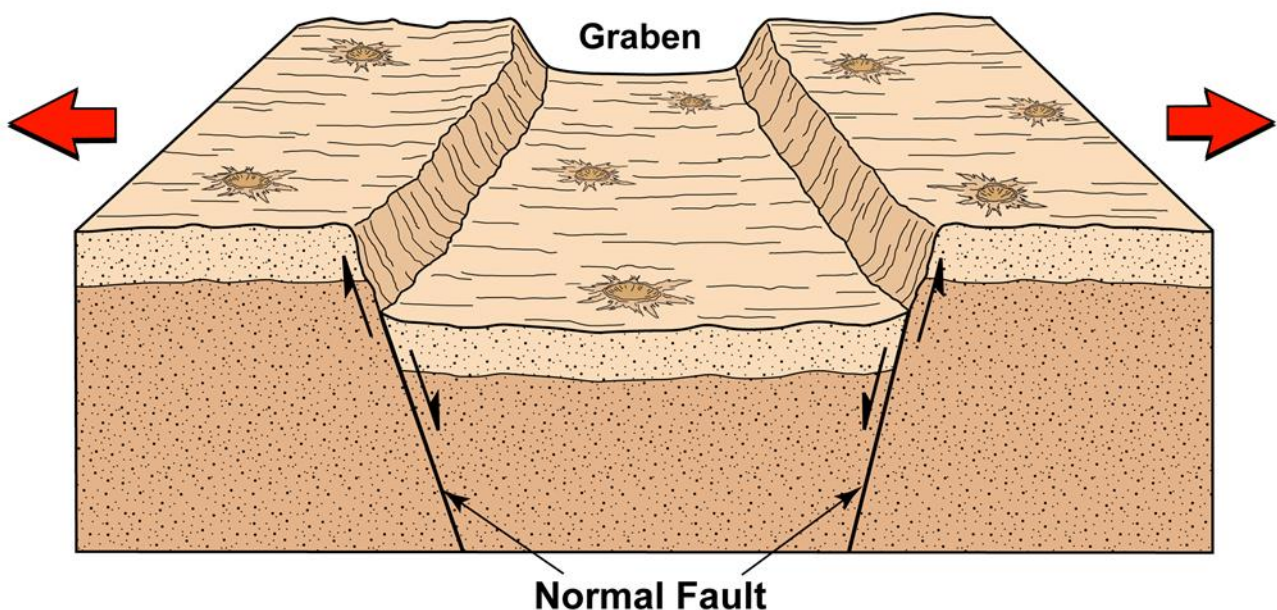
Figura 8.2 - Schematizzazione della struttura di una fossa tettonica
