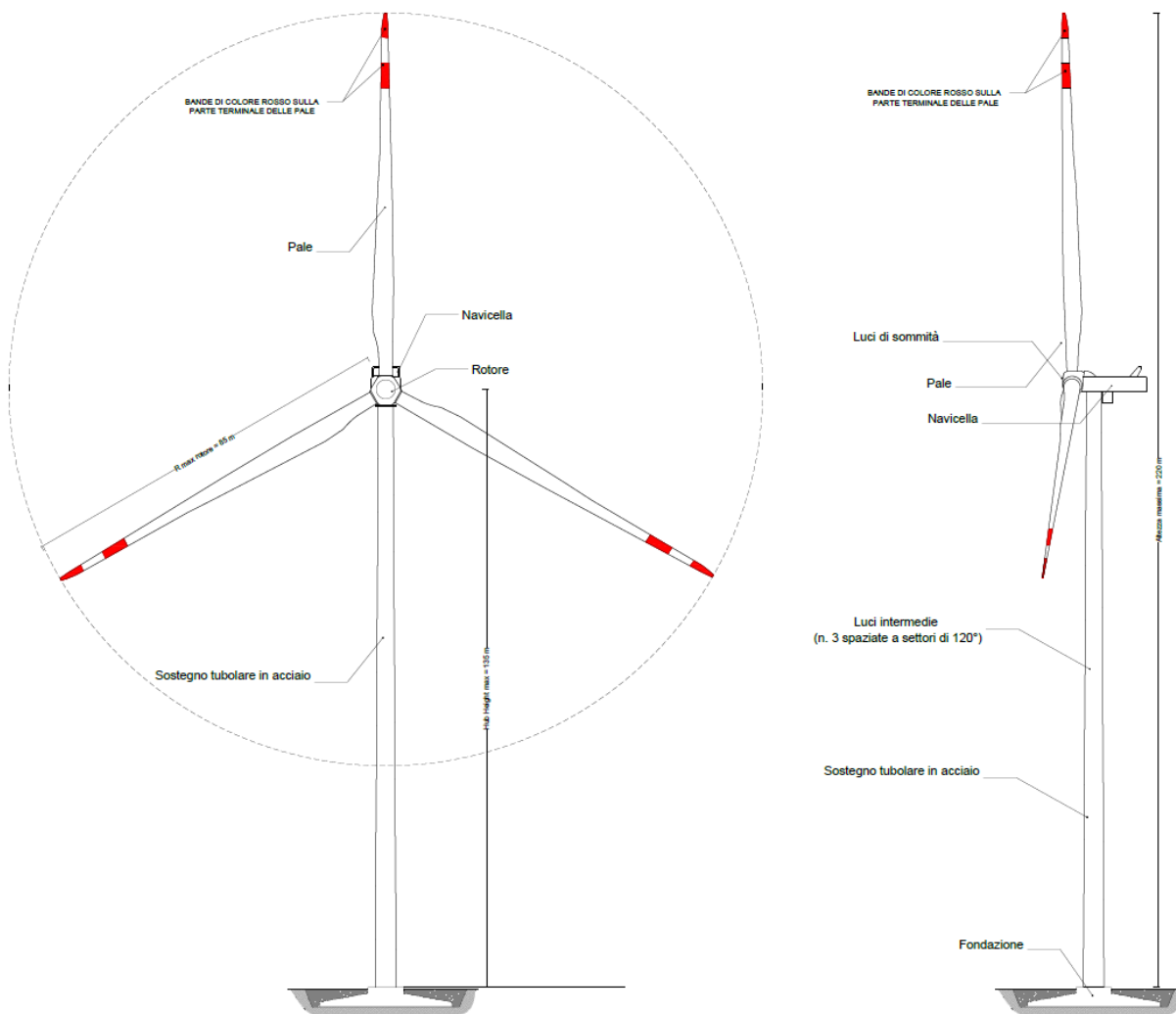
Figura 5.2 – Aerogeneratore tipo SG170 altezza al mozzo (1) 135 m, e diametro rotore (2) di 170 m
