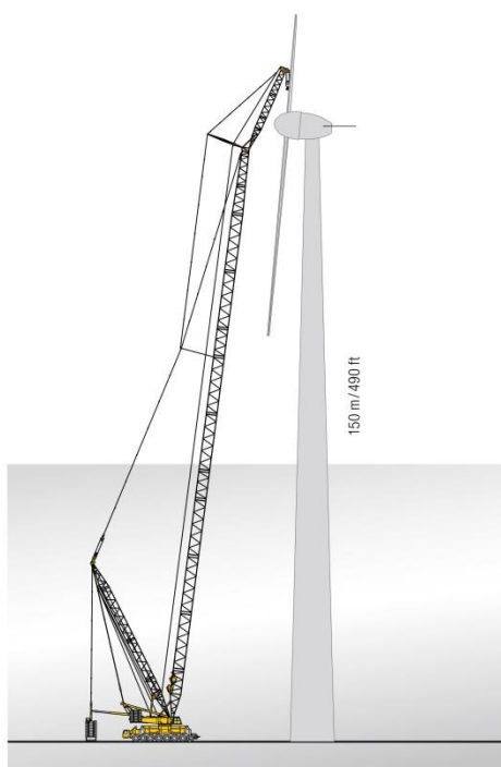
Figura 5.36 – Schema di una gru cingolata a traliccio con sistema derrick impiegata per l'innalzamento delle turbine eoliche dell'ultima generazione
