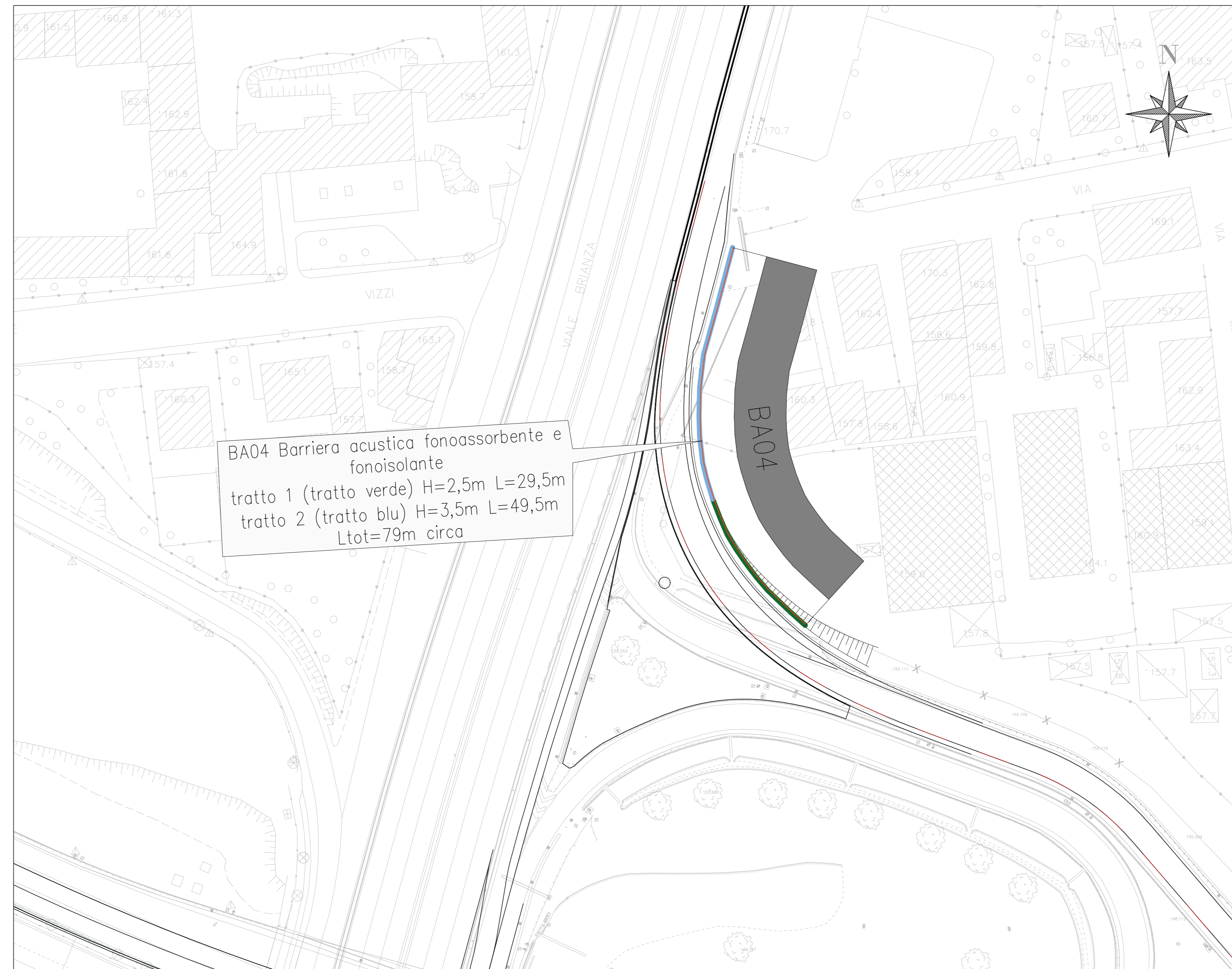
BARRIERA ACUSTICA BA04 - SCALA 1:500
