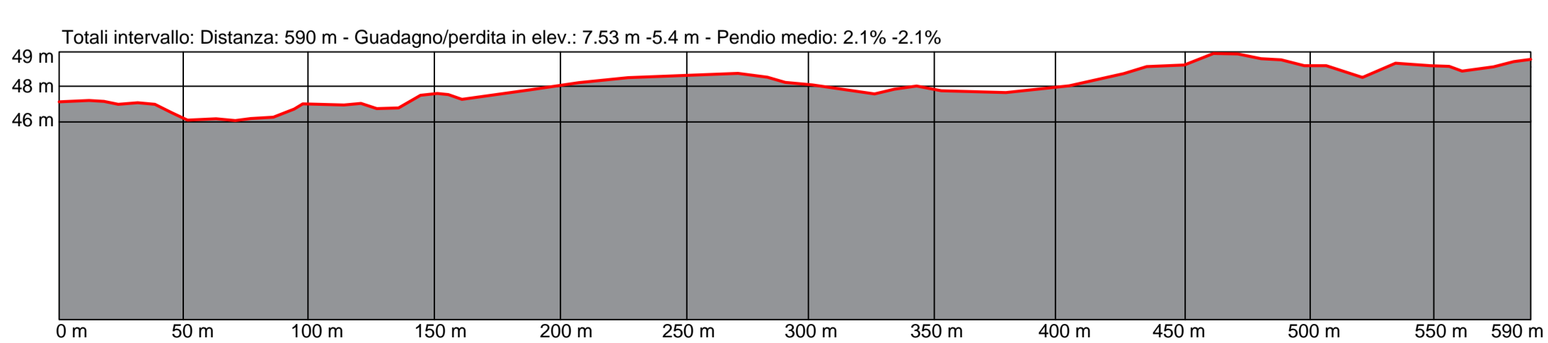
PROFILO I - I'
