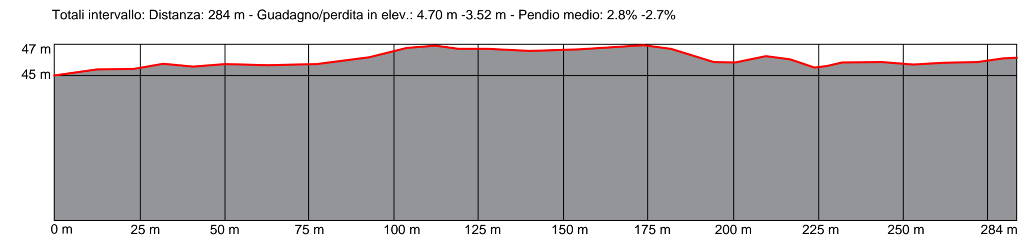
PROFILO L - L'
