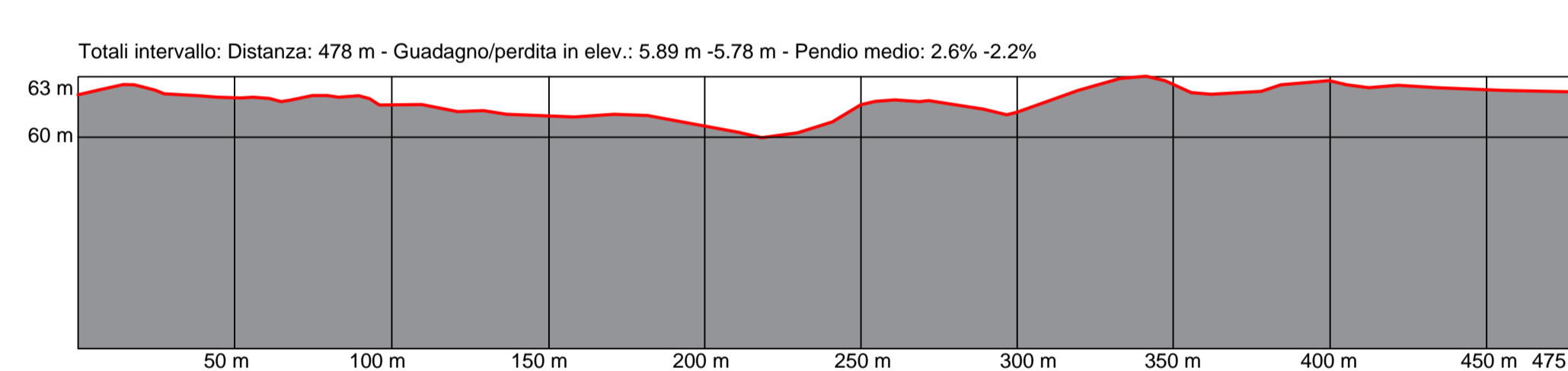
PROFILO D - D'
