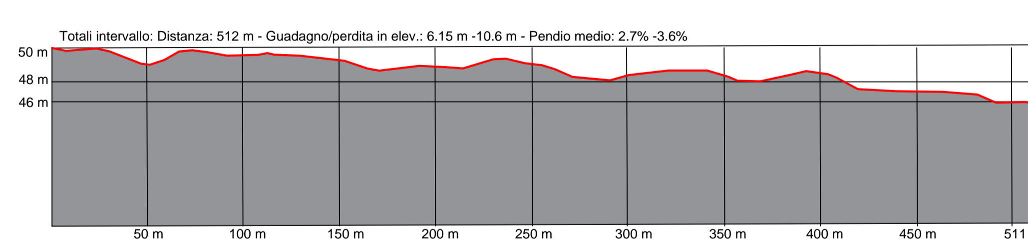
PROFILO F - F'
