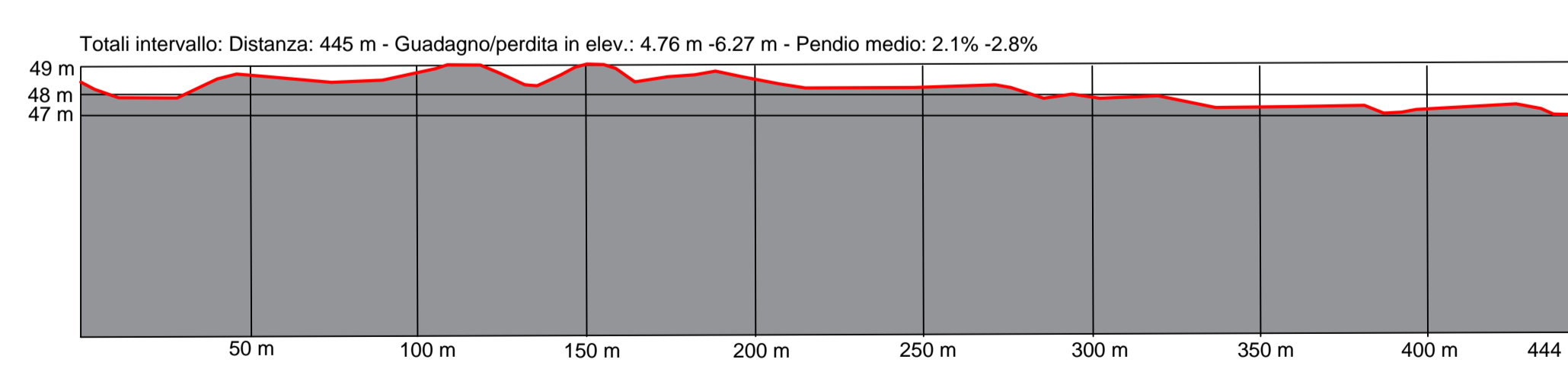
PROFILO H - H'
