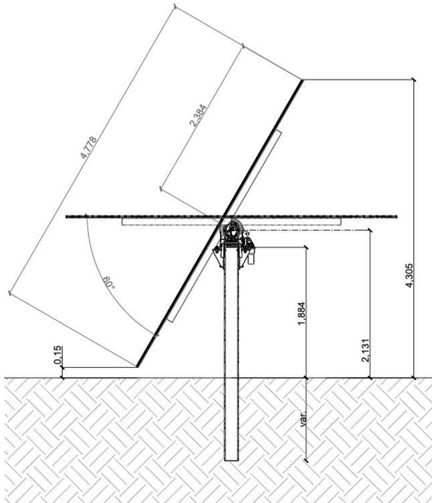
Figura 3 – Prospetto impianto
