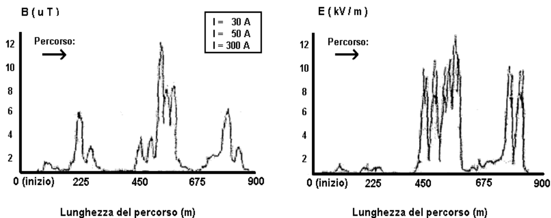
Fig. 2 - Risultati della misura dei campi elettrici e magnetici effettuati lungo le vie interne della sezione a 380 kV della stazione riportata in fig. 1.
