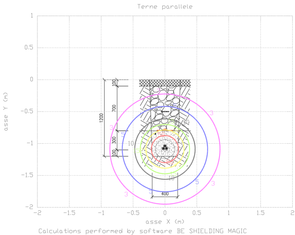
Figura 1 – Livelli di campo magnetico per il solo cavidotto B
