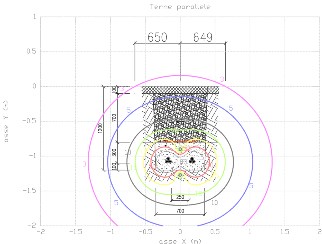
Figura 3 – Livelli di campo magnetico per il solo cavidotto A
