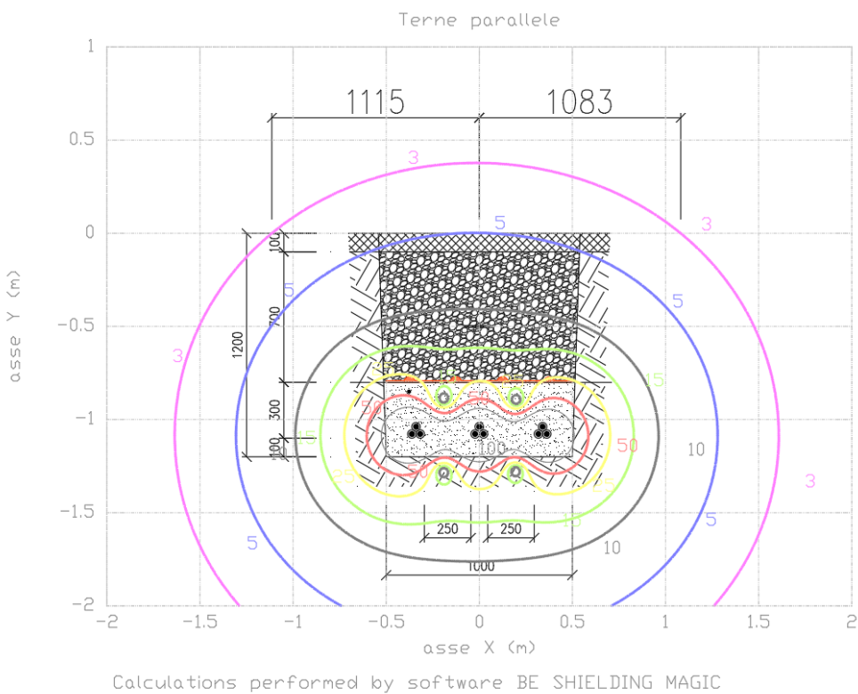
Figura 2 – Livelli di campo magnetico per il tratto in cui i cavidotti A e B sono interrati nel medesimo scavo
