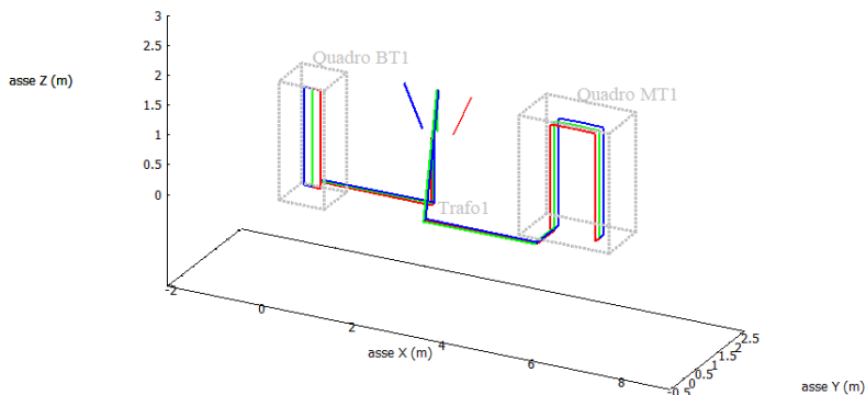
Fig.6 - Modello spaziale cablaggi nelle cabine di trasformazione MT/BT
