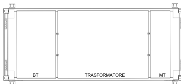
Fig.4 - Ingombri cabine di trasformazione MT/BT
