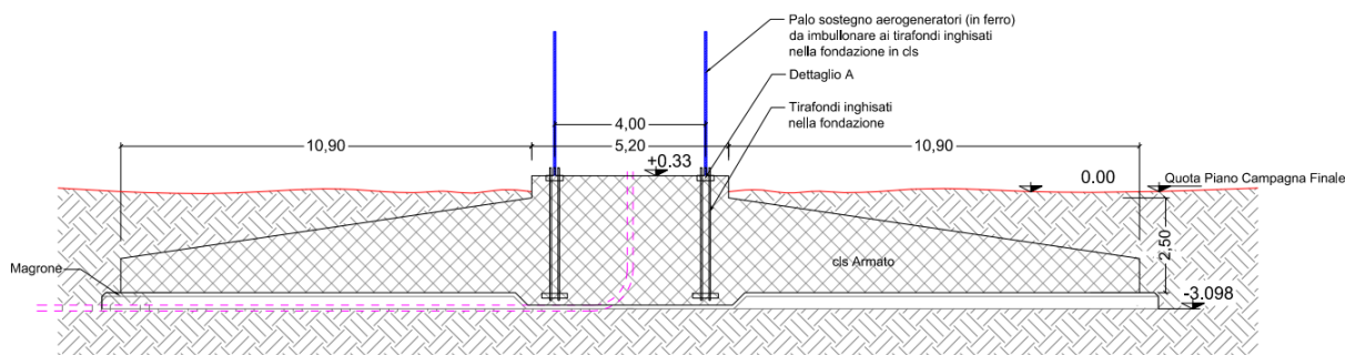
Figura 2-1 – Geometria del plinto di fondazione
