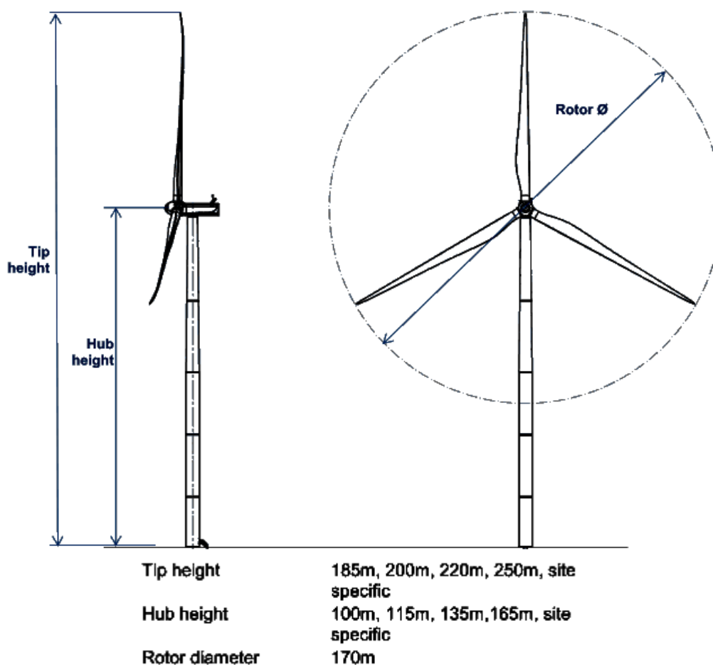
Figura 1-1 – Geometria dell'aerogeneratore Siemens Gamesa SG5.0-170
