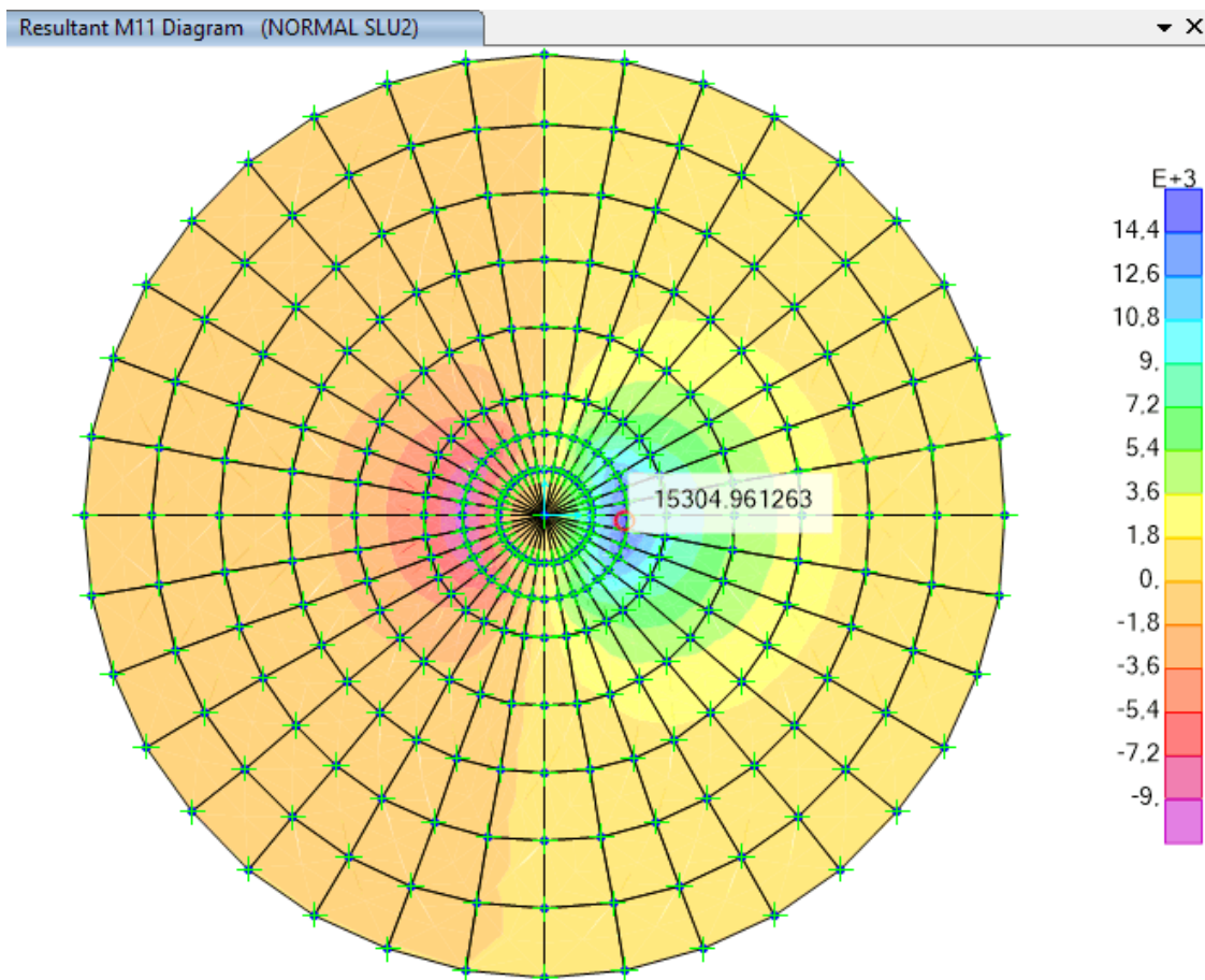
Figura 9-2 – Momento Massimo M11 Normal SLU 2 [kNm/m]
