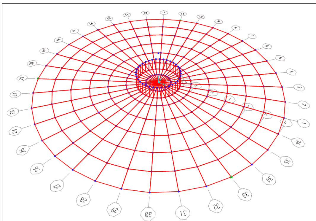
Figura 7-1 – Modello di calcolo della fondazione
