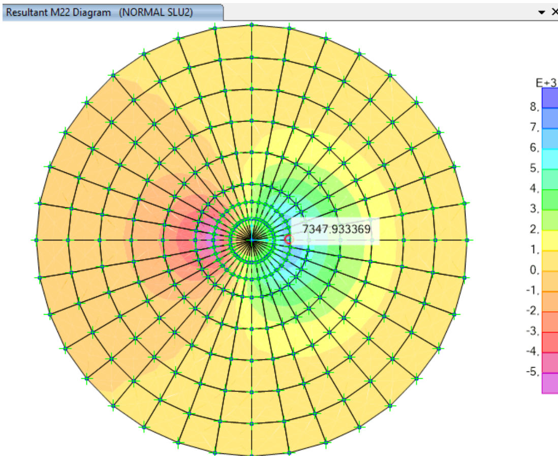
Figura 9-4 – Momento Massimo M22 Normal ELU 2 [kNm/m]
