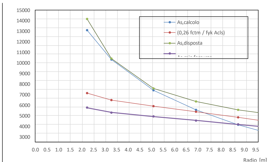
Figura 9-6 – Area armatura radiale inferiore: da calcolo, minima (da norma), effettivamente disposta e da fessurazione
