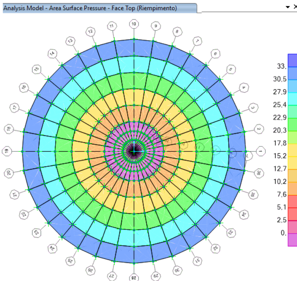
Figura 7-4 – Carico distribuito sul plinto, che simula il peso del terreno di riempimento (a spessore variabile)
