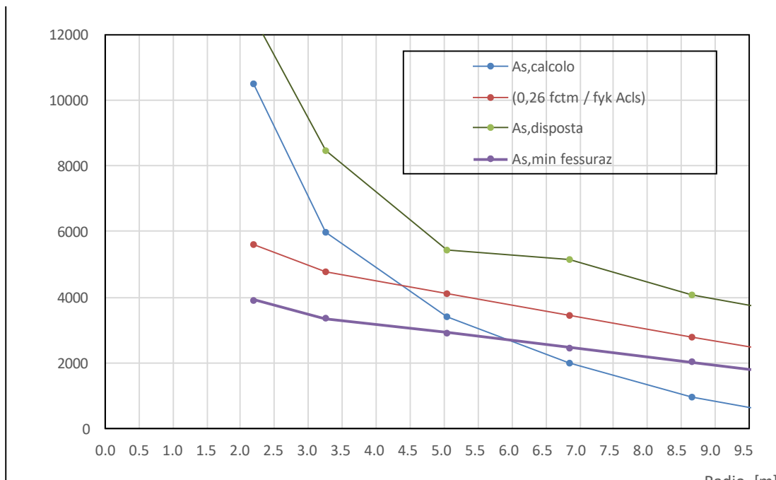
Figura 9-5 – Area armatura radiale superiore: da calcolo, minima (da norma), effettivamente disposta e da fessurazione
