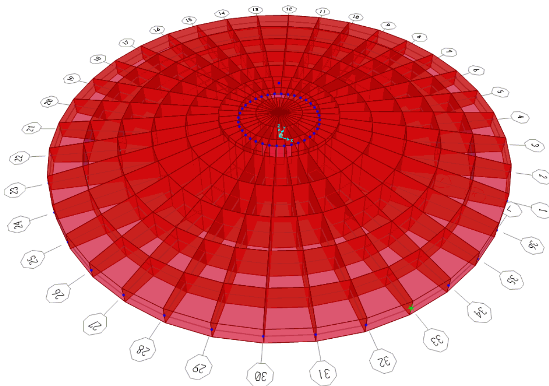
Figura 7-2 – Modello FEM della fondazione – vista solida
