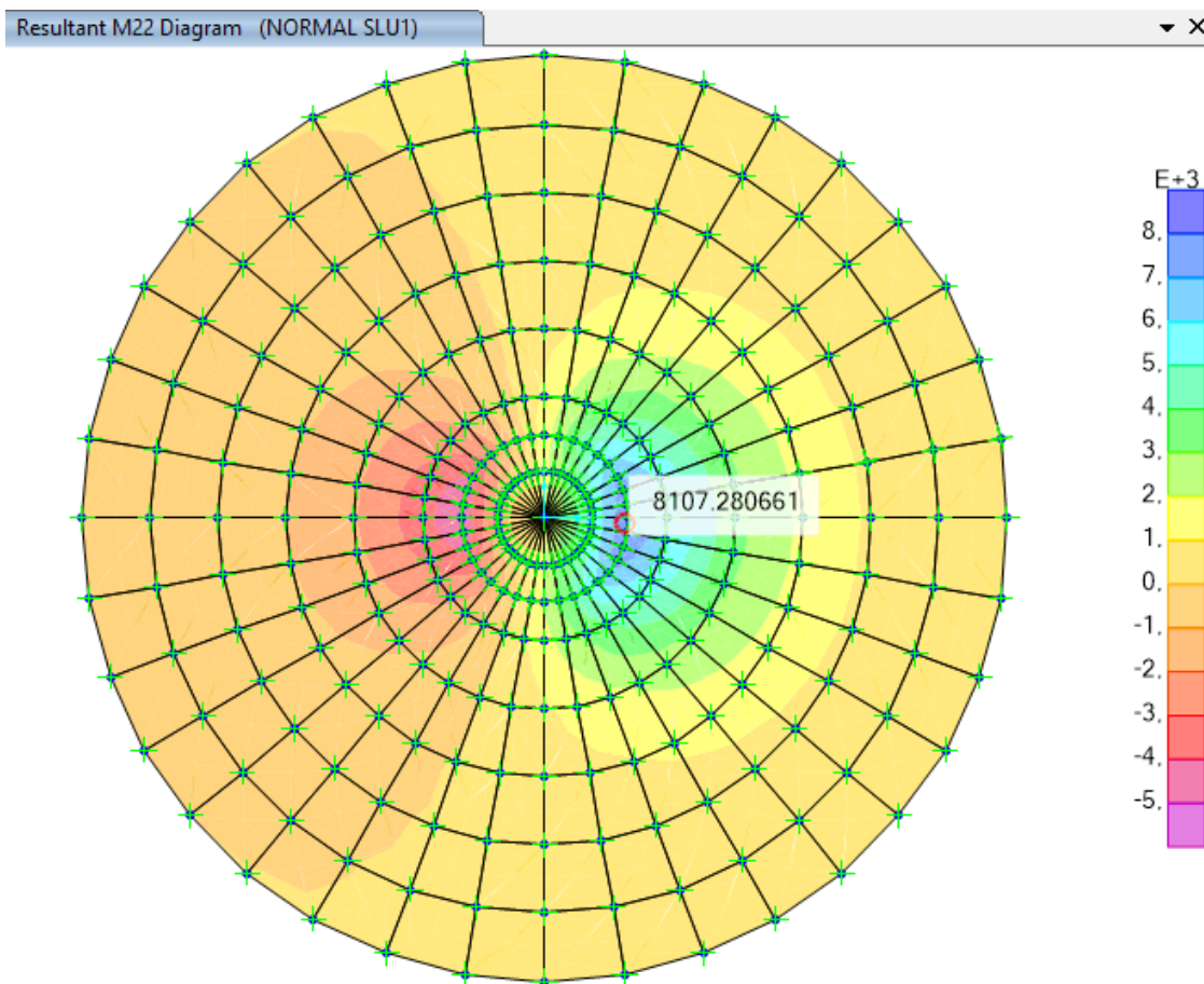
Figura 9-3 – Momento Massimo M22 Normal SLU 1 [kNm/m]
