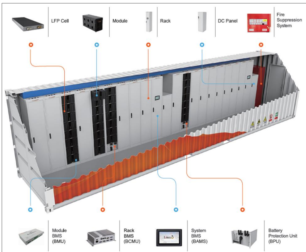
Figura 19: Particolare spaccato sistema di accumulo BESS
