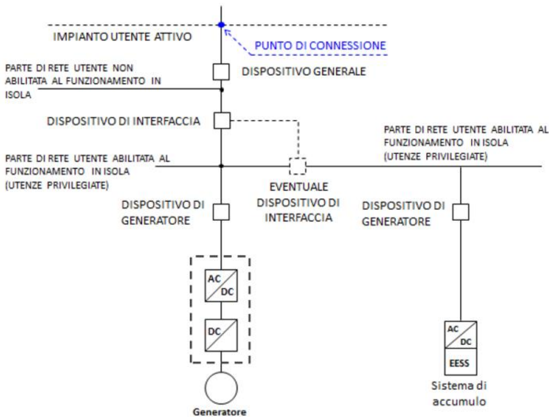
Figura 1: schema tipico di sistema impianto fotovoltaico integrato da un sistema di accumulo in configurazione AC-Coupling
