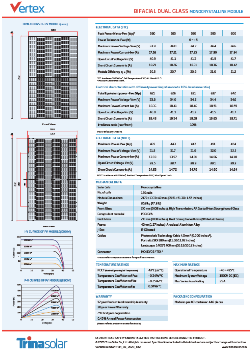
Figura 4: Datasheet moduli fotovoltaici
