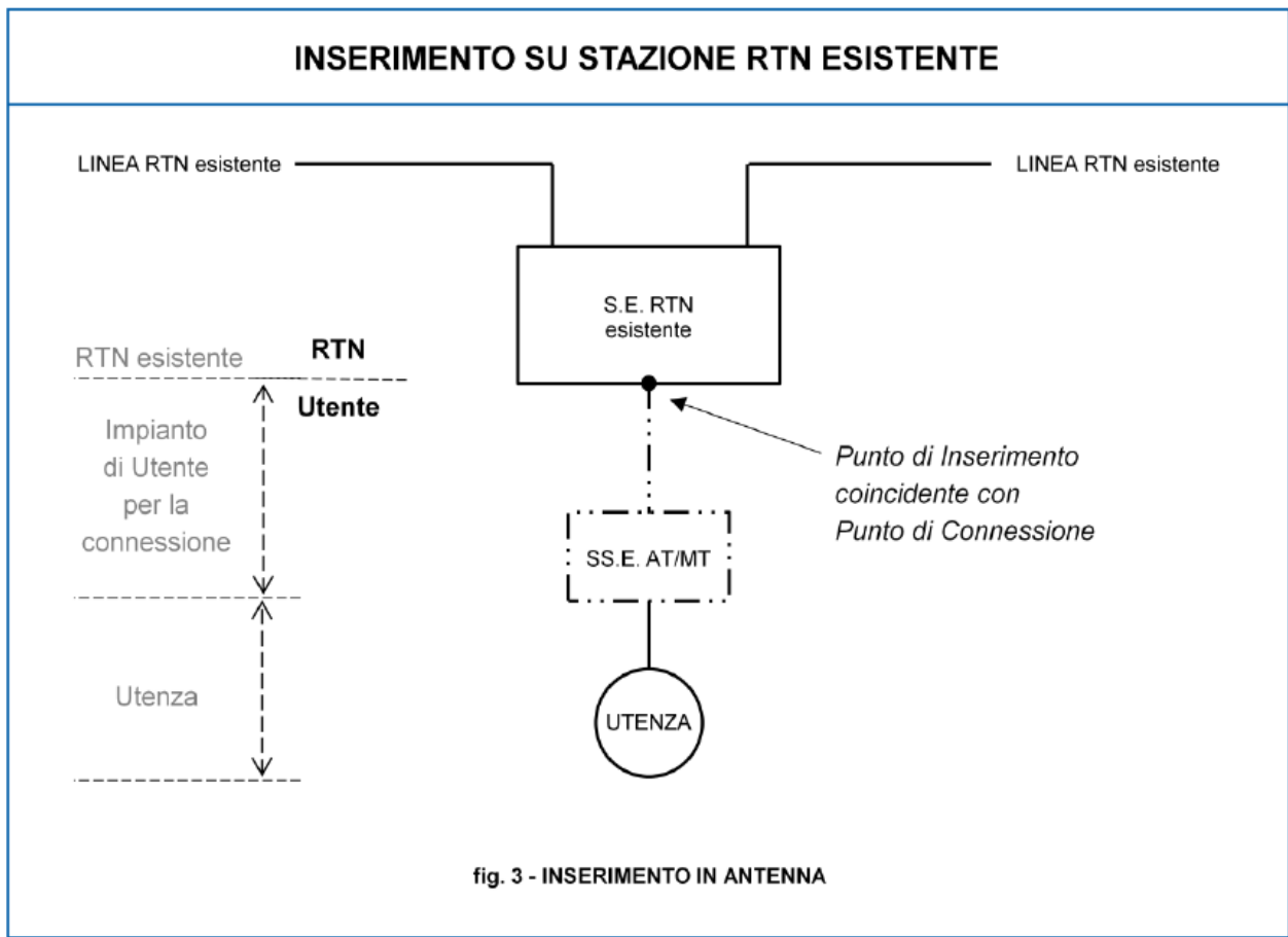
Figura 2: schema tipico di inserimento in antenna su Stazione RTN esistente
