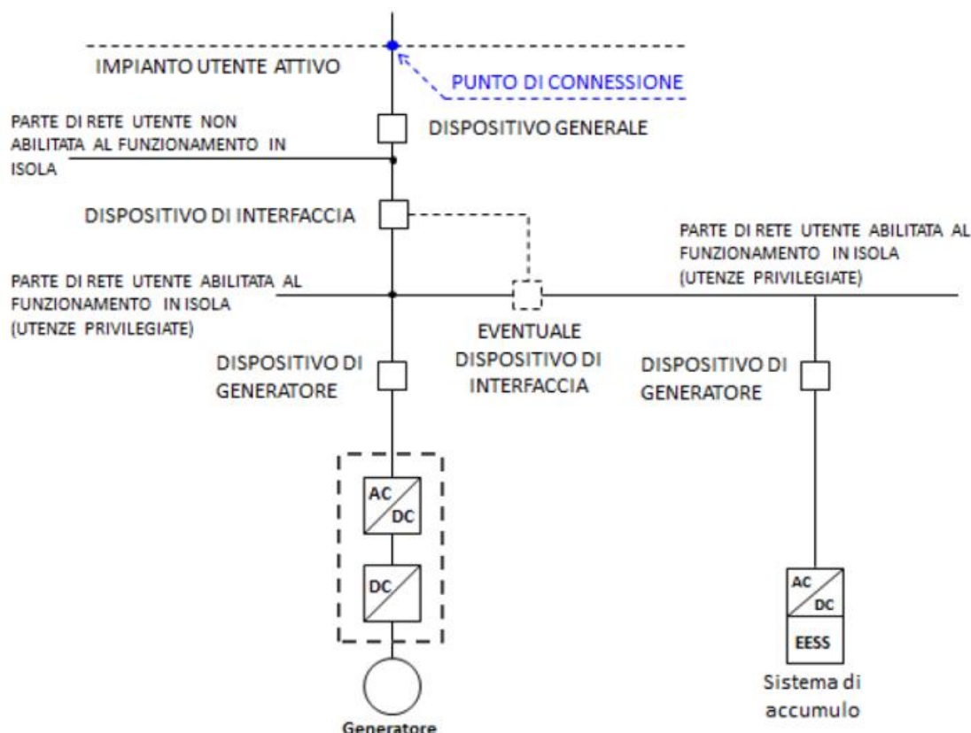
Figura 3: schema tipico di sistema impianto fotovoltaico integrato da un sistema di accumulo in configurazione AC-Coupling
