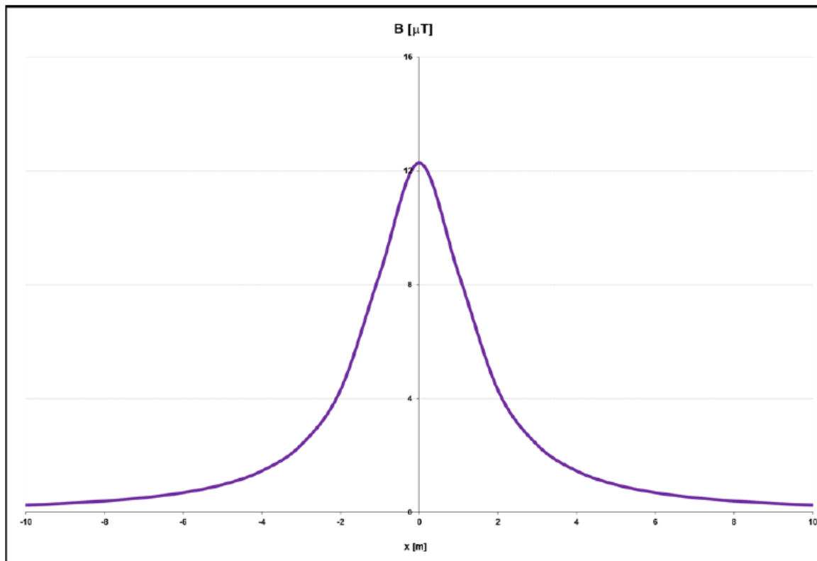
Figura 14: induzione magnetica generata durante l'esercizio dalla linea valutata applicando la procedura delle Norma CEI 211-4 – Guida ai metodi di calcolo dei campi elettrici e magnetici generati da linee elettriche
