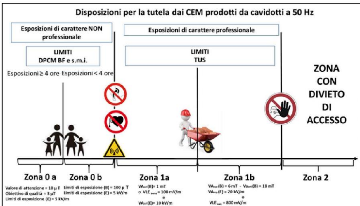
Figura 15: Misure di prevenzione e protezione per la tutela dai CEM prodotti da cavidotti a 50 Hz
