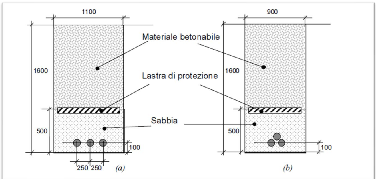
Figura 20: schermatura cavi elettrici interrati
