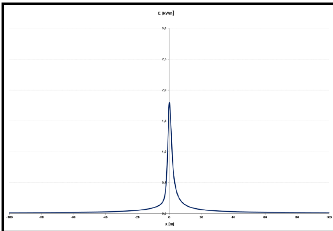
Figura 13: Campo elettrico generato dalla Linea durante l'esercizio valutato applicando la procedura della Norma CEI 211-4 - Guida ai metodi di calcolo dei campi elettrici e magnetici generati da linee elettriche
