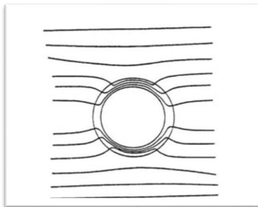
Figura 19: andamento qualitativo della deformazione delle linee di forza di un campo magnetico uniforme per effetto di un nucleo in materiale ferromagnetico
