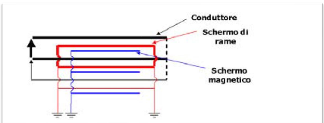
Figura 21: schema bidimensionale del cavo unipolare e della messa a terra degli schermi- tecnica "solid bonding"
