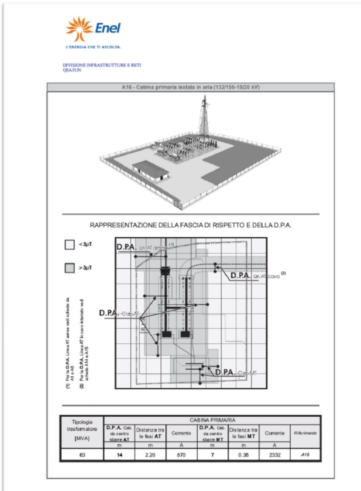
Figura 9: DPA Cabina Primaria AT/MT Enel equipaggiata con n° 2 trasformatori AT/MT da 63 MVA- Linea Guida per l'applicazione del § 5.1.3 dell'Allegato al D.M. 29.05.08 – Distanza di prima approssimazione da linee e cabine elettriche
