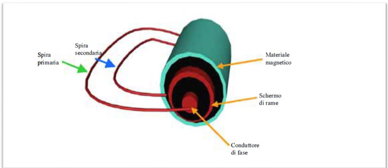
Figura 22: schema tridimensionale del cavo a debole emissione di campo magnetico- tecnica "Solid-bonding"
