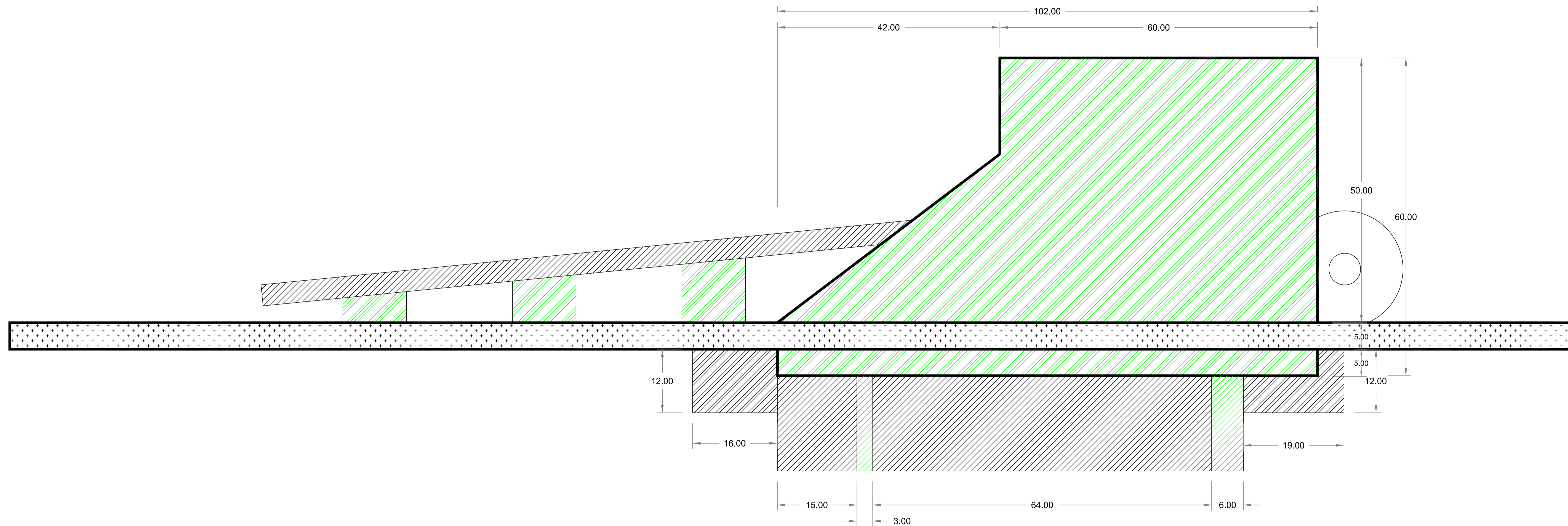
PIAZZOLA DI MONTAGGIO "TIPO" PIANTA SCHEMATICA
