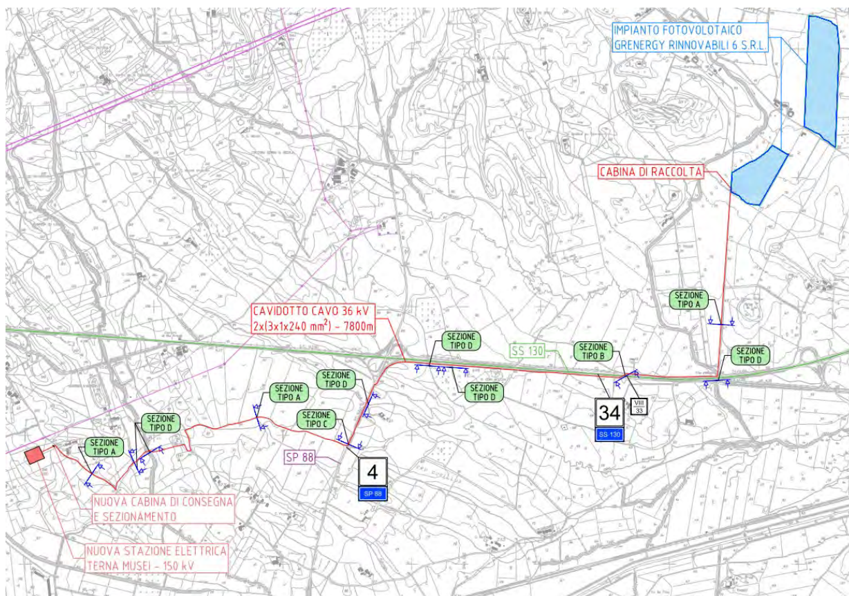
Figura 1 Inquadramento su CTR con identificazione area di pertinenza
