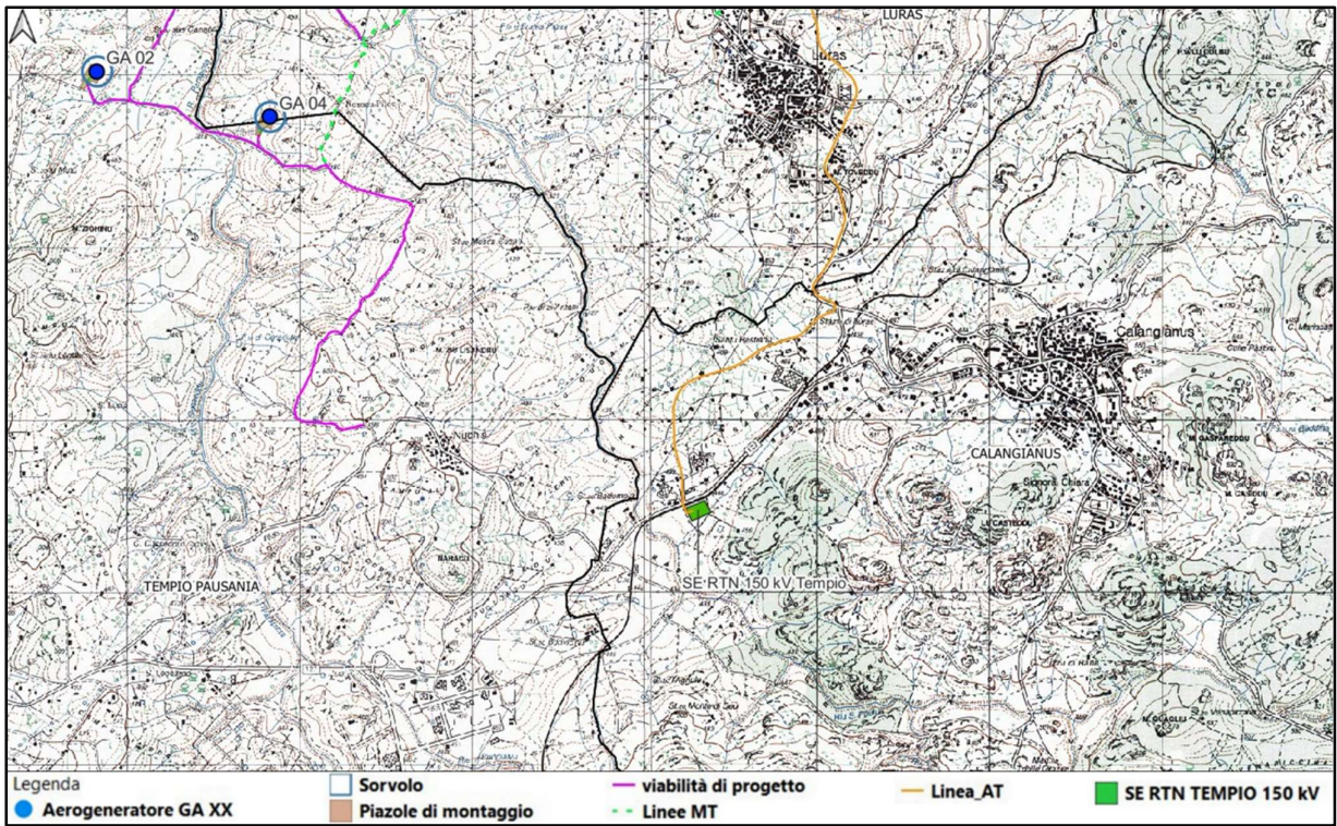
Figura 6.3.6.1: Individuazione su IGM della Stazione RTN 150 kV “Tempio” di futura realizzazione
