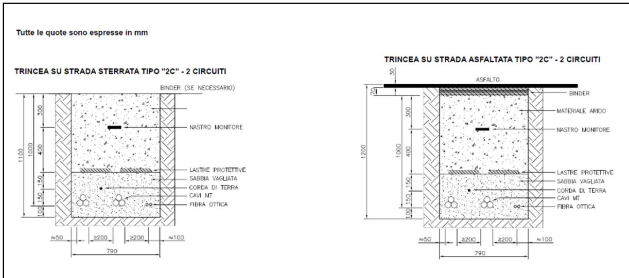
Figura 6.3.3.3: Sezioni tipiche delle trincee cavidotto per due terne di cavi in parallelo su strada sterrata e asfaltata
