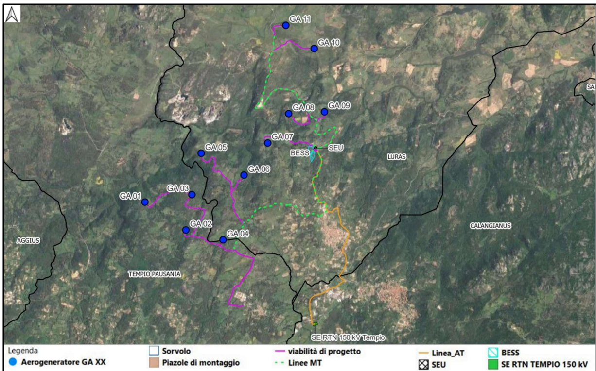
Figura 6.3: Inquadramento territoriale dell'impianto eolico Gallura su ortofoto con i limiti amministrativi dei comuni interessati
