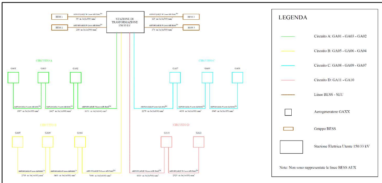
Figura 6.3.3.1: Schema a blocchi del Parco Eolico Gallura
