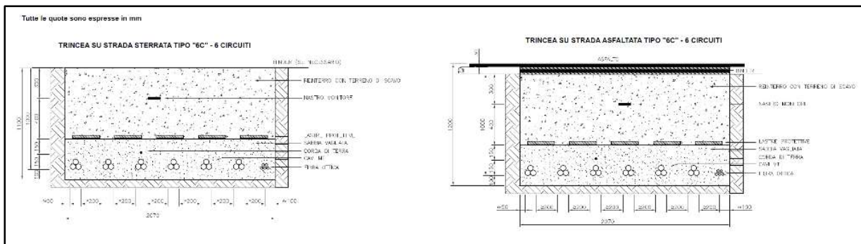
Figura 6.3.3.7: Sezioni tipiche delle trincee cavidotto per sei terne di cavi in parallelo su strada sterrata e asfaltata
