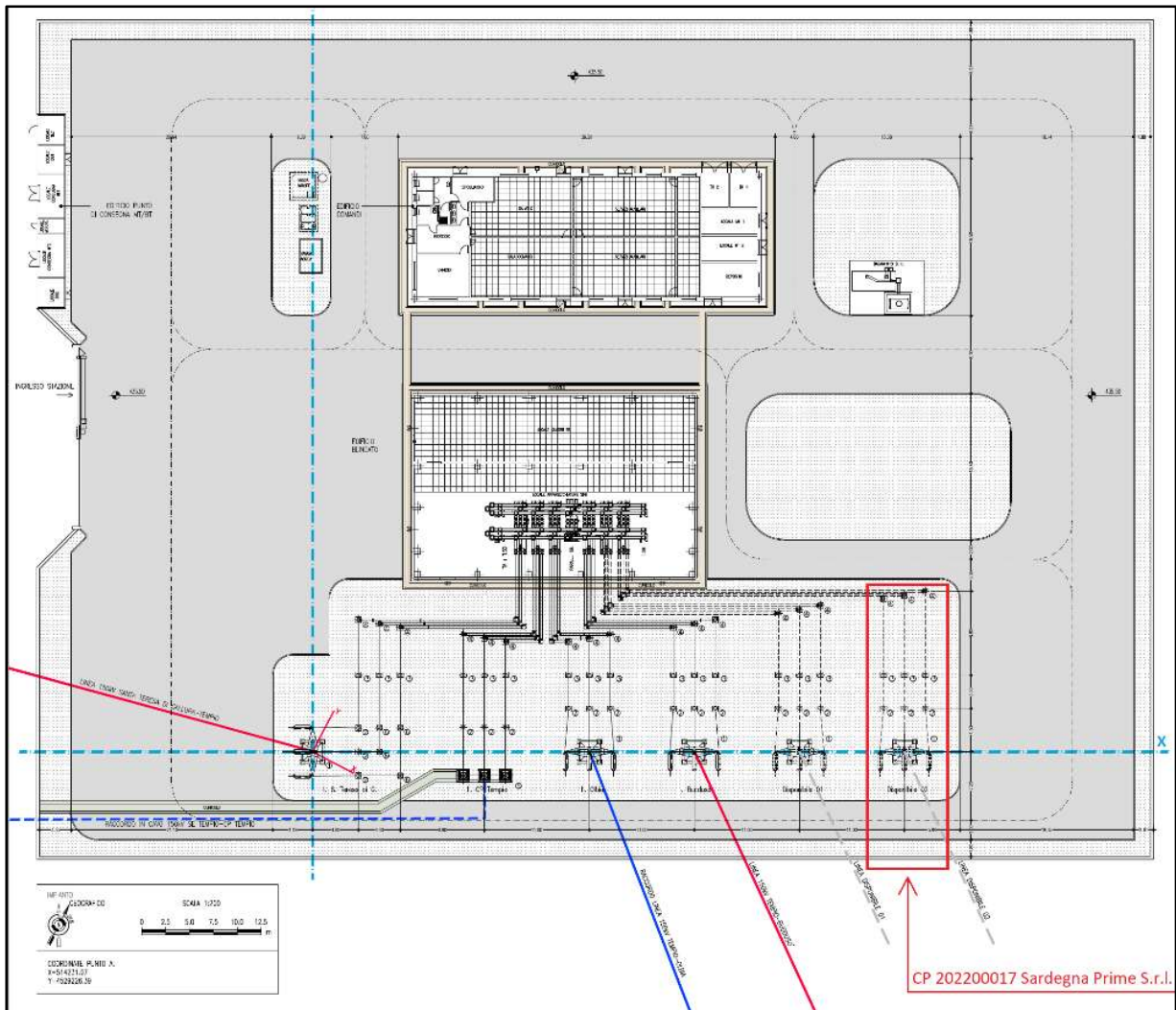
Figura 6.3.6.2: Planimetria della SE RTN a 150 kV “Tempio” con l’ubicazione dello stallo a 150 kV
