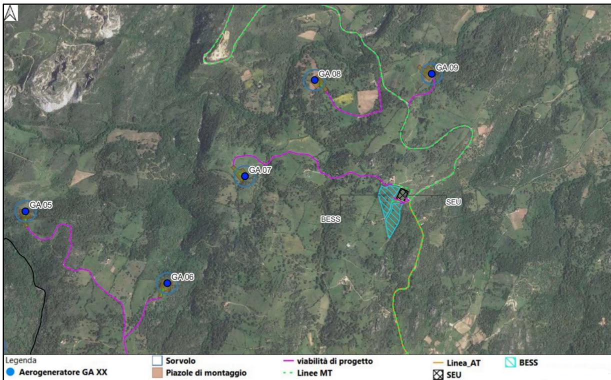
Figura 6.3.4.1: Localizzazione SEU 150/33 kV e BESS su ortofoto
