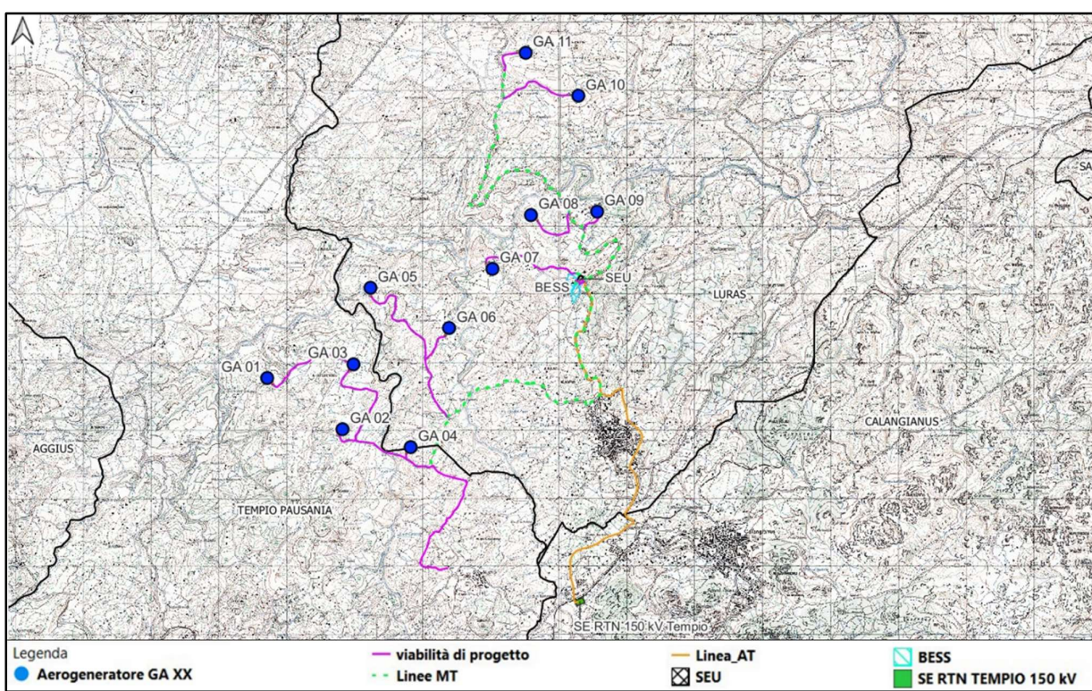
Figura 6.1: Inquadramento territoriale dell'impianto eolico Gallura su IGM con i limiti amministrativi dei comuni interessati
