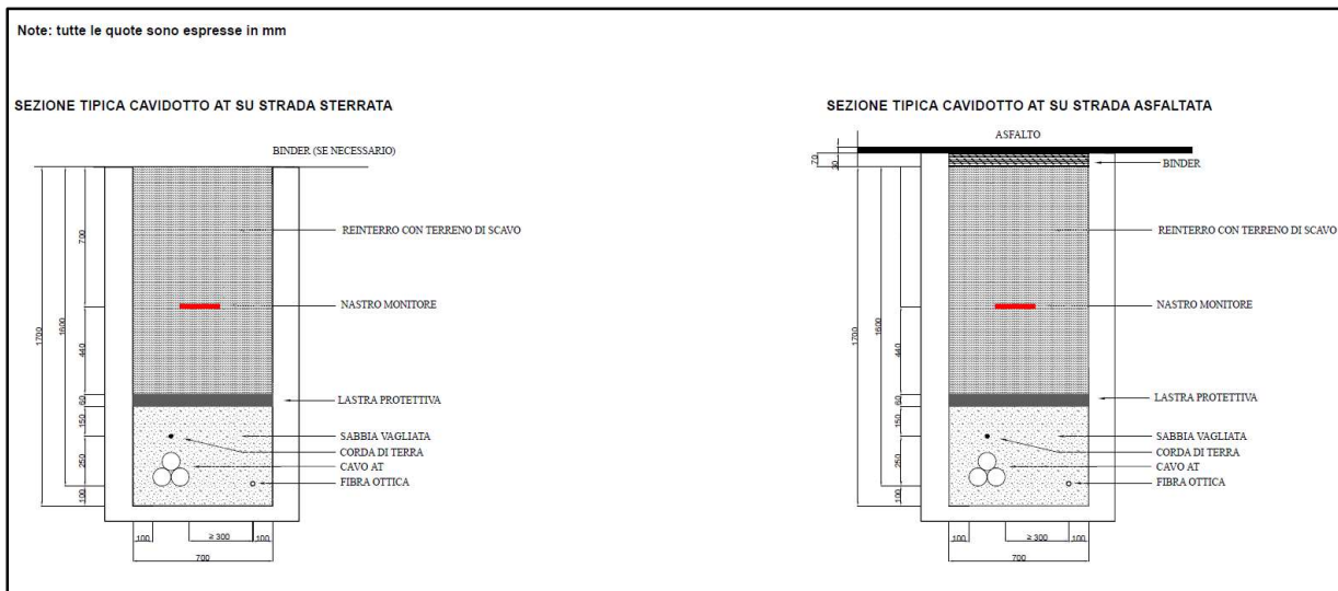
Figura 6.3.5.1: Sezione tipica del cavidotto AT di connessione tra la SEU 150/33 kV e il nuovo stallo della Stazione Elettrica della RTN 150 kV denominata "Tempio"
