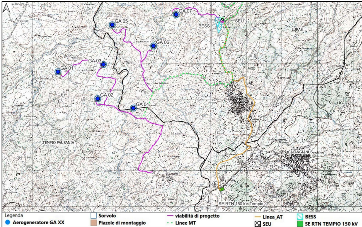
Figura 6.2: Soluzione di connessione a 150 kV in corrispondenza della stazione elettrica RTN Terna 150 kV Tempio (di futura realizzazione)
