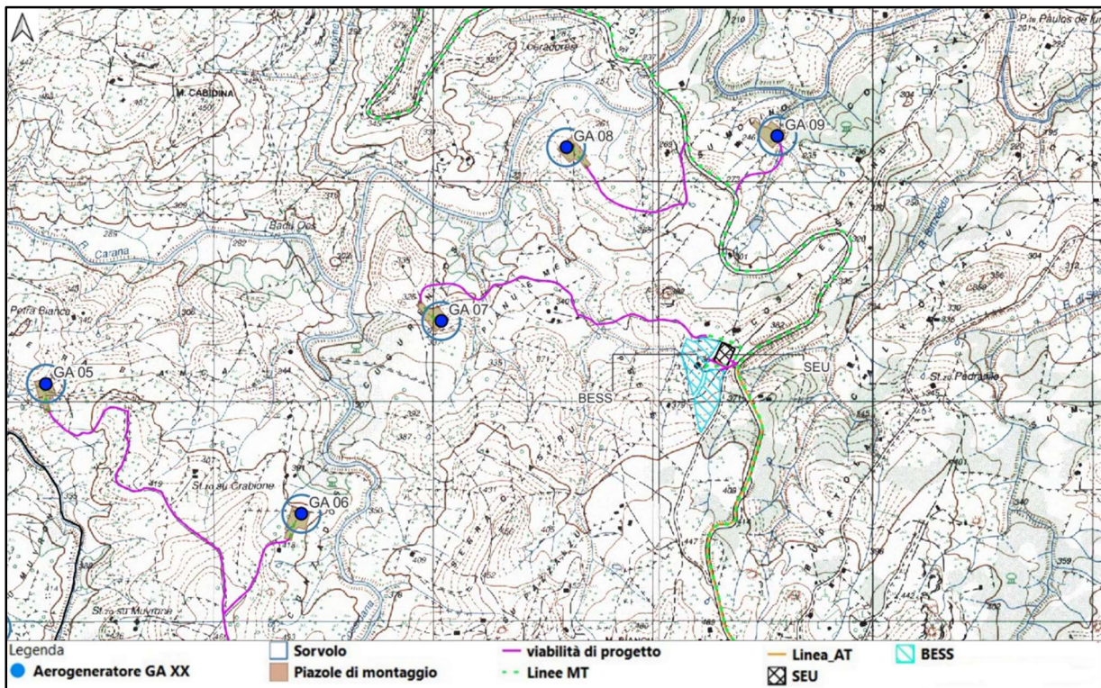
Figura 6.3.2.1: Localizzazione della SEU 150/33 kV e del BESS su IGM
