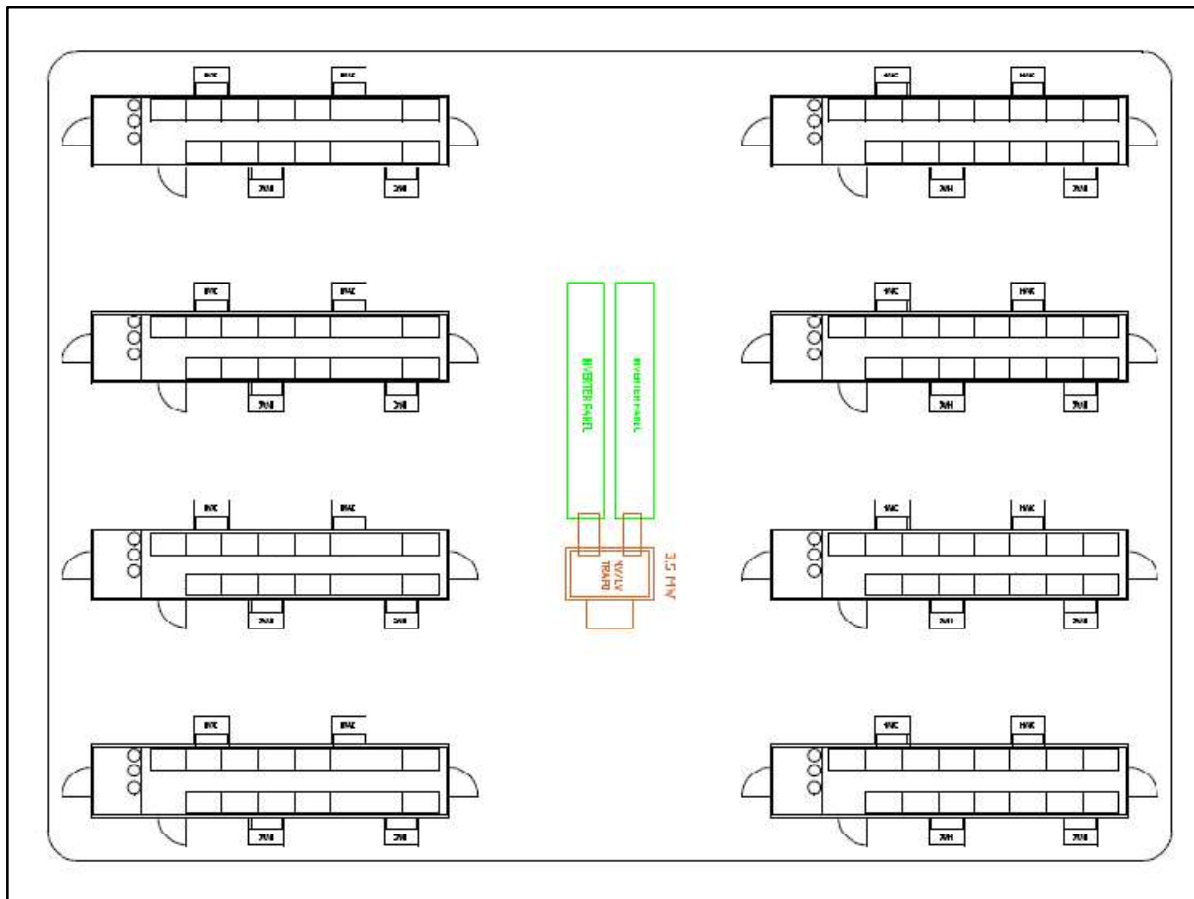
Figura 6.3.4.2: Unità base da 4,0 MW del BESS
