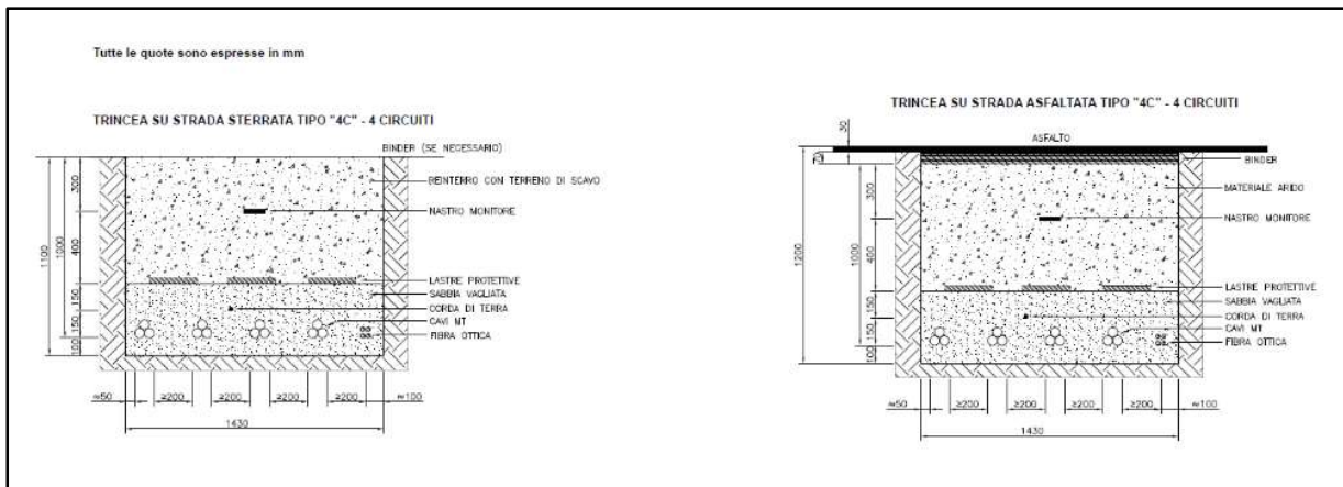
Figura 6.3.3.5: Sezioni tipiche delle trincee cavidotto per quattro terne di cavi in parallelo su strada sterrata e asfaltata
