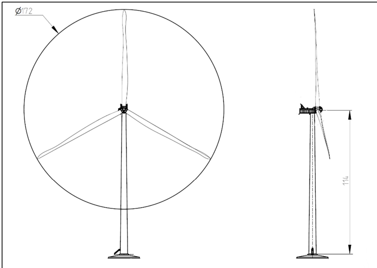
Figura 6.1.1: Profilo aerogeneratore V172 – 7,2 MW – HH= 114 m – D=172 m
