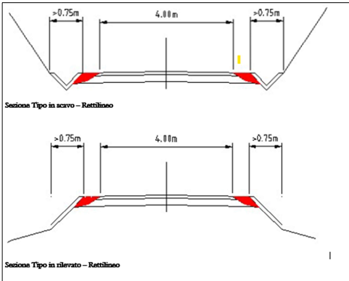
Figura 6.2.1: Sezioni tipo viabilità parco eolico
