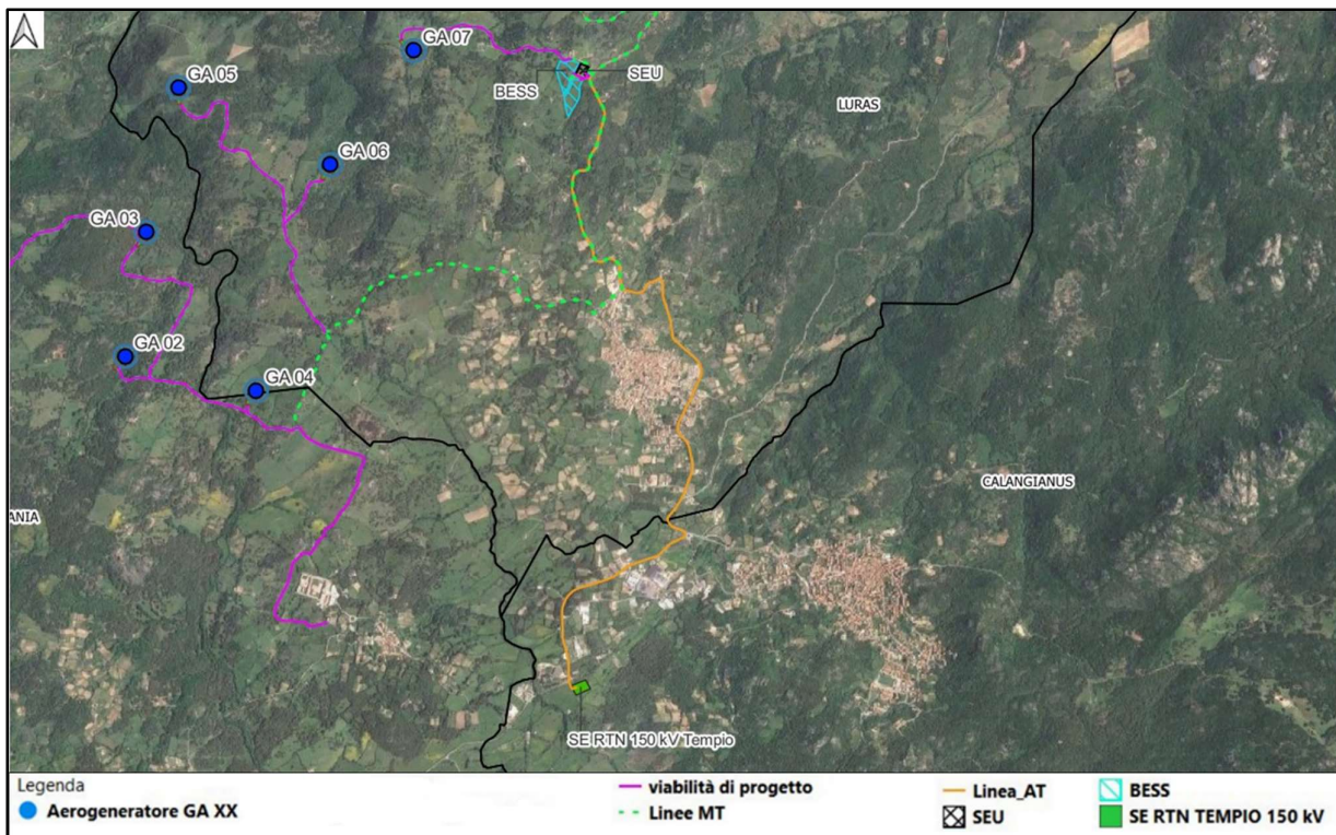
Figura 6.3.2.2: Localizzazione della SEU 150/33 kV, del BESS e della SE RTN 150 kV Tempio su ortofoto
