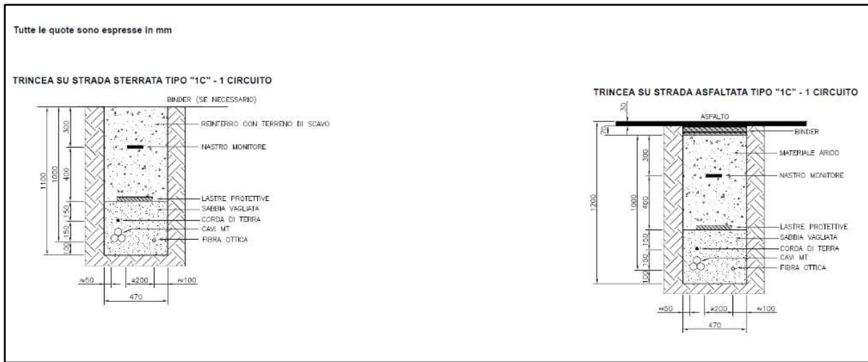
Figura 6.3.3.2: Sezioni tipiche delle trincee cavidotto per una terna di cavi in parallelo su strada sterrata e asfaltata
