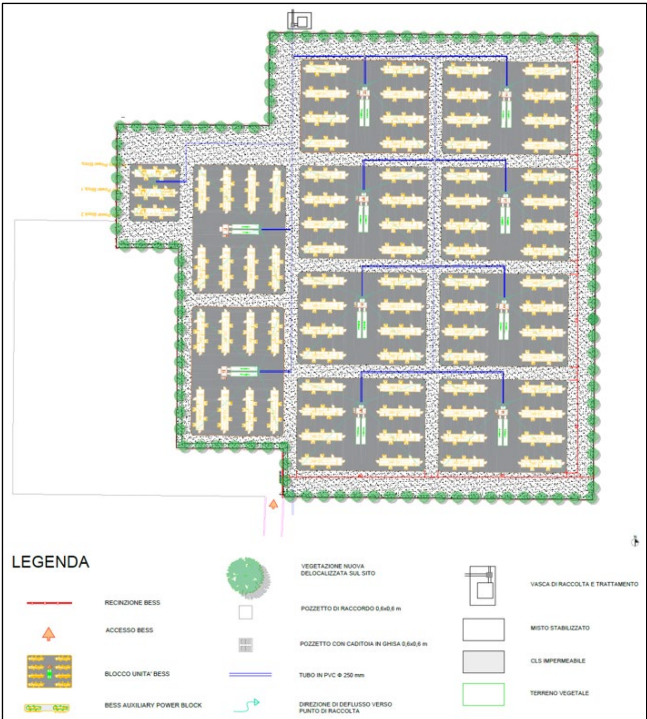
Figura 11.1: Planimetria architettonica BESS con sistema di smaltimento acque e rappresentazione degli alberi lungo il perimetro
