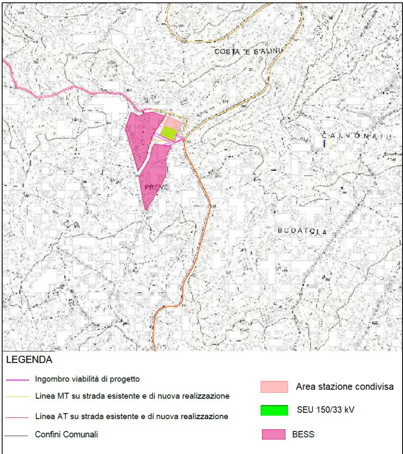
Figura 9.1.1: Area stazione condivisa, SEU 150/33 kV e BESS 64,8 MWp su CTR
