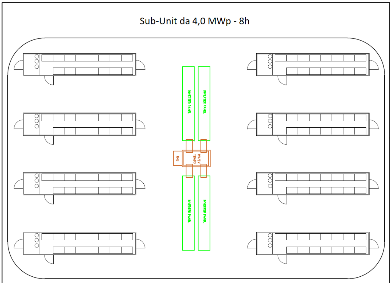
Figura 9.1.3: Unità base da 4,0 MWp - 8h del BESS
