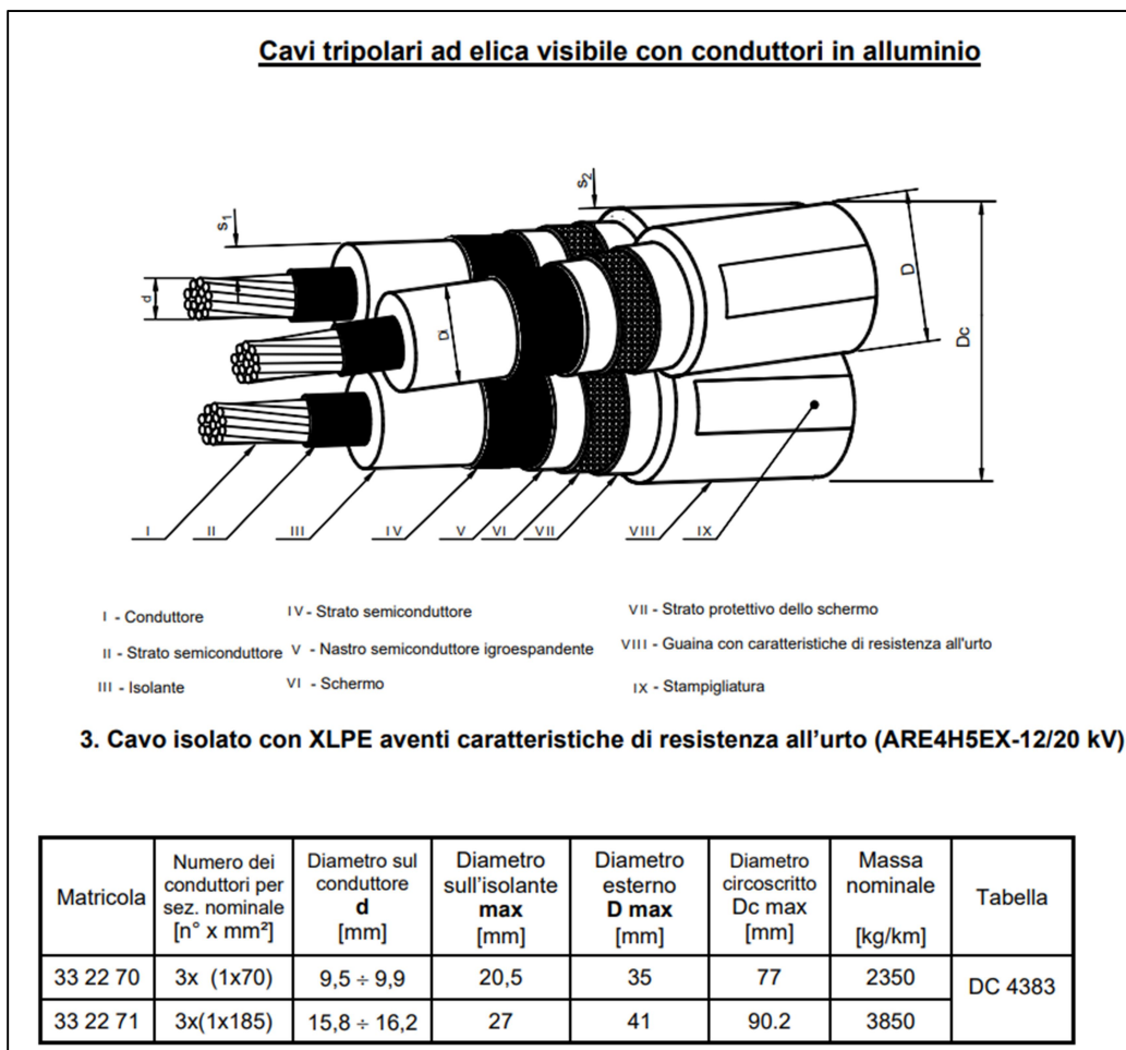
Figura 3 – Tipologia di cavo da 185 mmq da specifiche tecniche di E-Distribuzione
