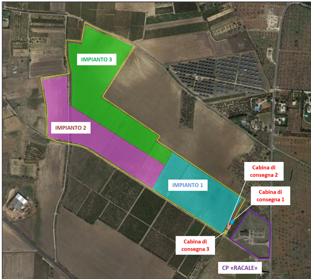
Figura 1 – Stralcio su ortofoto con indicazione dell'area dell'impianto FV – cabine di consegna- area CP "Racale"
