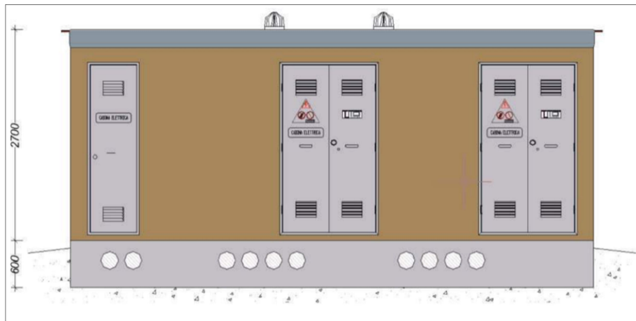
Figura 6 – Vista della cabina di consegna tipo
