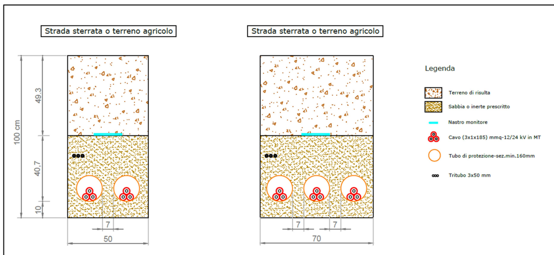
Figura 5 – Sezioni degli scavi previste nel progetto
