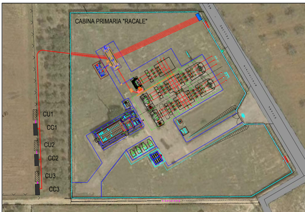
Figura 2 – Stralcio su ortofoto con indicazione delle opere di connessione alla rete MT-cavidotto in MT con n.3 terne cavi interrati di connessione tra le cabine di consegna e la CP (in rosso)
