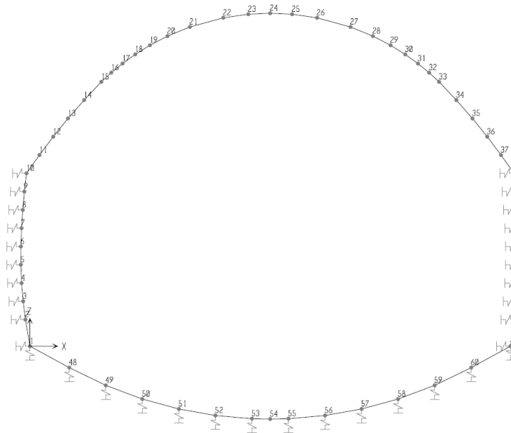
Figura 4: Numerazione dei nodi del modello e disposizione molle terreno
