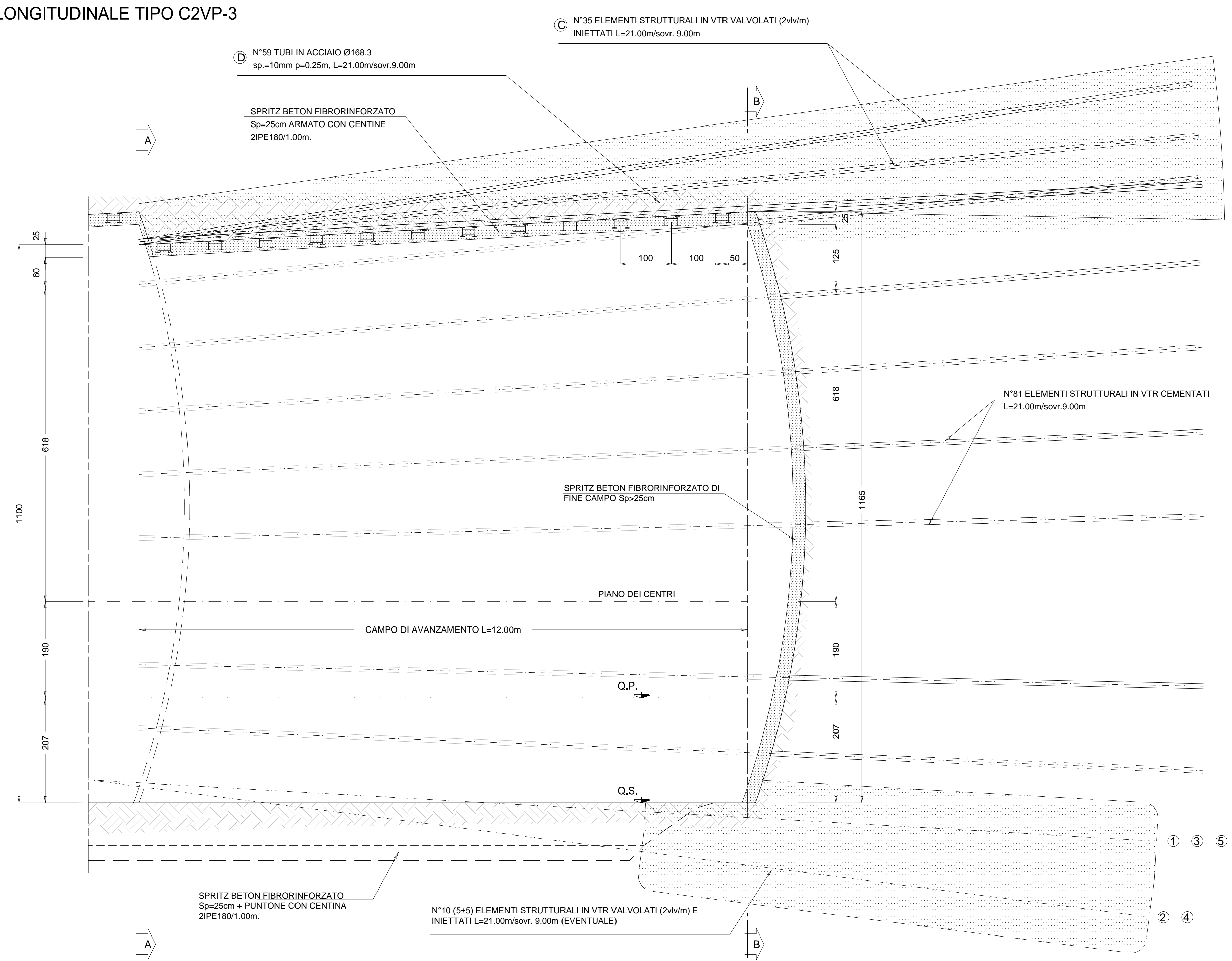
N.B. LE INCLAZIONI RADIALI RIPORTATE IN TABELLA SONO DA RIFERIRSI ALLA LIVELLETTA STRADALE
