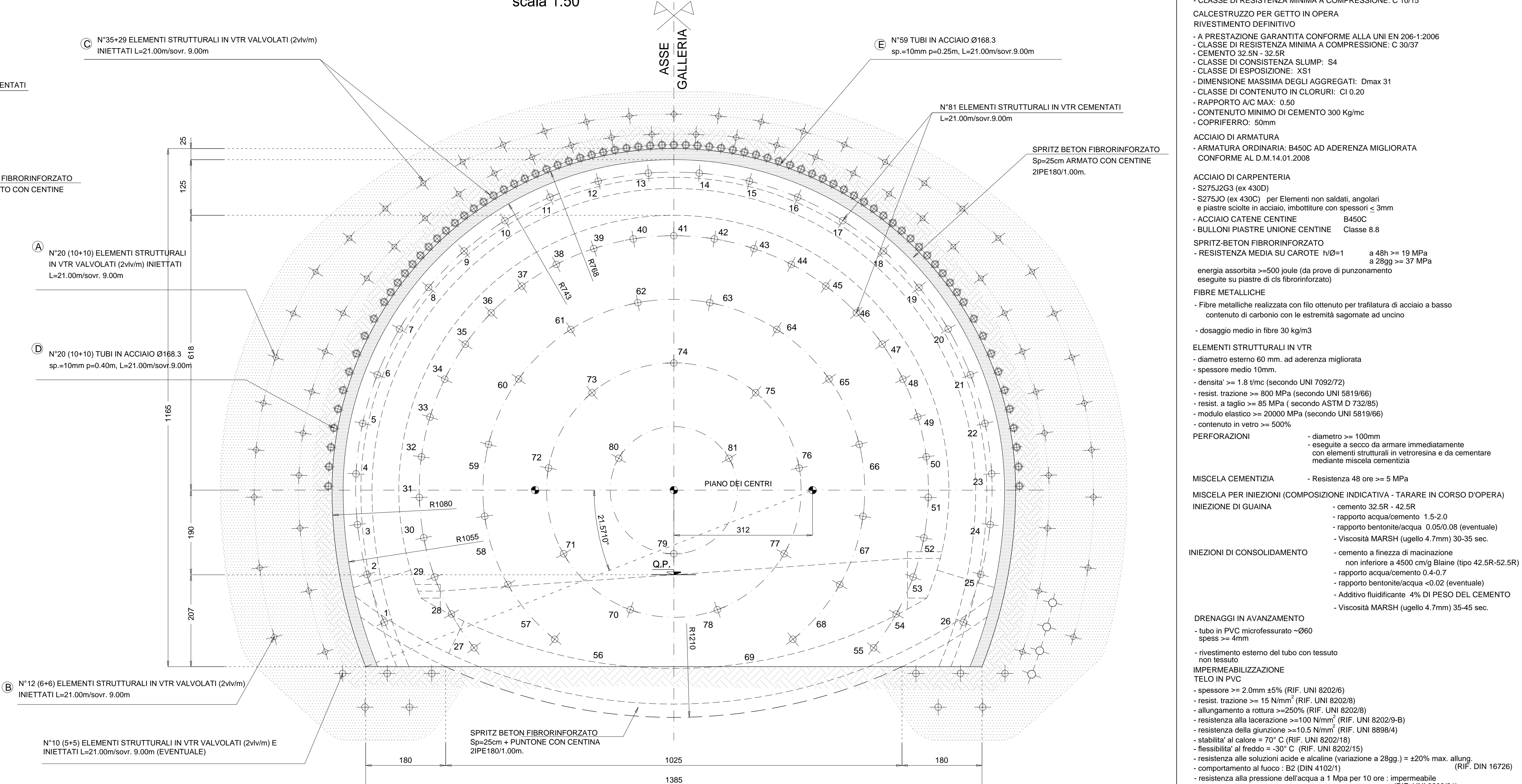
SEZIONE TRASVERSALE B-B (CAMPO FINALE) scala 1:50
