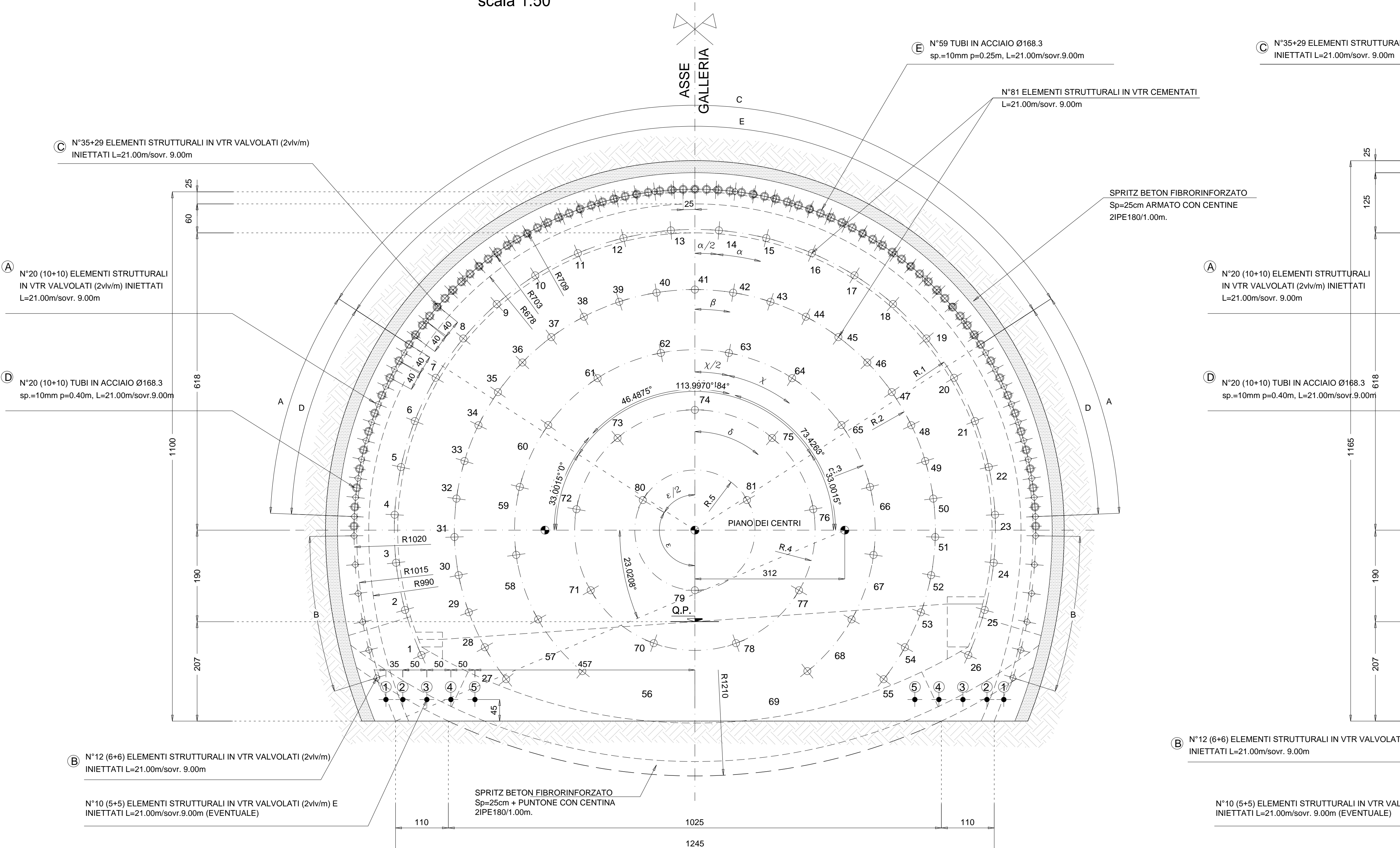
SEZIONE TRASVERSALE A-A (CAMPO INIZIALE) scala 1:50
