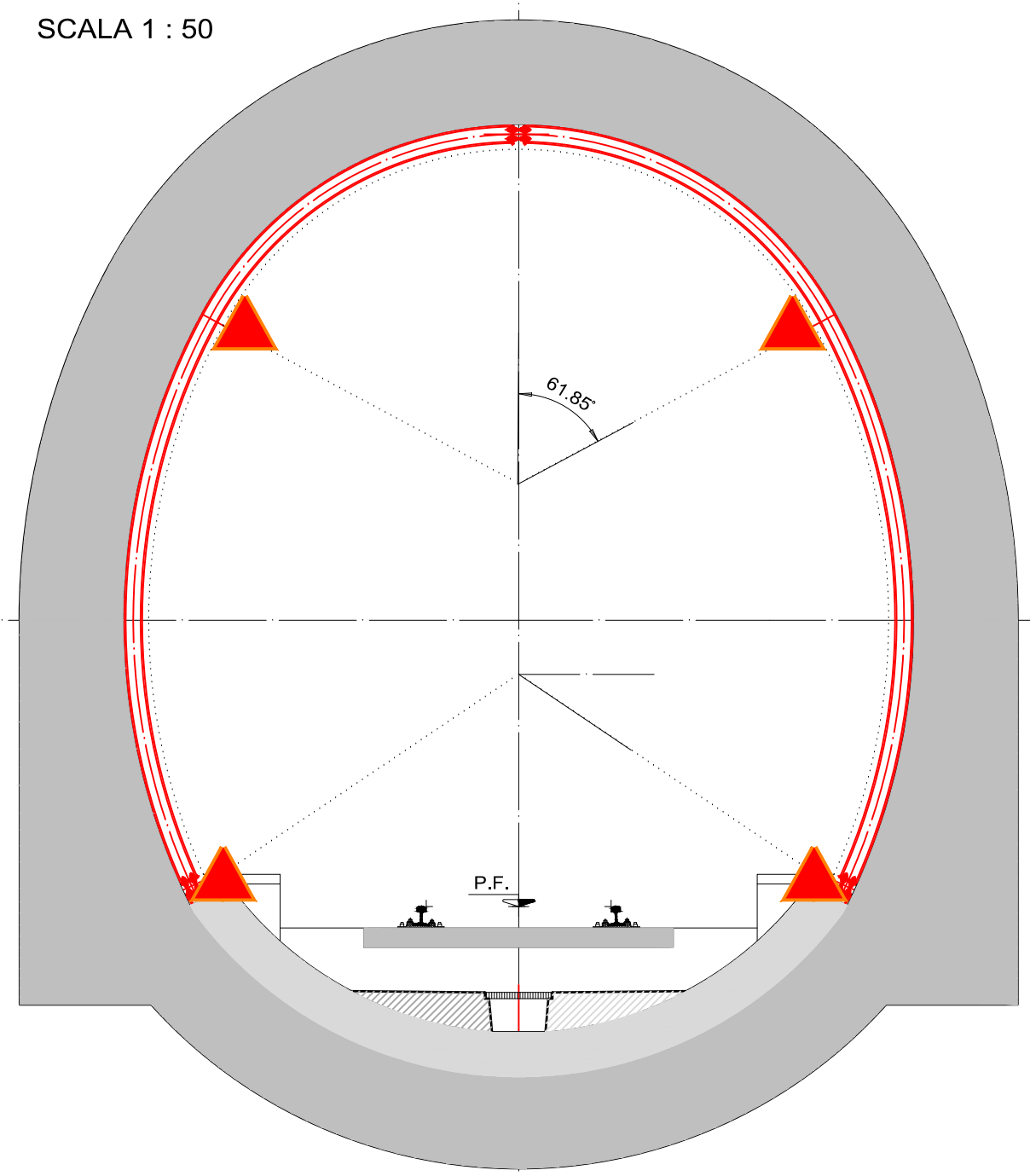
SEZIONE TIPO T1
