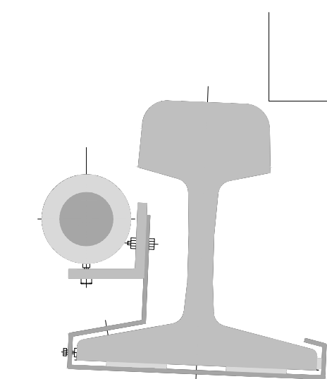
PARTICOLARE MICROPRISMI MONITORAGGIO PER BINARIO
