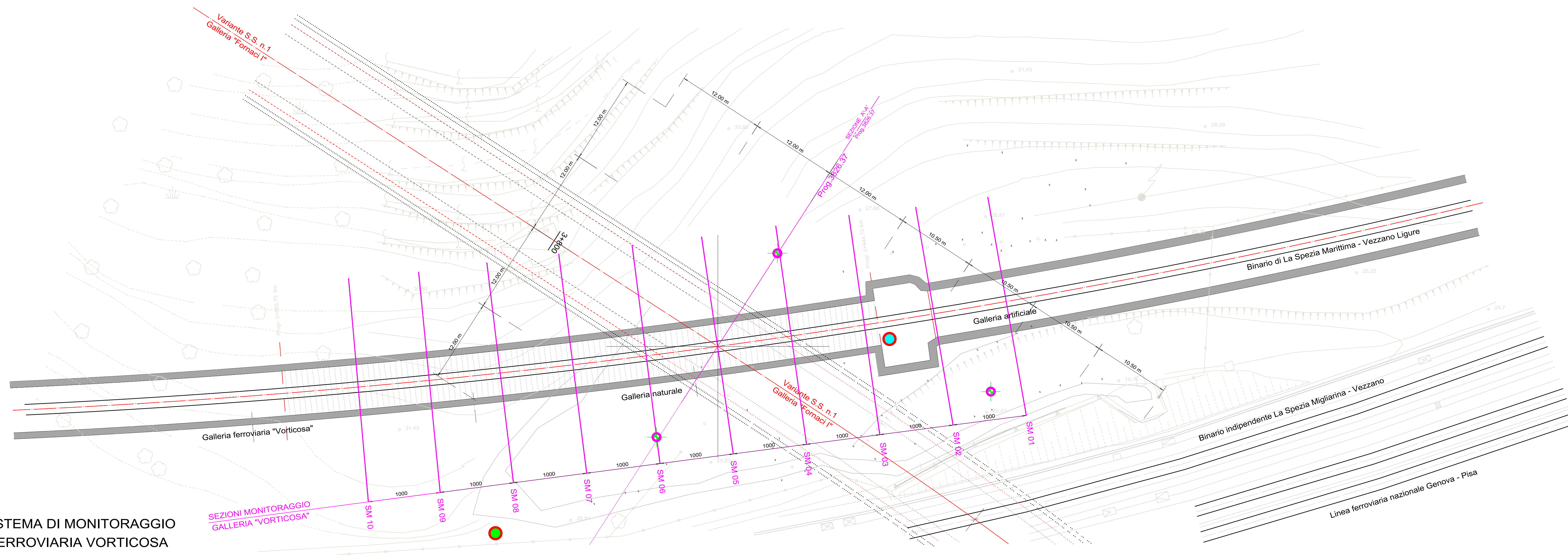
GALLERIA FERROVIARIA "VORTICOSA" COMPOSIZIONE SEZIONI DI MONITORAGGIO
