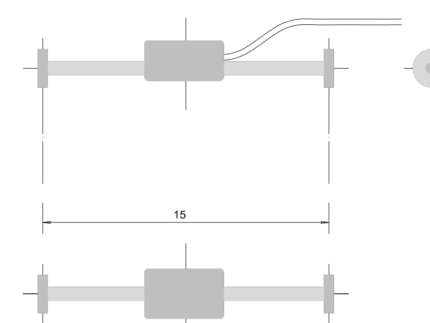
BARRETTA ESTENSIMETRICA TIPO A CORDA VIBRANTE (Interna a CLS rinforzo arco rovescio)
