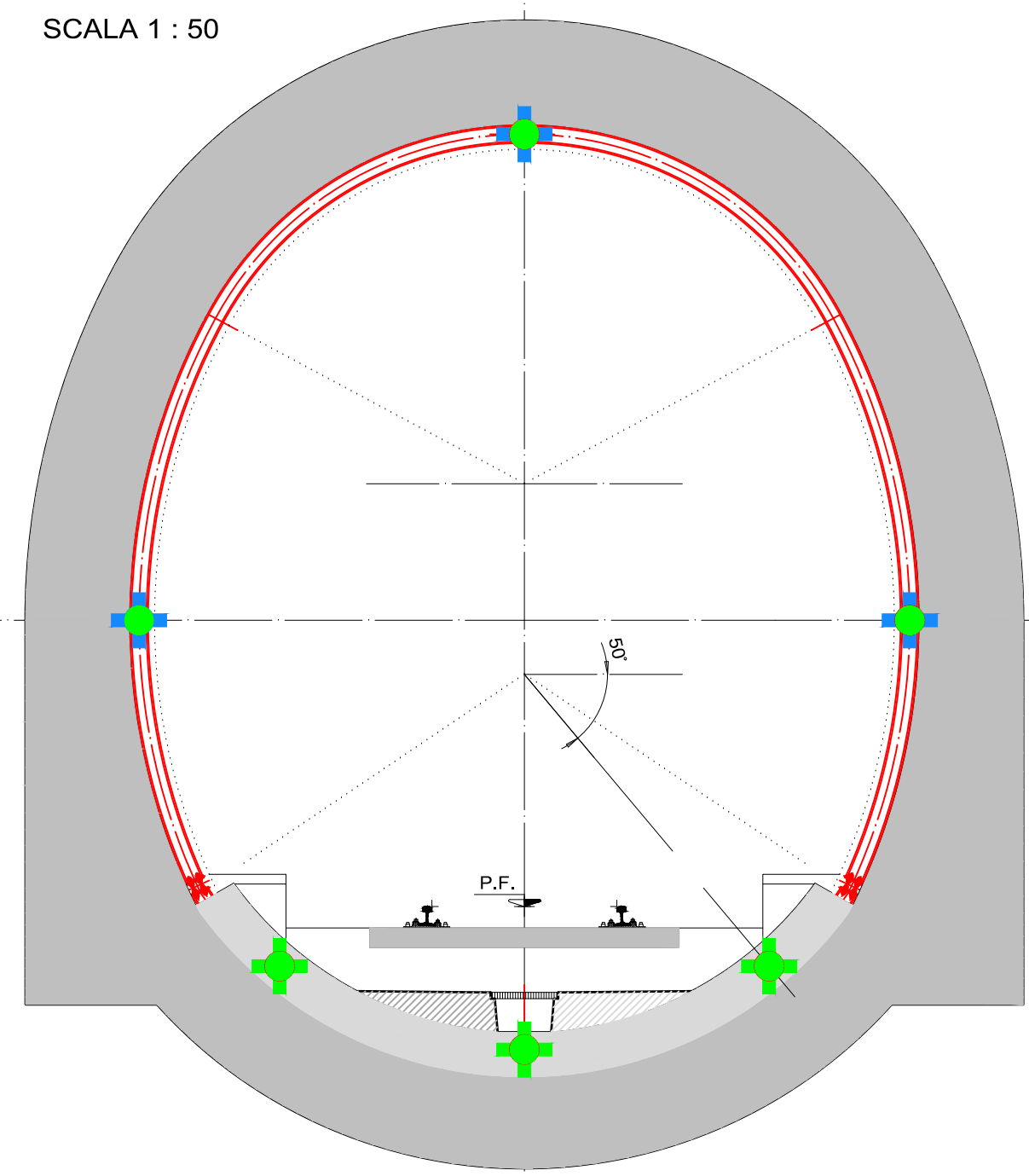
SEZIONE TIPO T2
