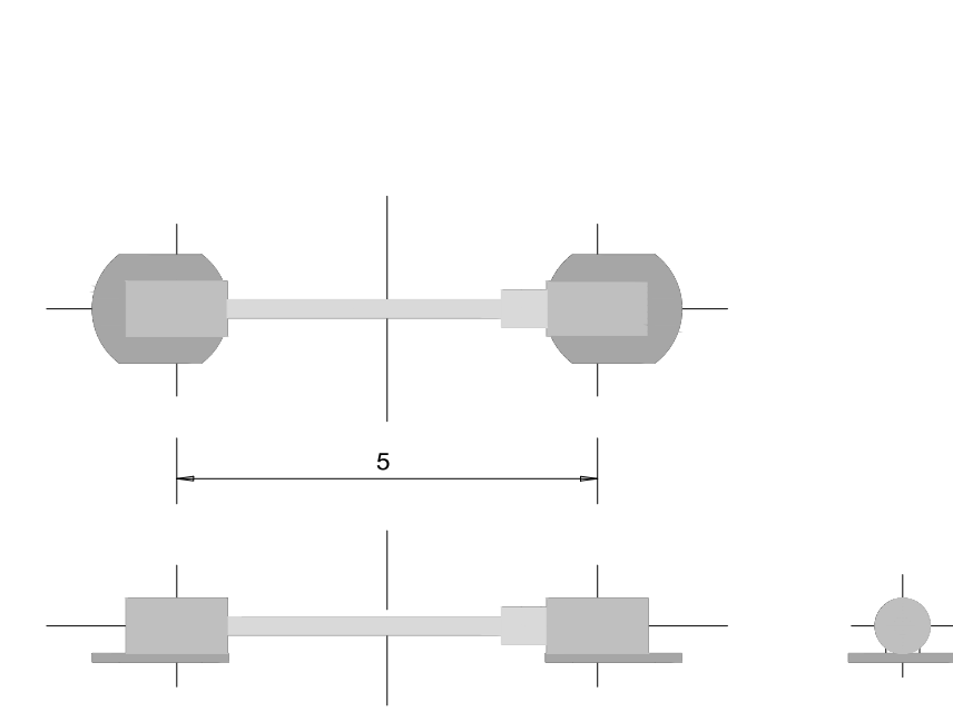
BARRETTA ESTENSIMETRICA TIPO A CORDA VIBRANTE (Per centine metalliche)
