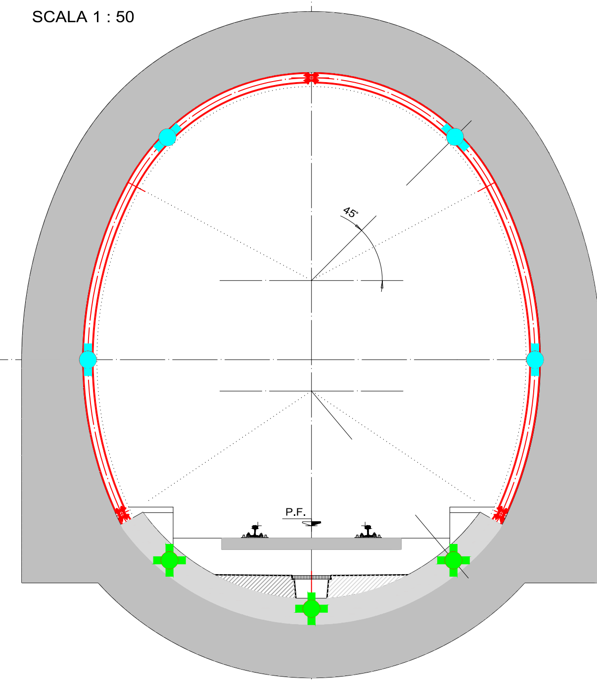
SEZIONE TIPO T4
