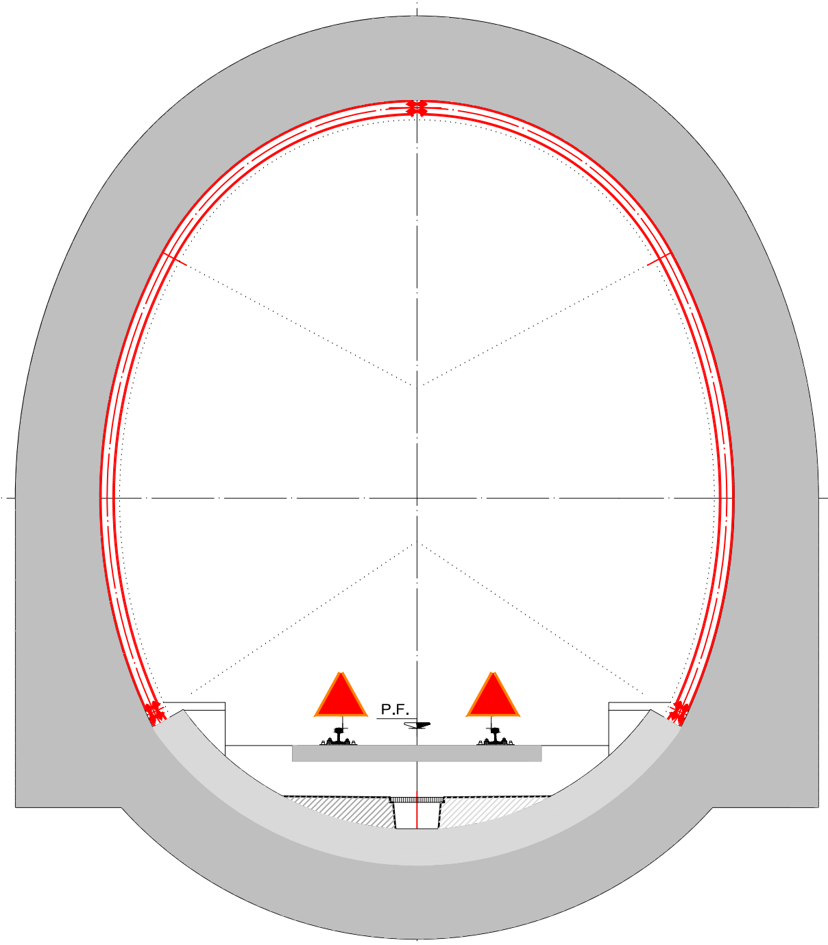
SEZIONE TIPO T5
