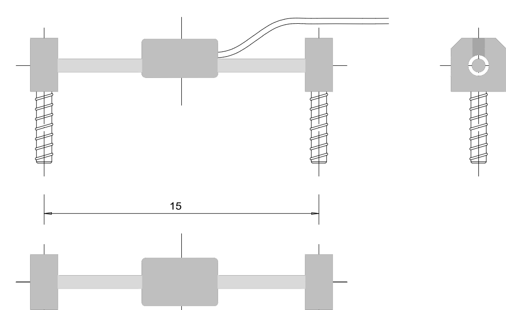
BARRETTA ESTENSIMETRICA TIPO A CORDA VIBRANTE (Per intradossso rivestimento)
