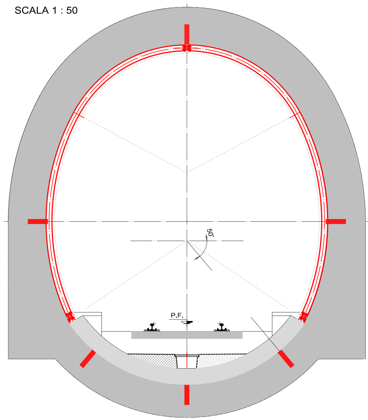
SEZIONE TIPO T3
