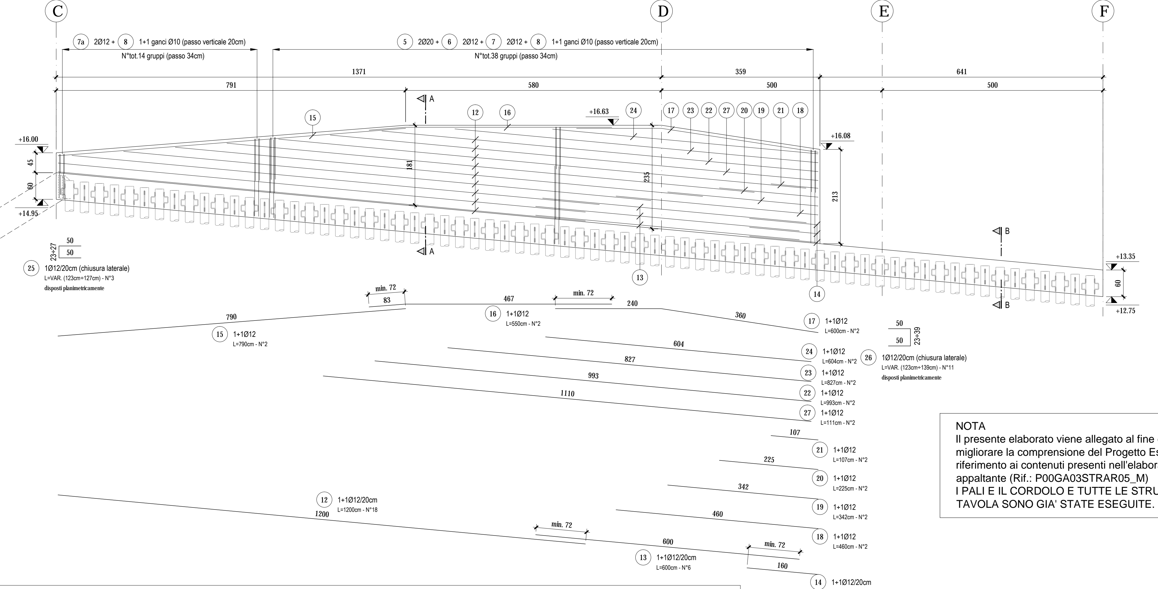
VISTA FRONTALE MURO IN ELEVAZIONE scala 1:50
