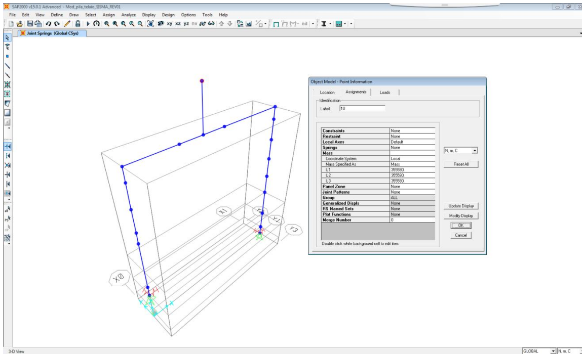
Figura 32 – modello di calcolo per sismica
