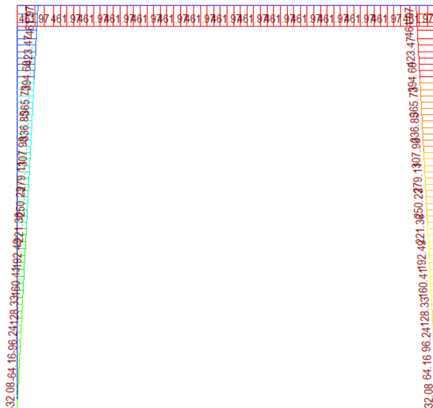
Figura 29 – Gradiente termico +10^{\circ}\text{C} – momento flettente
