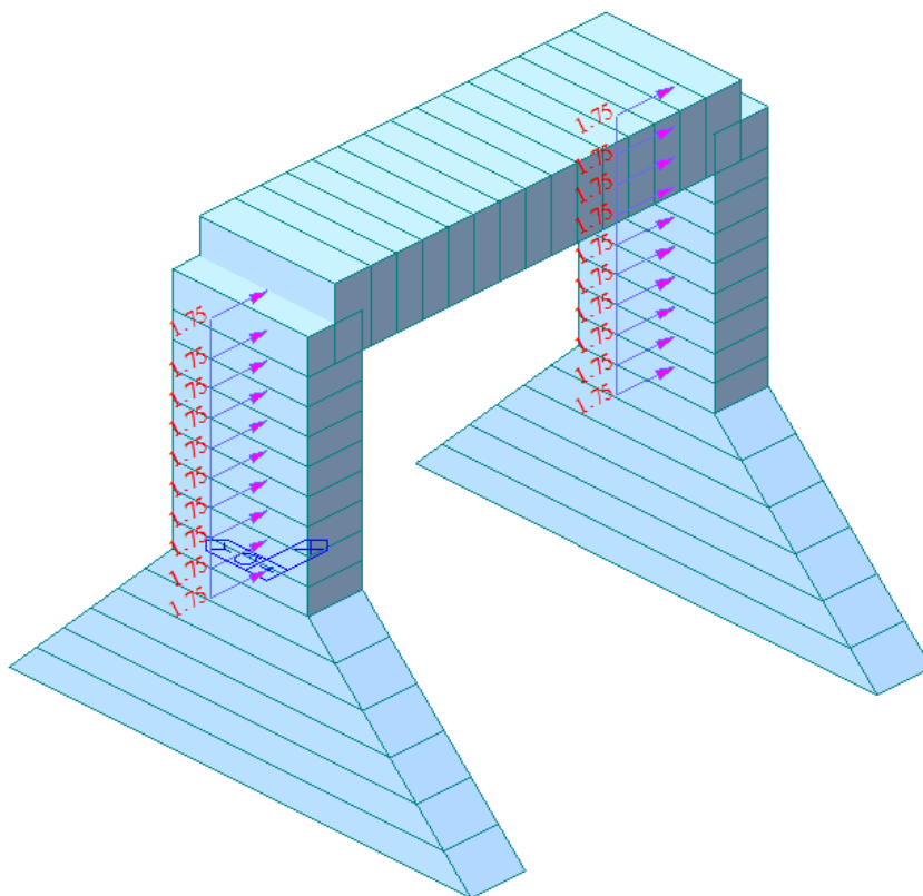
Figura 17 – Azione del vento in direzione trasversale
