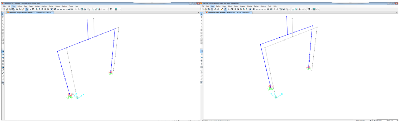
Figura 33 – 1° e 2° modo di vibrazione
