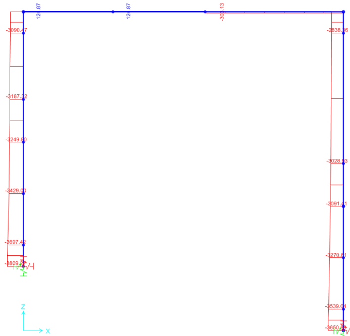
Figura 16 – diagramma sforzo normale – combinazione SLE
