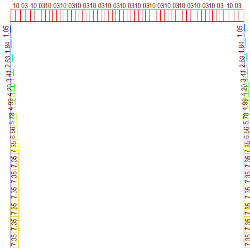
Figura 22 – Vento trasversale – forze di taglio
