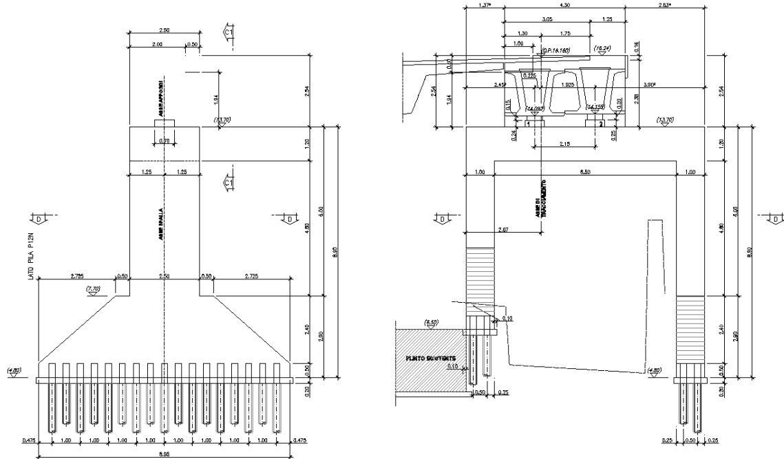
Figura 3 – Pila a telaio-carpenteria
