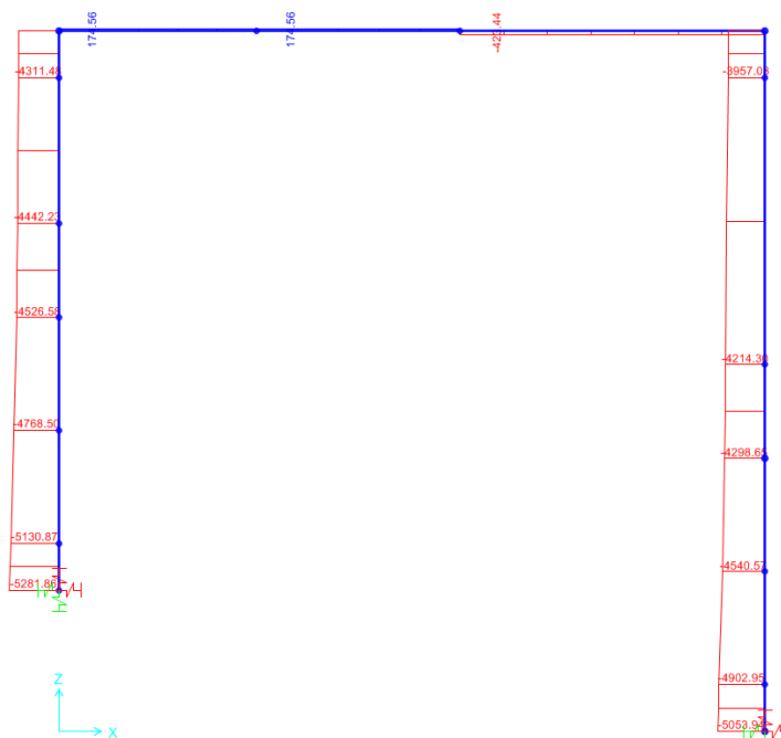
Figura 14 – diagramma sforzo normale – combinazione SLU
