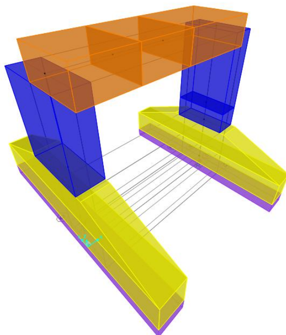
Figura 7 – modello di calcolo per la statica
