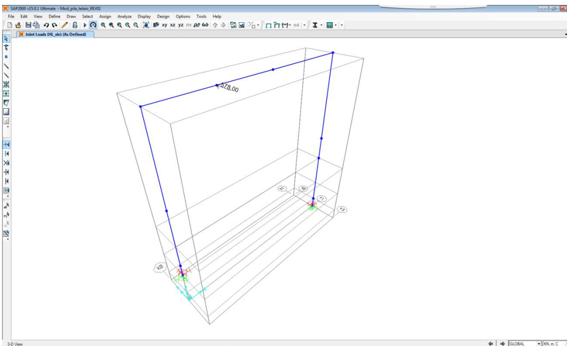
Figura 10 – applicazione carico longitudinale
