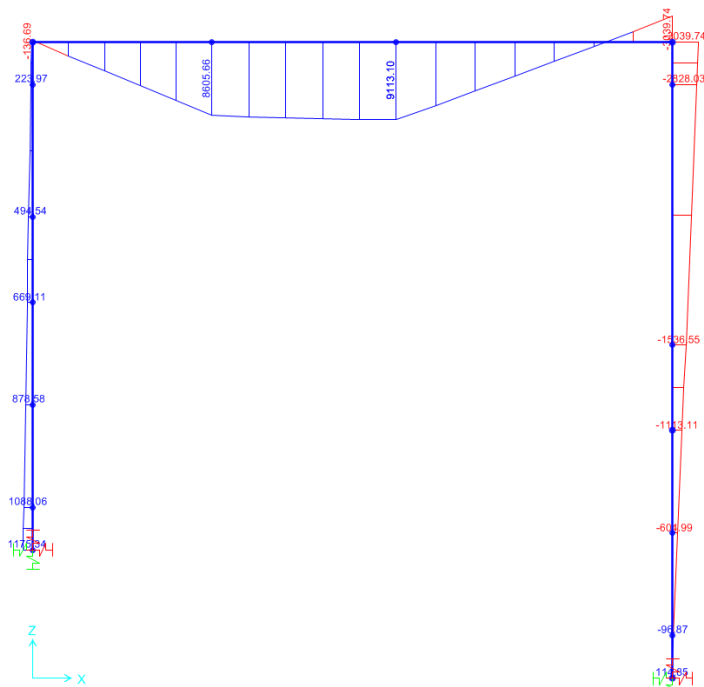
Figura 12 – diagramma del momento flettente – combinazione SLU
