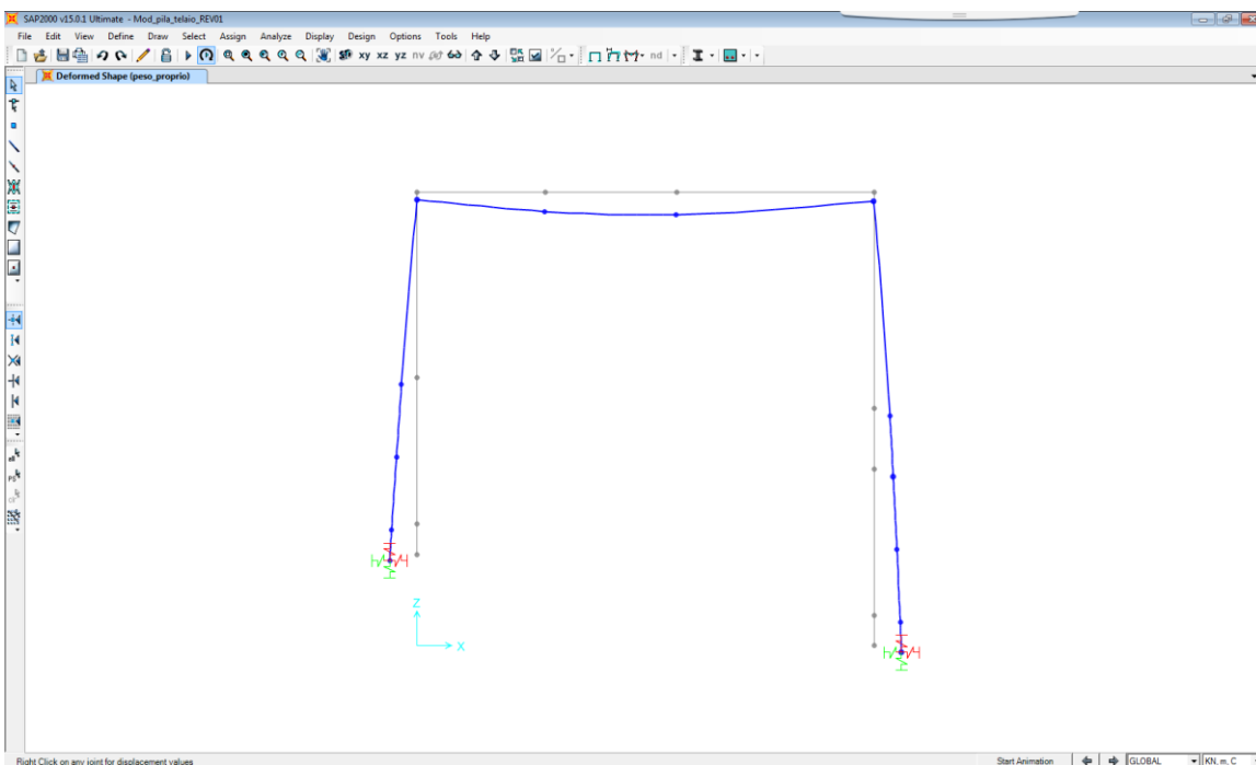
Figura 11 – deformata dovuta al peso proprio
