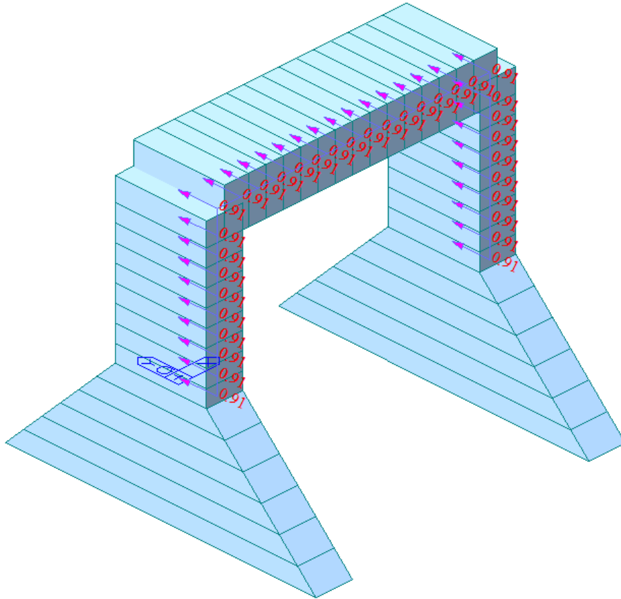
Figura 18 – Azione del vento in direzione longitudinale
