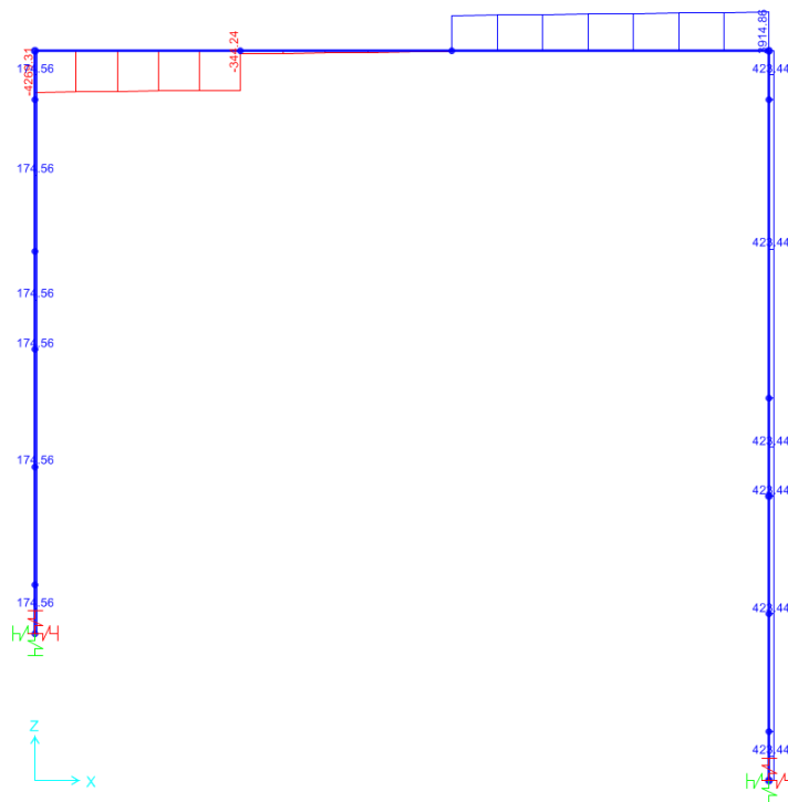
Figura 13 – diagramma del taglio – combinazione SLU
