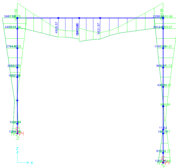
Figura 34 – diagramma momento flettente – combinazione SLC
