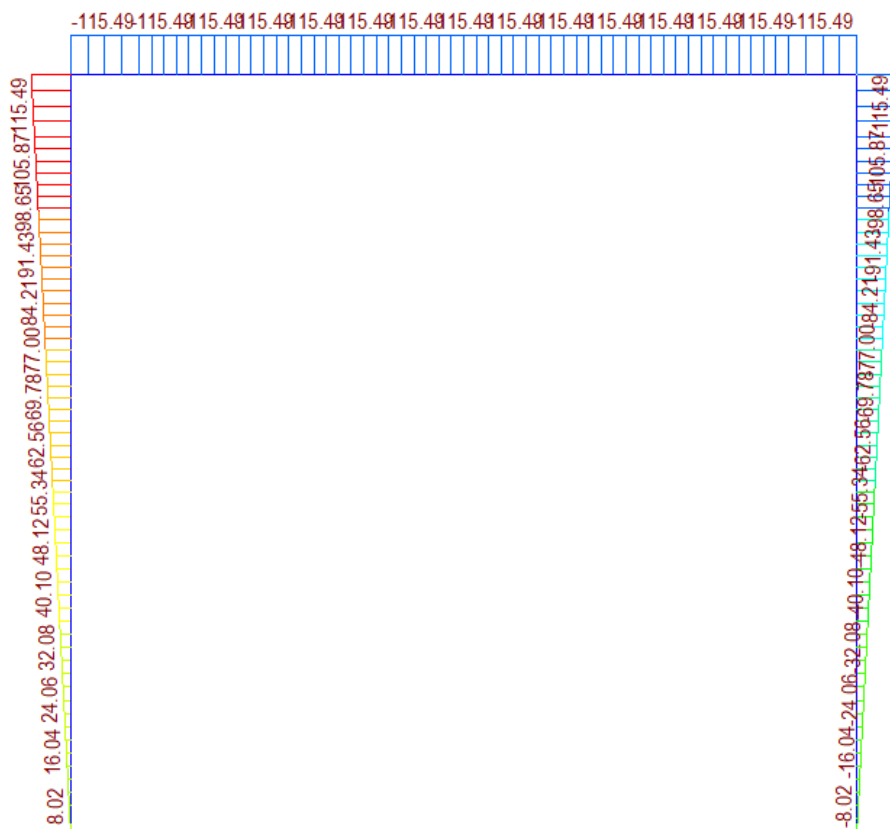
Figura 26 – Variazione termica uniforme +15°C – momento flettente
