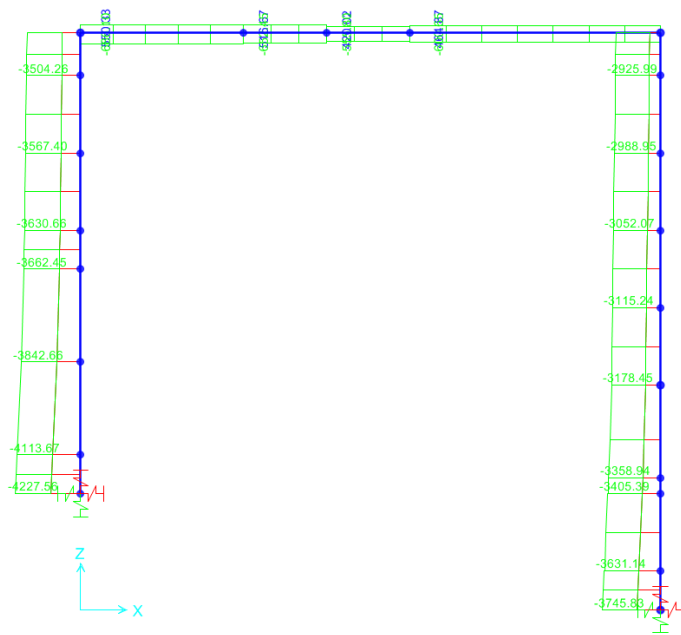
Figura 36 – diagramma sforzo normale – combinazione SLC
