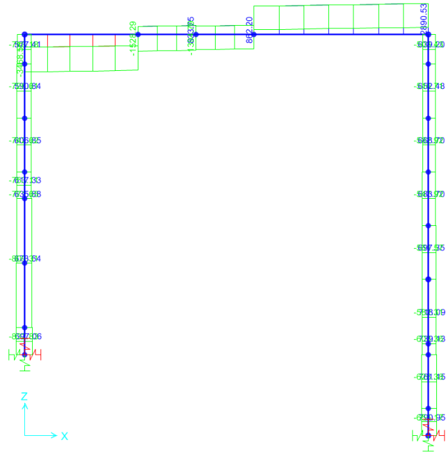
Figura 35 – diagramma taglio – combinazione SLC
