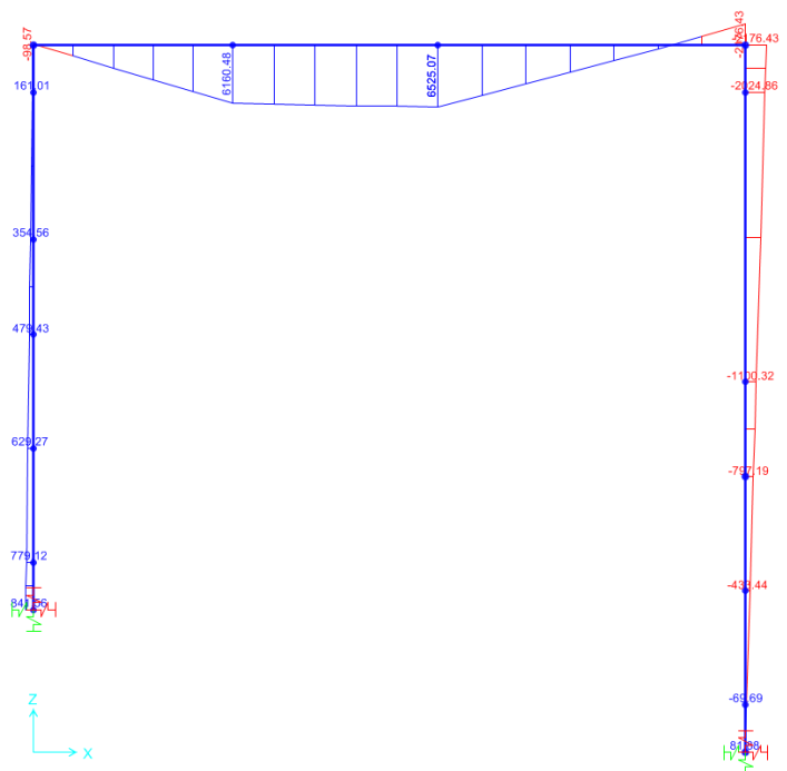
Figura 15 – diagramma del momento flettente – combinazione SLE
