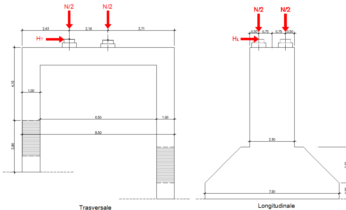
Figura 4 – schema di carico statico
