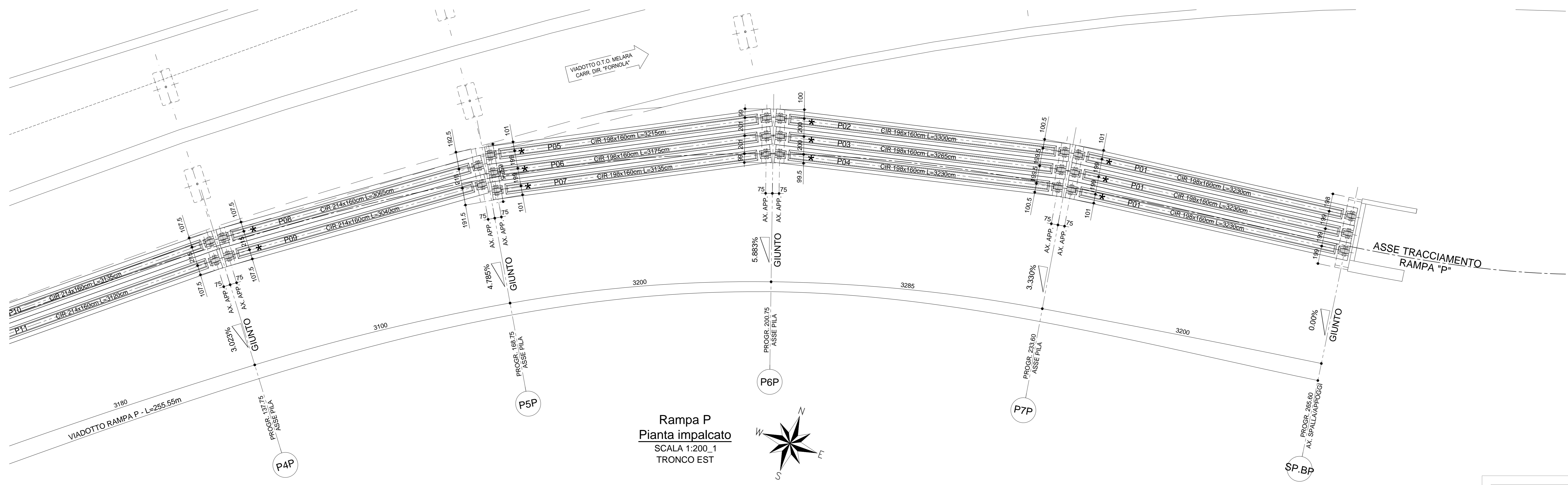
Rampa P Pianta impalcato SCALA 1:200_1 TRONCO OVEST
