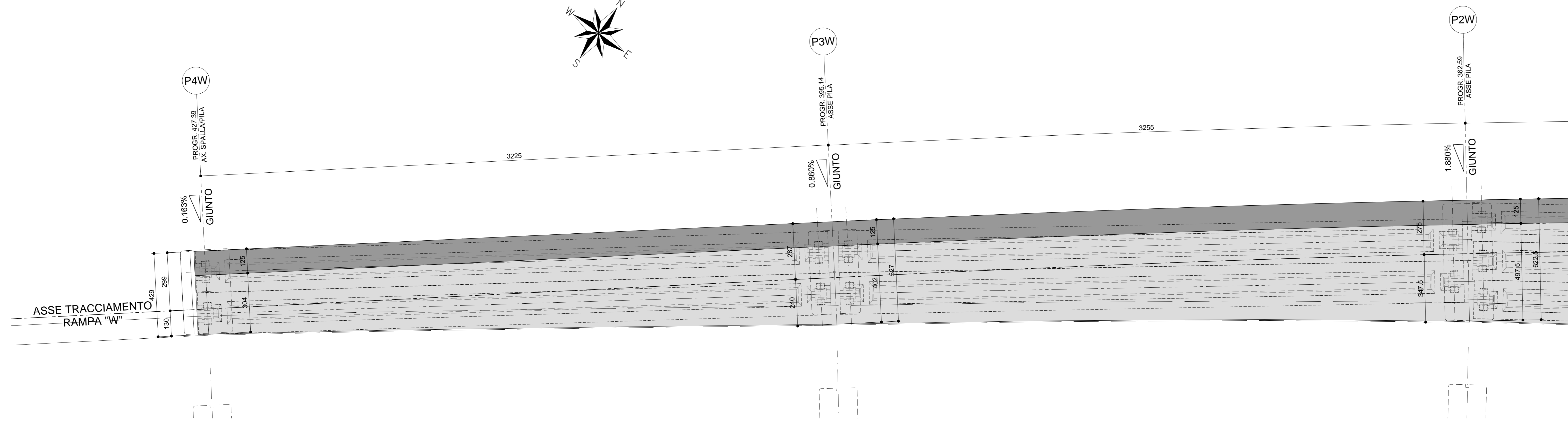
Rampa W Pianta soletta e traversi SCALA 1:100_2
