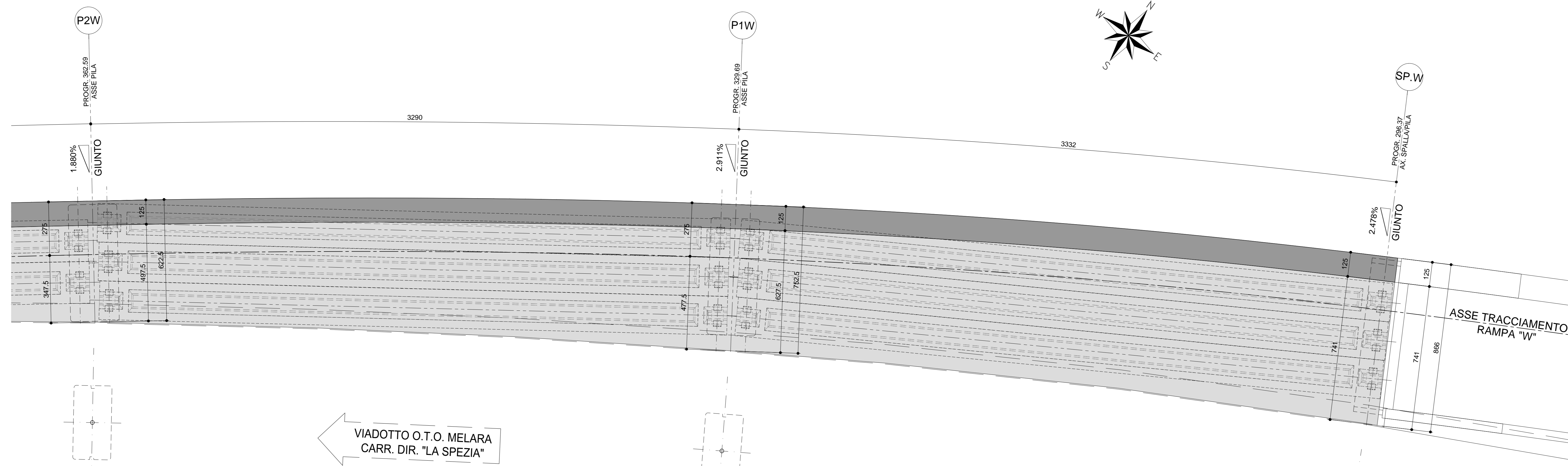
Rampa W Pianta soletta e traversi SCALA 1:100_2
