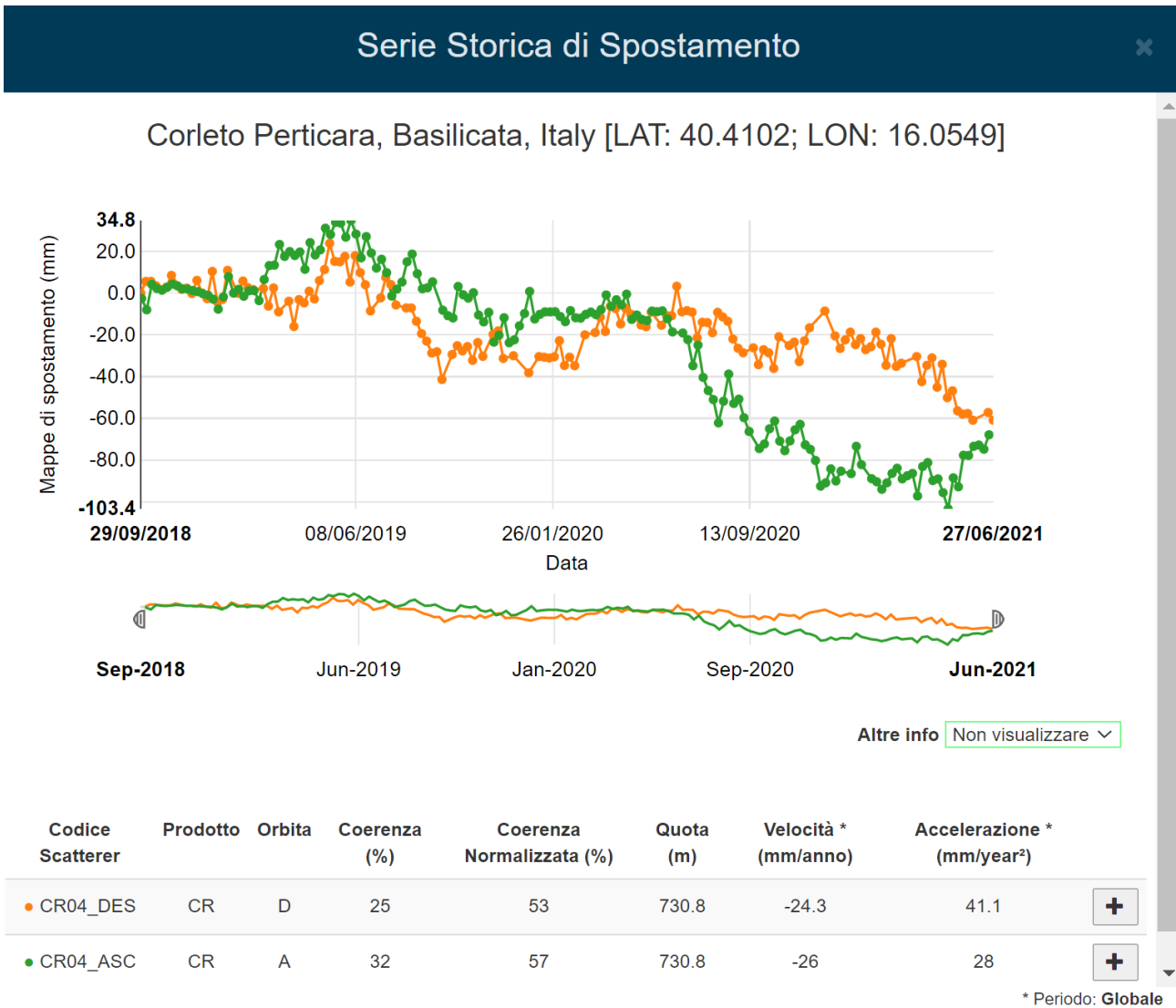
Figura 22: serie temporale di spostamento relativa al periodo settembre 2018 – Giugno 2021 misurata in corrispondenza del Corner Reflector CR04. La serie temporale di spostamento in verde è relativa all’orbita Ascending mentre quella arancione rappresenta la serie temporale relativa all’orbita Descending.
