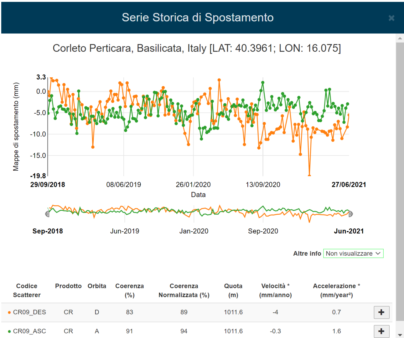
Figura 28: serie temporale di spostamento relativa al periodo settembre 2018 – Giugno 2021 misurata in corrispondenza del Corner Reflector CR09. La serie temporale di spostamento in verde è relativa all’orbita Ascending mentre quella arancione rappresenta la serie temporale relativa all’orbita Descending.
