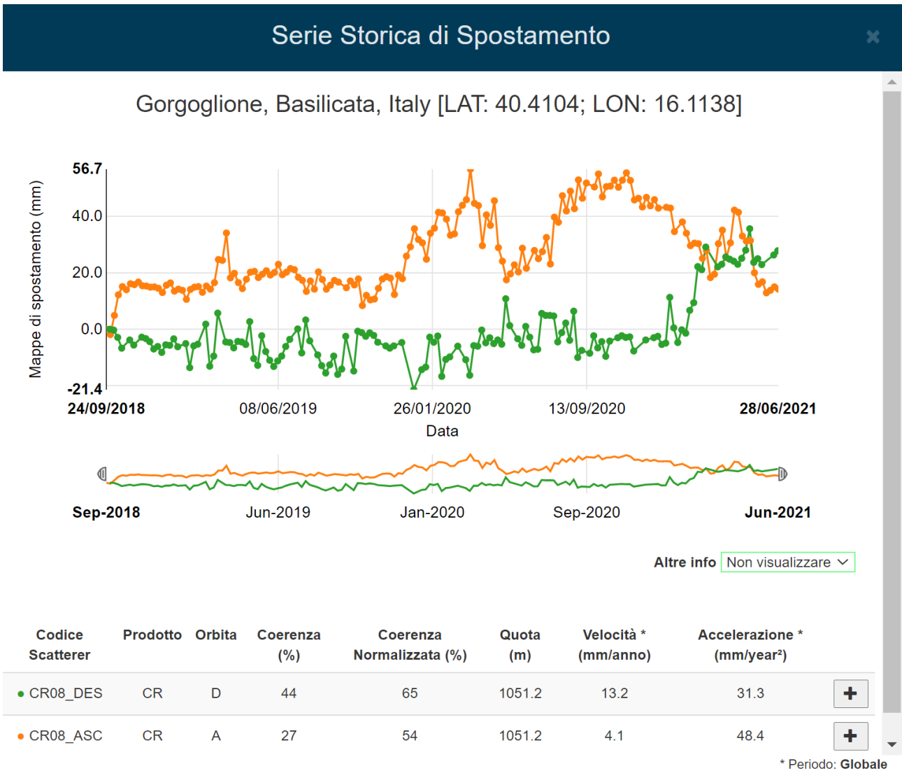
Figura 16: serie temporale di spostamento relativa al periodo settembre 2018 – Giugno 2021 misurata in corrispondenza del Corner Reflector CR08. La serie temporale di spostamento in arancione è relativa all’orbita Ascending mentre quella verde rappresenta la serie temporale relativa all’orbita Descending.
