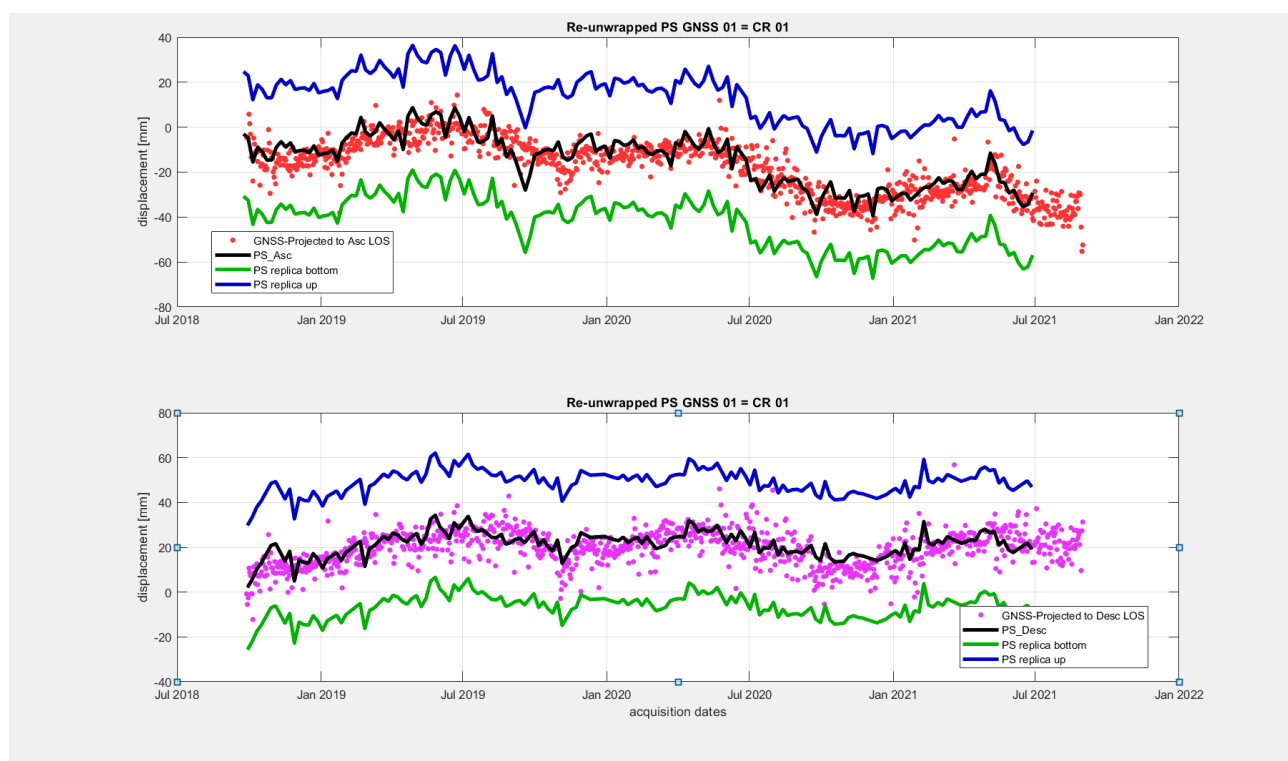
Figura 39: la figura in alto riporta la proiezione delle misure GNSS in corrispondenza del Corner Reflector CR01 (punti rossi) sulla viste SAR ascending mentre la figura in basso riporta la proiezione delle misure GNSS sulla vista SAR descending (punti viola) e raffronto con le misure SAR rappresentate dalla linea nera (le linee blu e verdi rappresentano le due repliche delle misure SAR di una quantità pari a \pm \lambda/2 ). Si nota un ottimo accordo a livello qualitativo.
