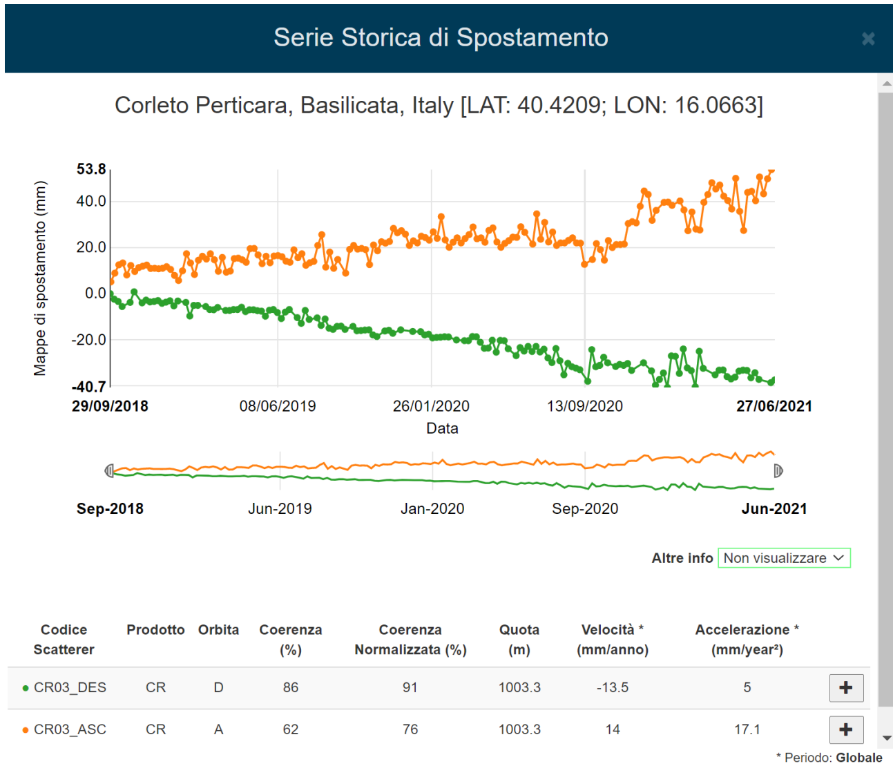
Figura 25: serie temporale di spostamento relativa al periodo settembre 2018 – giugno 2021 misurata in corrispondenza del Corner Reflector CR03. La serie temporale di spostamento in verde è relativa all'orbita Descending mentre quella arancione rappresenta la serie temporale relativa all'orbita Ascending.
