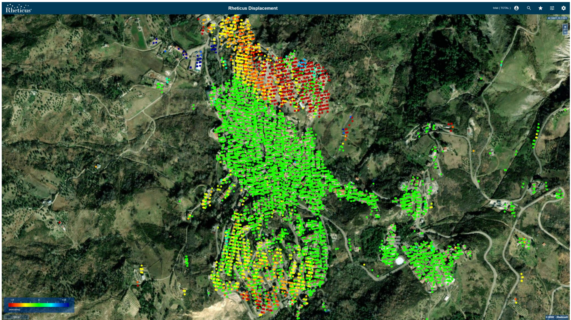
Figura 9: La mappa di velocità media (mm/anno) PS/DS sul centro abitato di Stigliano calcolata sul periodo esteso a Giugno 2021 non mostra variazioni significative rispetto al rapporto precedente [RD10].
