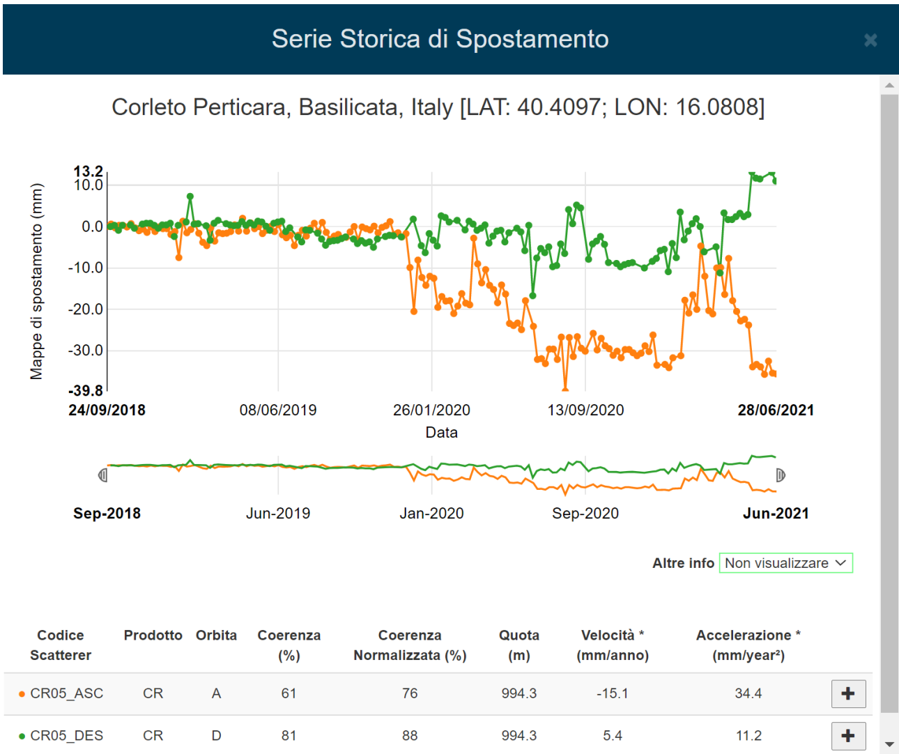
Figura 13: serie temporale di spostamento relativa al periodo settembre 2018 – Giugno 2021 misurata in corrispondenza del Corner Reflector CR05. La serie temporale di spostamento in arancione è relativa all’orbita Ascending mentre quella verde rappresenta la serie temporale relativa all’orbita Descending. Dall’analisi delle serie temporali si evince uno spostamento misurato in orbita descending di circa 2 cm nel semestre Dicembre 2020 - Giugno 2021.
