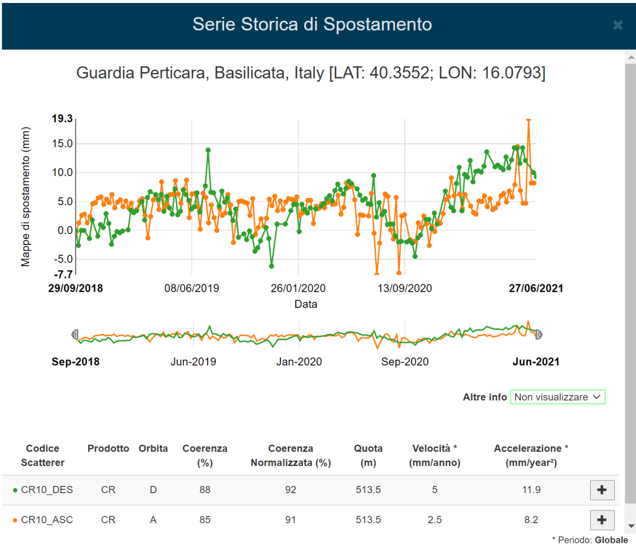
Figura 31: serie temporale di spostamento relativa al periodo settembre 2018 – Giugno 2021 misurata in corrispondenza del Corner Reflector CR10. La serie temporale di spostamento in verde è relativa all’orbita Descending mentre quella arancione rappresenta la serie temporale relativa all’orbita Ascending.
