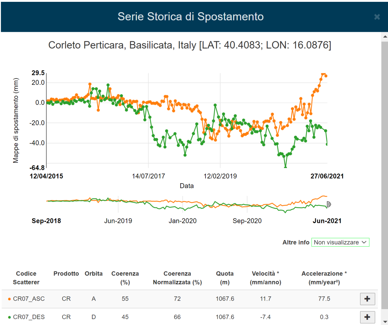
Figura 34: serie temporale di spostamento relativa al periodo settembre 2018 – Giugno 2021 misurata in corrispondenza del Corner Reflector CR07. La serie temporale di spostamento in verde è relativa all'orbita Descending mentre quella arancione rappresenta la serie temporale relativa all'orbita Ascending. Il ripristino atteso della risposta radiometrica sia in orbita Ascending che Descending, diminuita a partire dal 2020, grazie alle attività di manutenzione effettuate su tutti i CR, verrà verificato nel prossimo rapporto.
