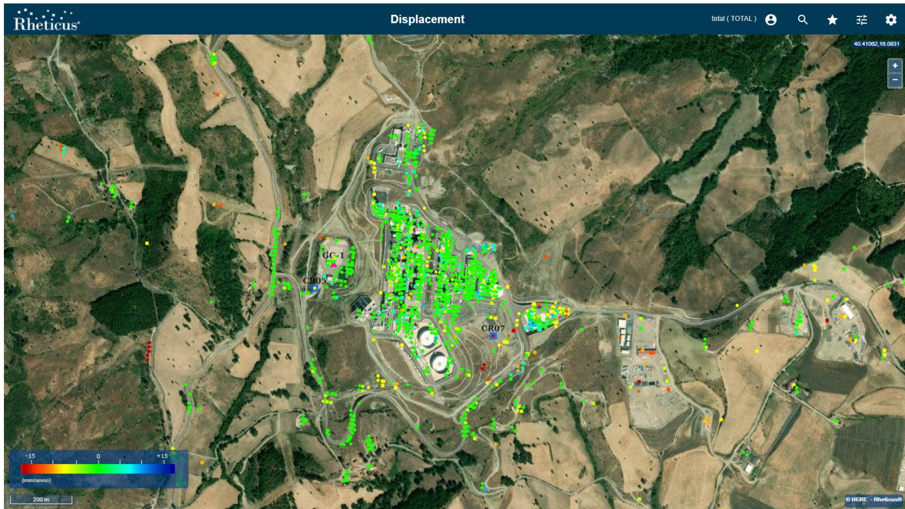
Figura 33: Oil Center caratterizzato da una buona copertura di PS e dai quali nel periodo esteso a Giugno 2021, non si evincono variazioni significative di velocità media rispetto al precedente rapporto [RD10].
