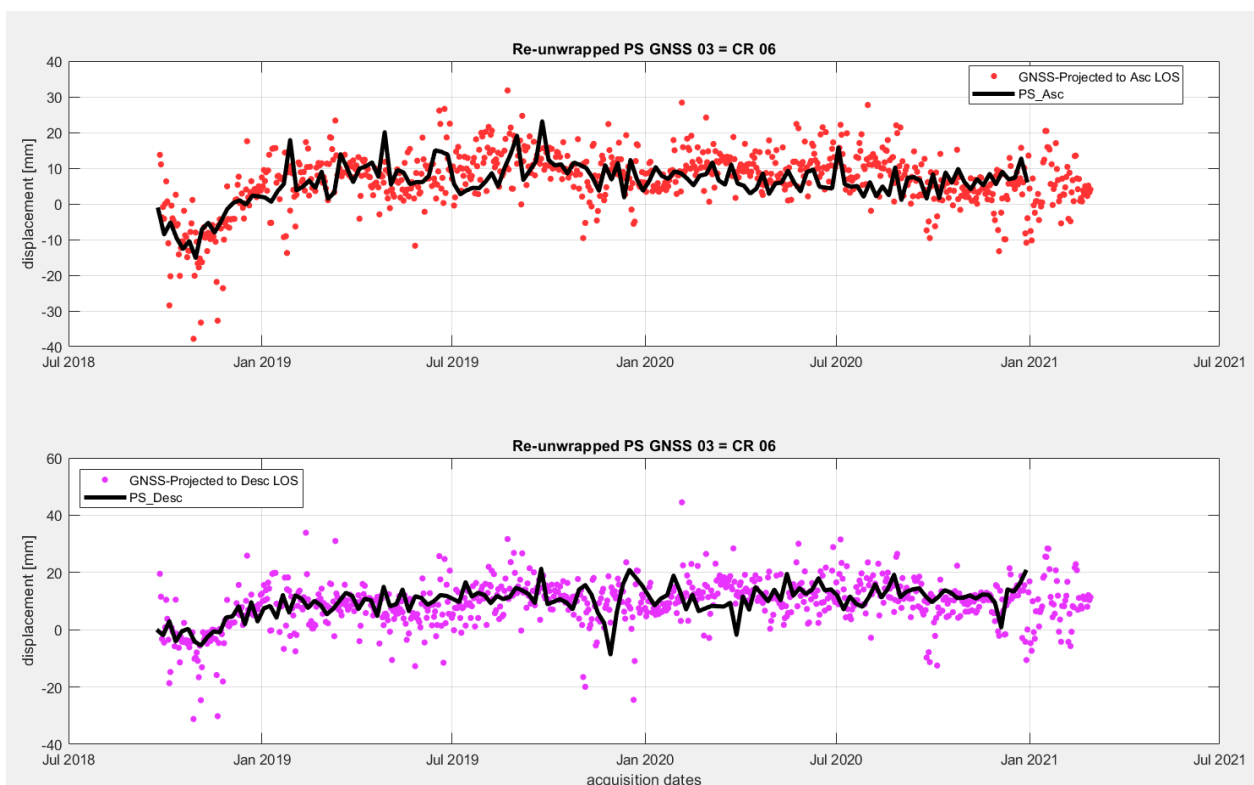
Figura 41: la figura in alto riporta la proiezione delle misure GNSS in corrispondenza del Corner Reflector CR06 (punti rossi) sulla viste SAR ascending mentre la figura in basso riporta la proiezione delle misure GNSS sulla vista SAR descending (punti viola) e raffronto con le misure SAR (linea nera). Si nota un ottimo accordo a livello qualitativo.
