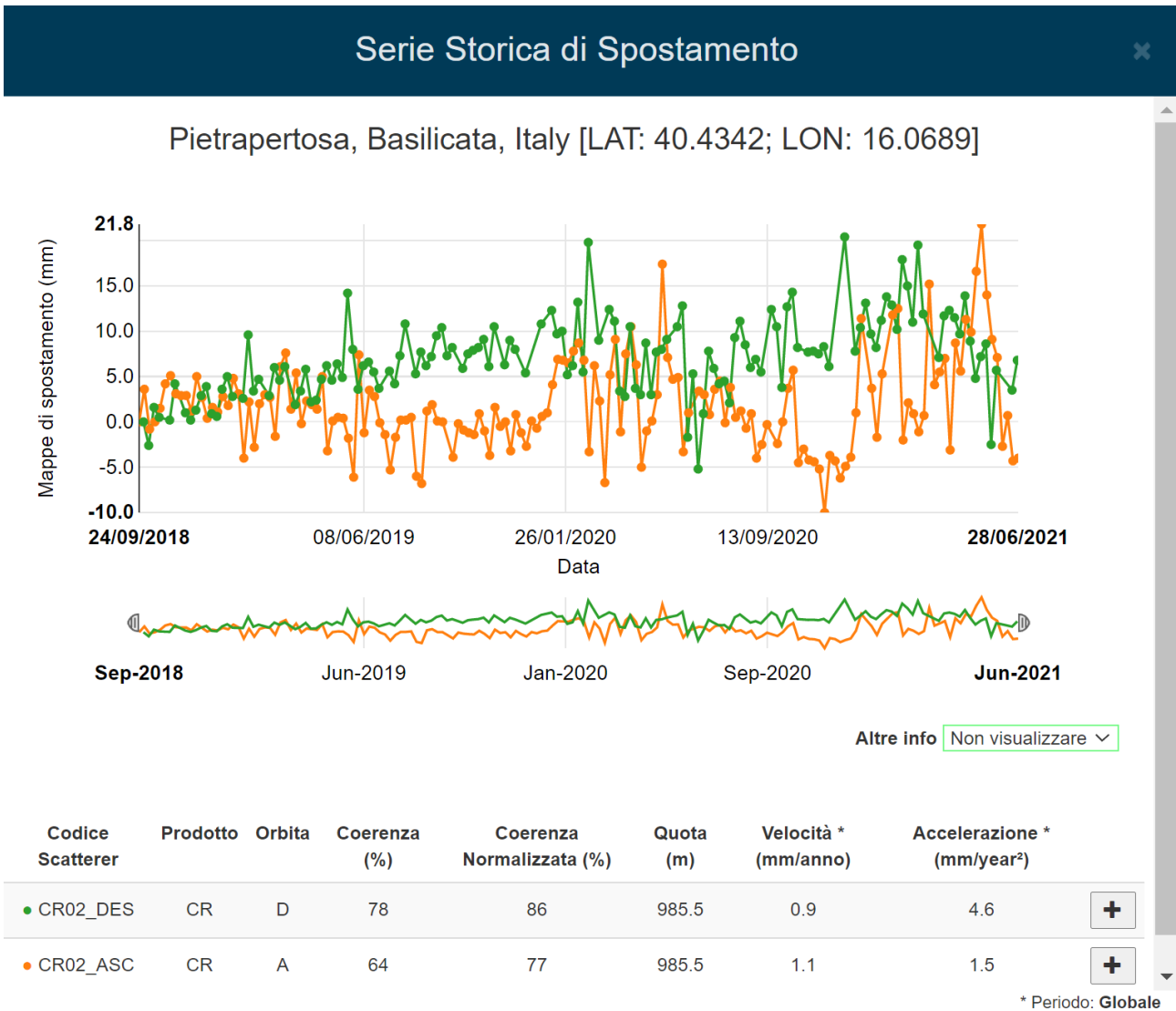
Figura 19: serie temporale di spostamento relativa al periodo settembre 2018 – Giugno 2021 misurata in corrispondenza del Corner Reflector CR02. La serie temporale di spostamento in verde è relativa all’orbita Descending mentre quella arancione rappresenta la serie temporale relativa all’orbita Ascending. Dall’analisi delle serie temporali non si evincono spostamenti significativi, in linea con quanto misurato nel precedente rapporto [RD10].
