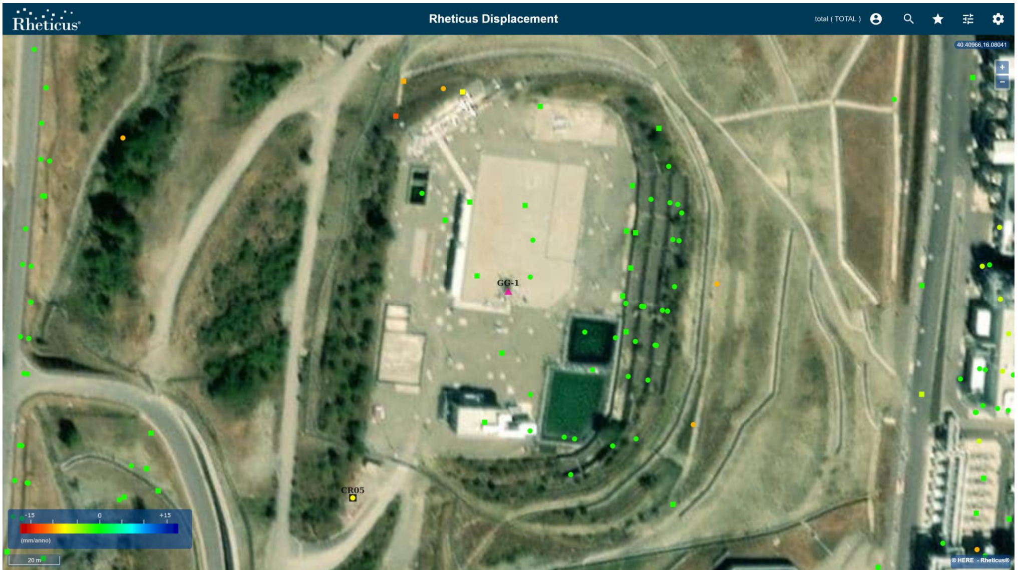
Figura 12: Pozzo GG-1 (indicato dal triangolo fucsia) caratterizzato da una buona copertura di PS e dai quali, nel periodo esteso a Giugno 2021, non si evincono variazioni significative di velocità media rispetto al precedente rapporto [RD10].
