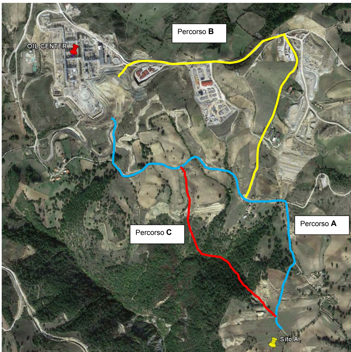
Fig. 5.a Individuazione dei percorsi della flowline proposti A, B, e C su ortofoto.
