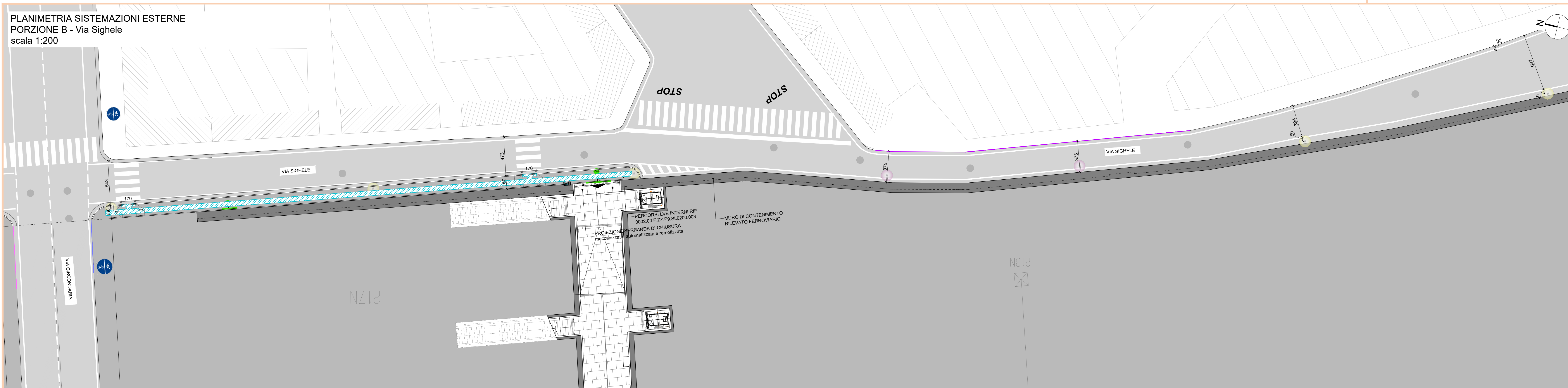
PLANIMETRIA SISTEMAZIONI ESTERNE PORZIONE C - Via Sighele scala 1:200
