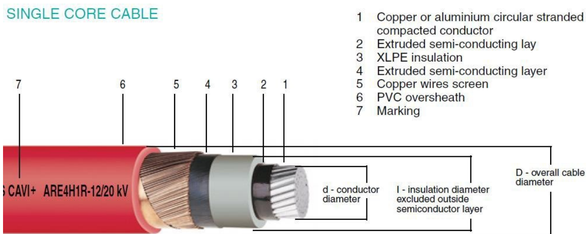
Fig. 1: caratteristiche cavi unipolari
