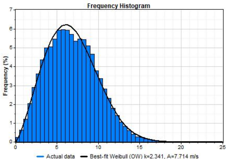
Figura 15: Distribuzione delle frequenze di Weibull
