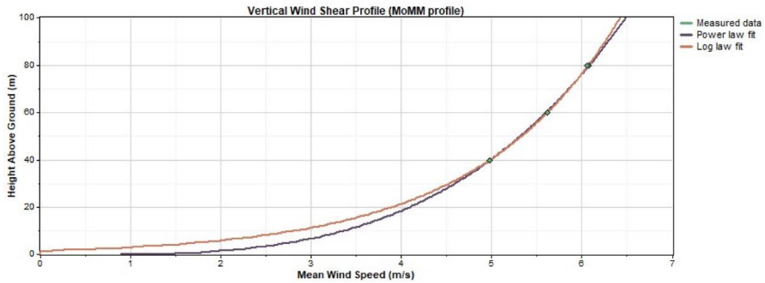
Figura 8: Stazione Anemometrica - Profilo verticale diurno del vento
