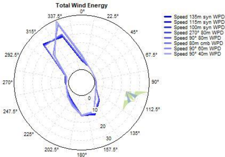
Figura 16: Energia totale del vento
