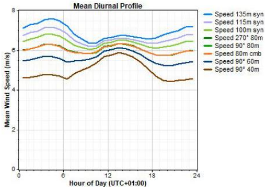
Figura 13: Profilo medio diurno del vento elaborato ad altezza mozzo
