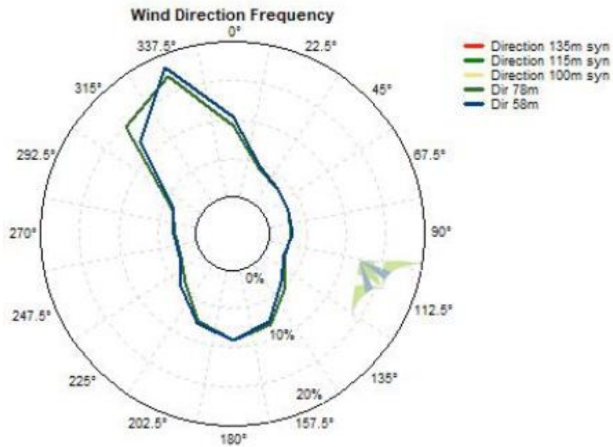
Figura 12: Direzione prevalente del vento elaborato ad altezza mozzo
