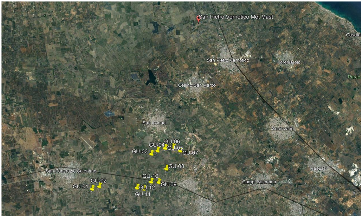
Figura 4: Posizione della Stazione Anemometrica rispetto all'impianto
