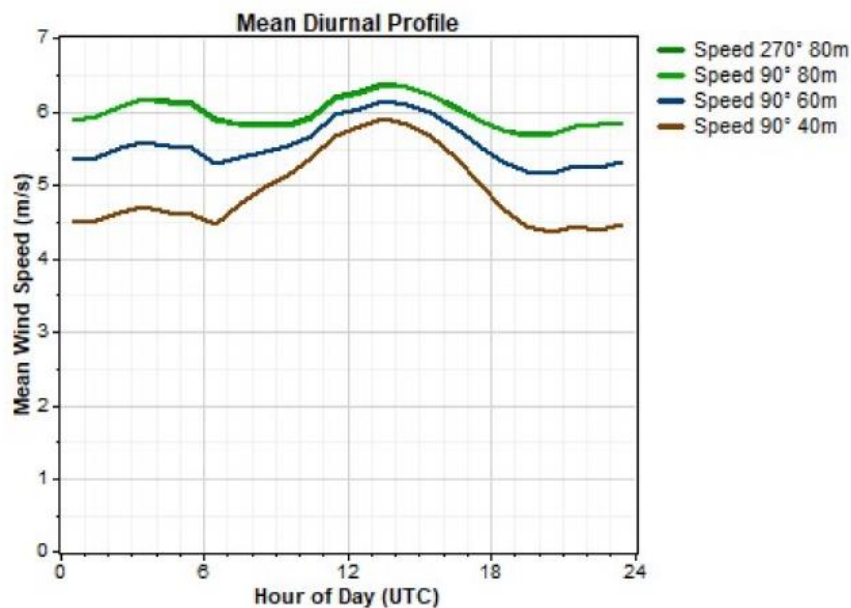
Figura 7: Stazione Anemometrica - Profilo medio diurno del vento
