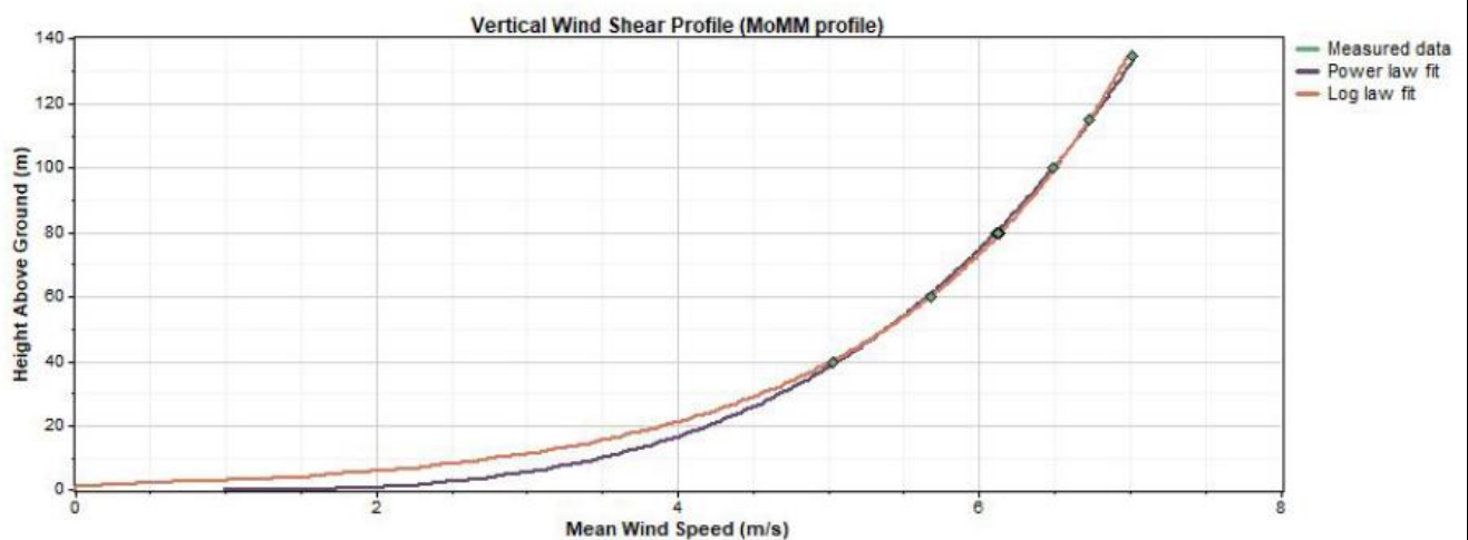
Figura 14: Profilo verticale diurno del vento elaborato ad altezza mozzo
