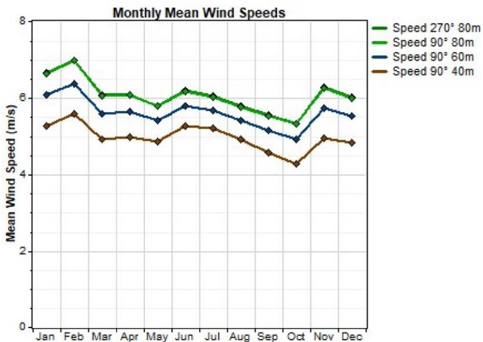
Figura 5: Stazione Anemometrica - Profilo medio mensile di velocità del vento a diverse altezze
