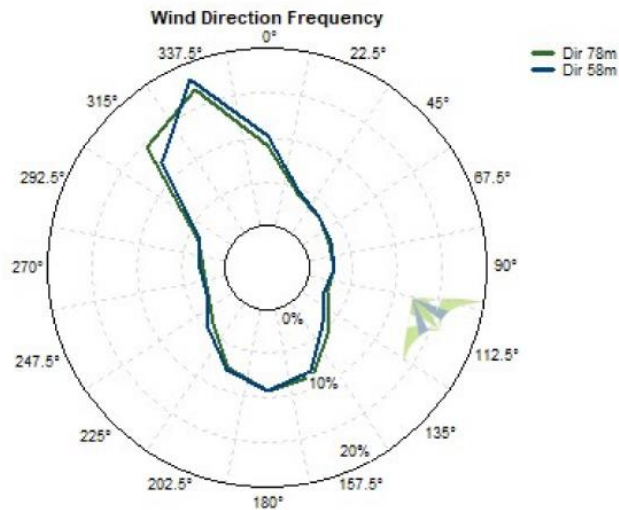
Figura 6: Stazione Anemometrica - Direzione prevalente del vento a diverse altezze
