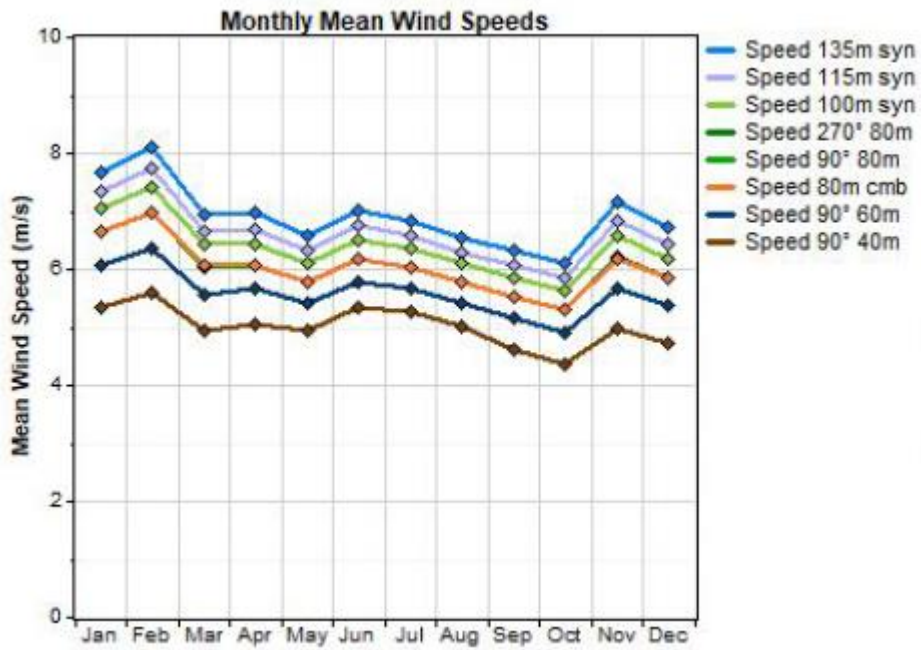
Figura 11: Profilo medio mensile di velocità del vento elaborato ad altezza mozzo
